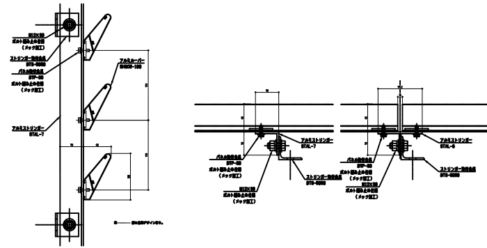
アルミルーバー SHGCW-100 アルミストリンガー STAL-7 STAL-8
