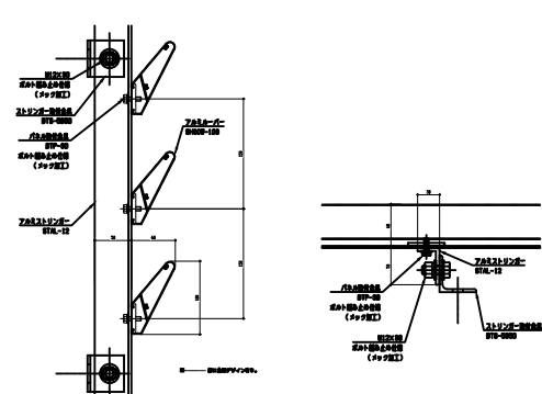
アルミルーバー SHGCW-100 アルミストリンガー STAL-12
