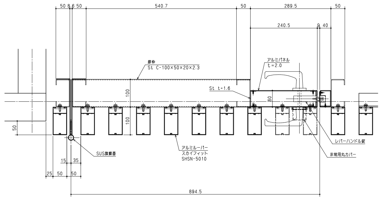
平面詳細図
