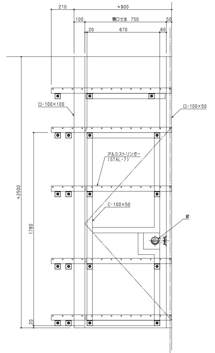
胴縁立面図
