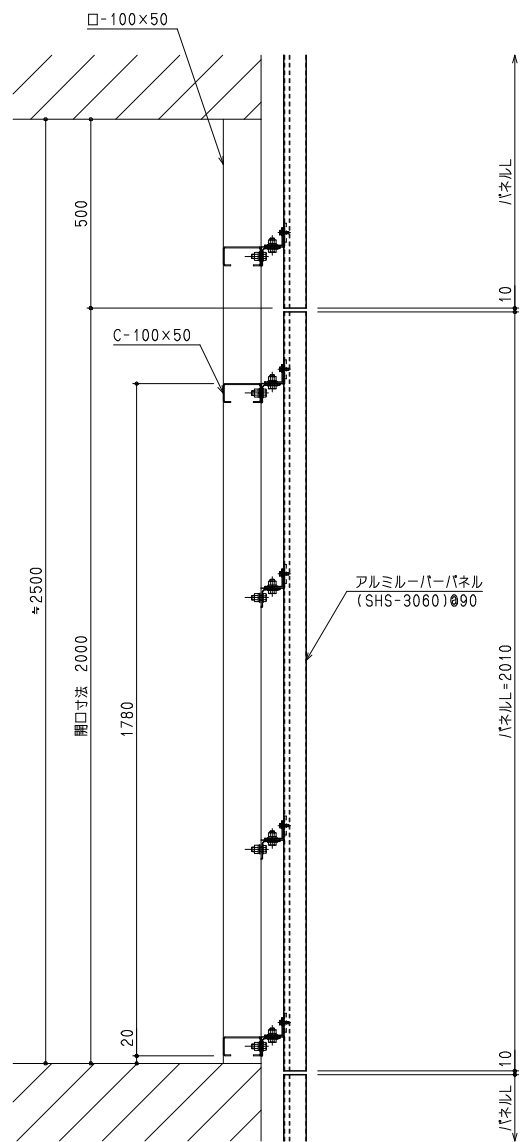
断面図
