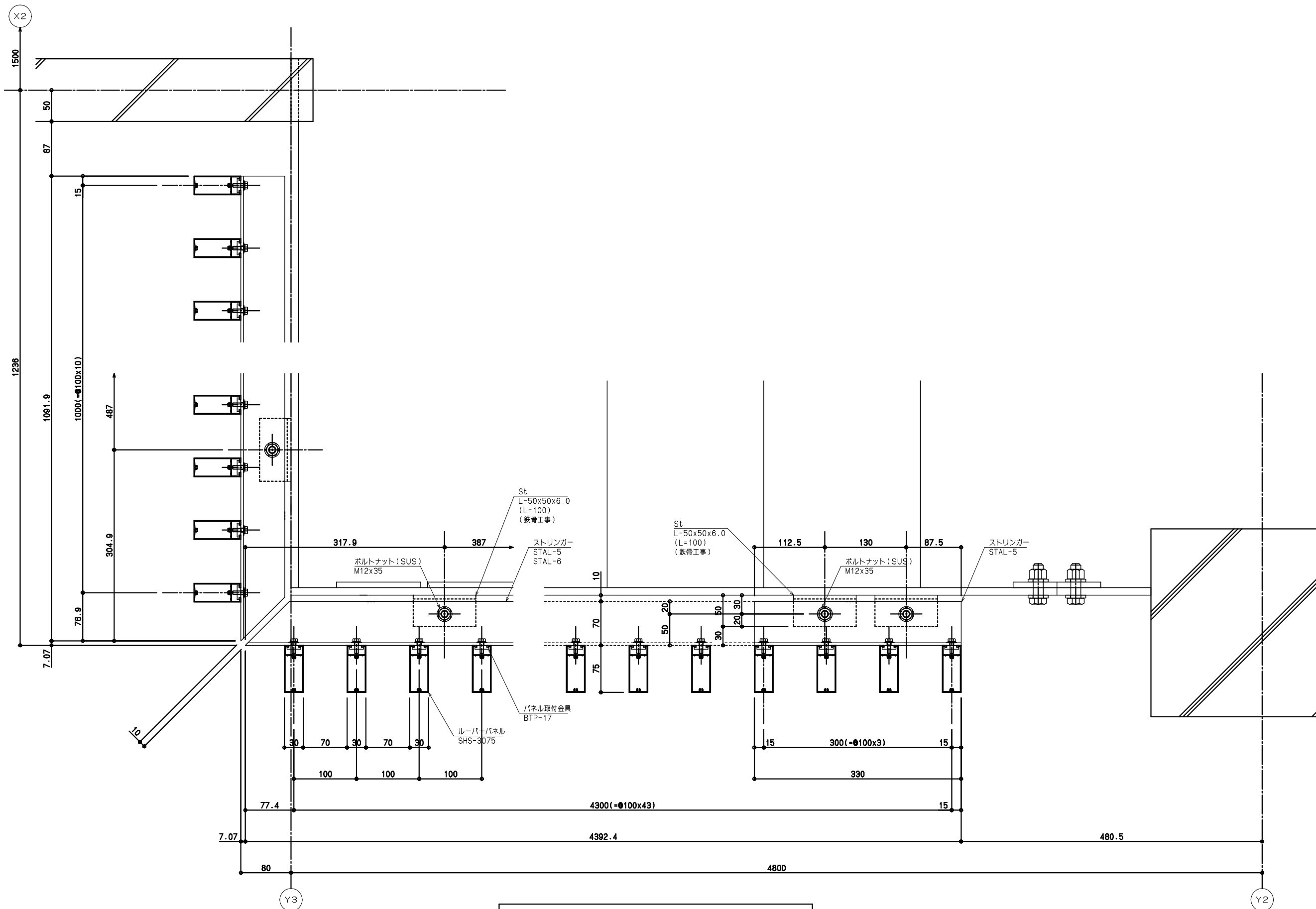
C-C 断面詳細図
