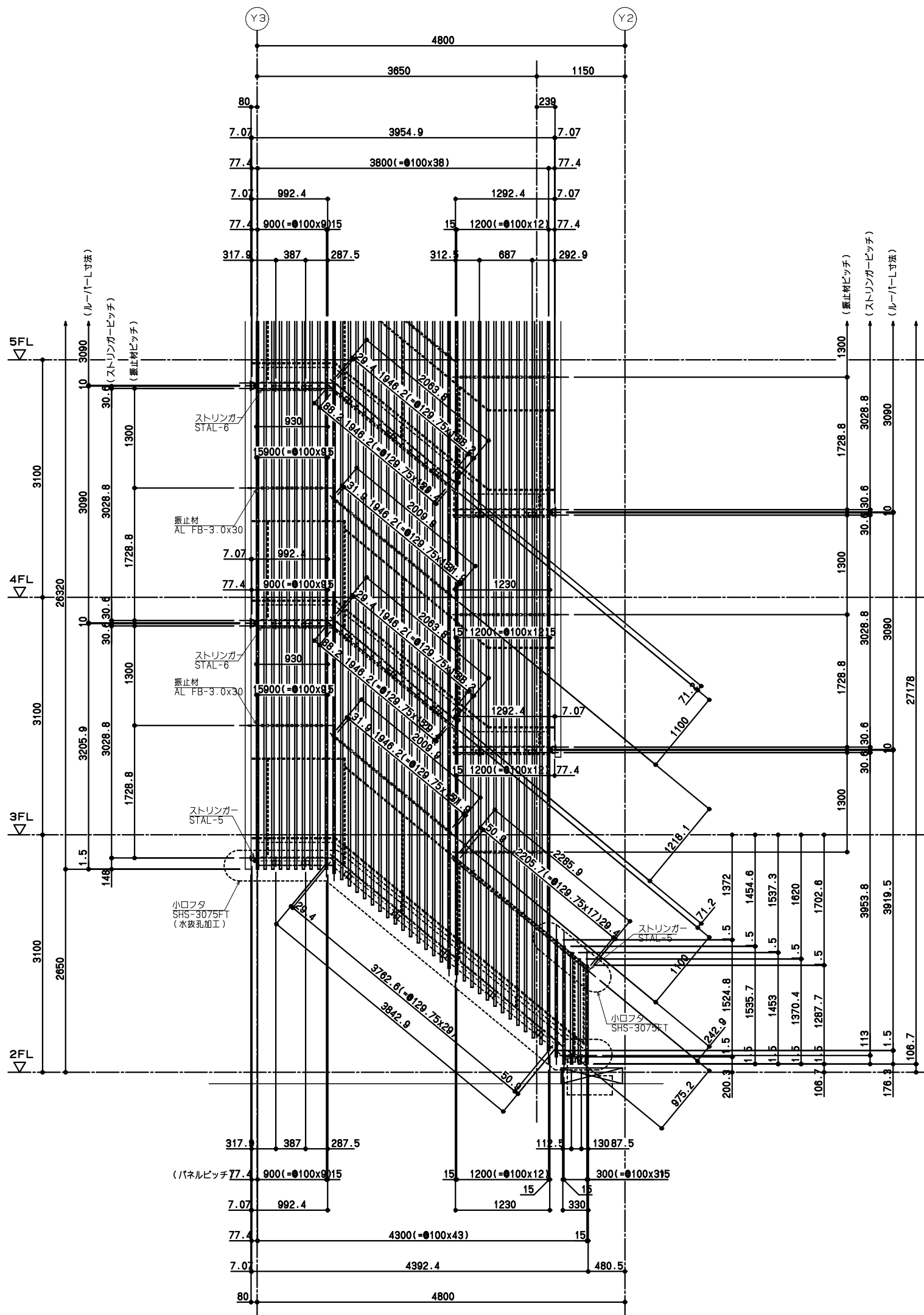
ア矢視 立面詳細図 (下部)
