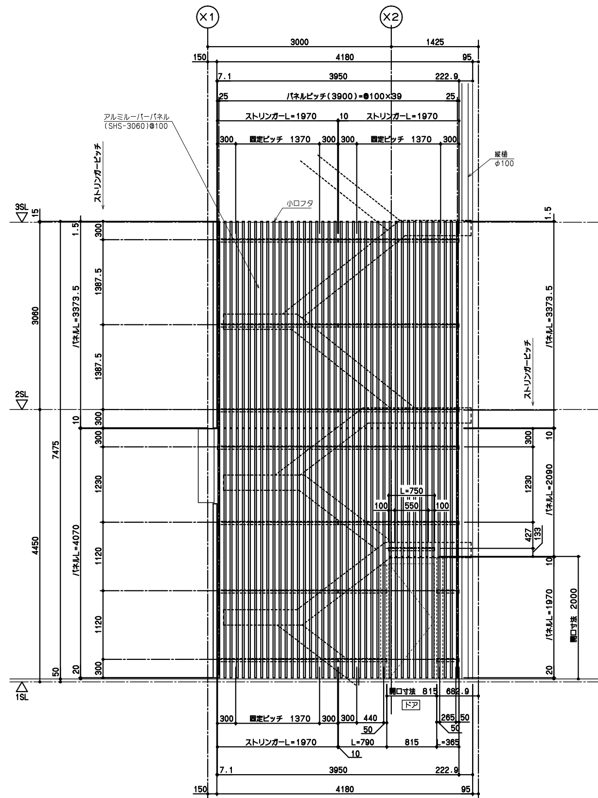
イ矢視 立面図
