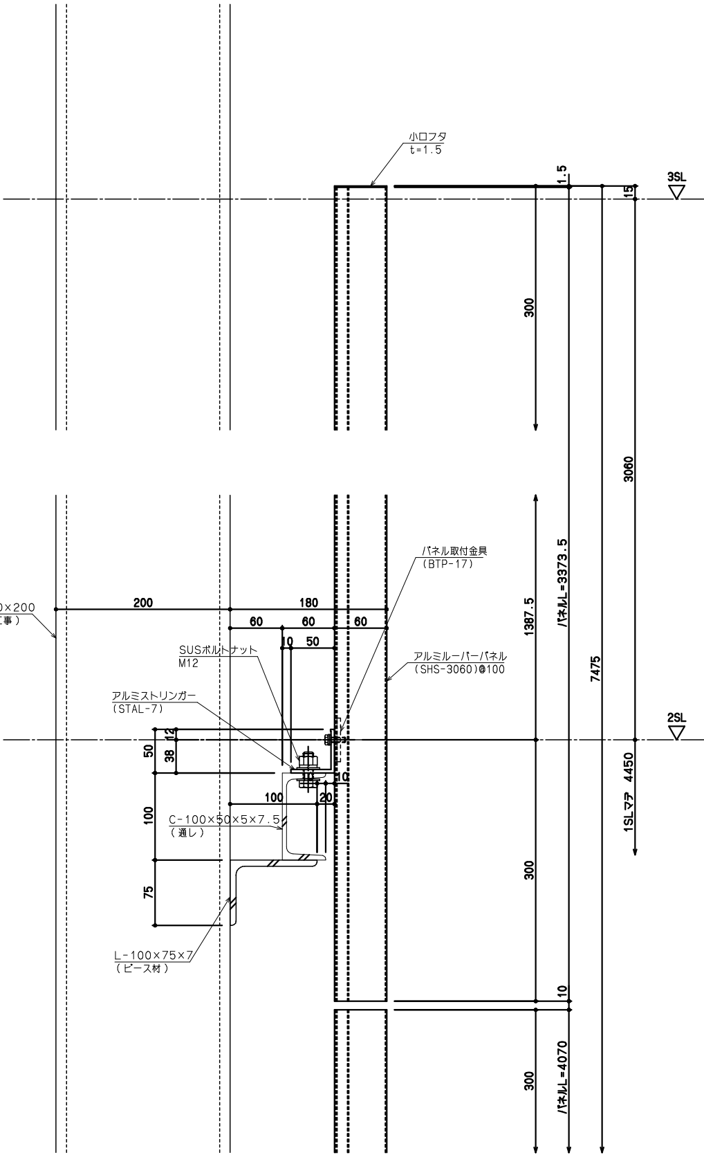
断面2 詳細図
