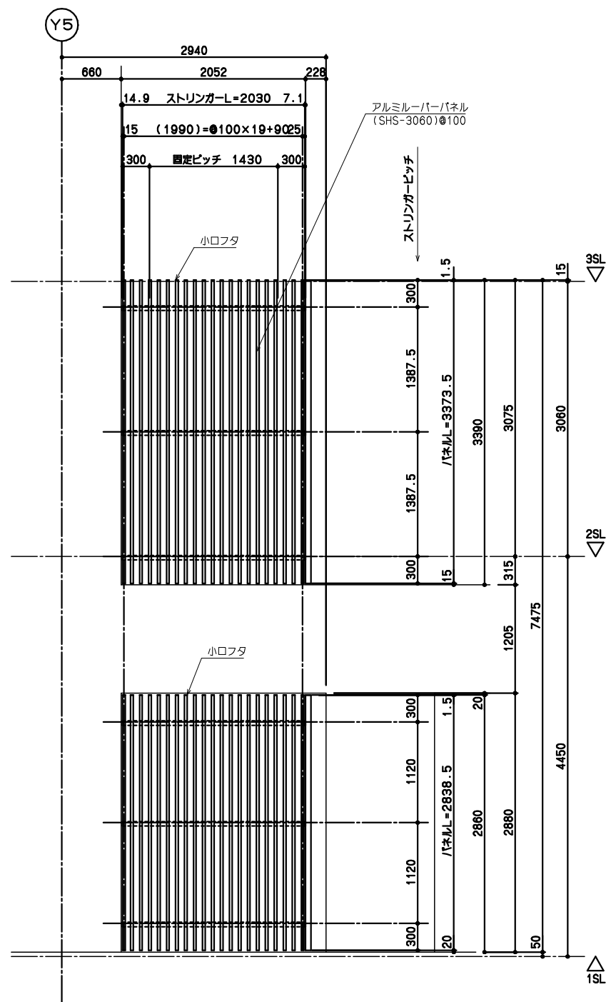
ア矢視 立面図
