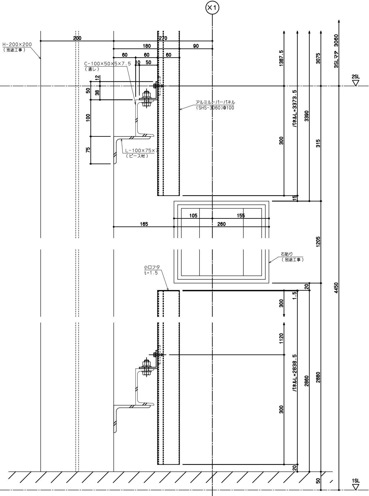
断面1 詳細図
