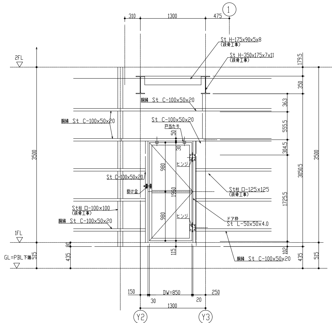
【胴縁・ドア枠 立面図】
