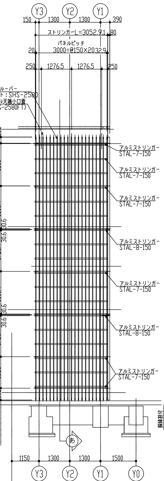
A 立面矢視図
