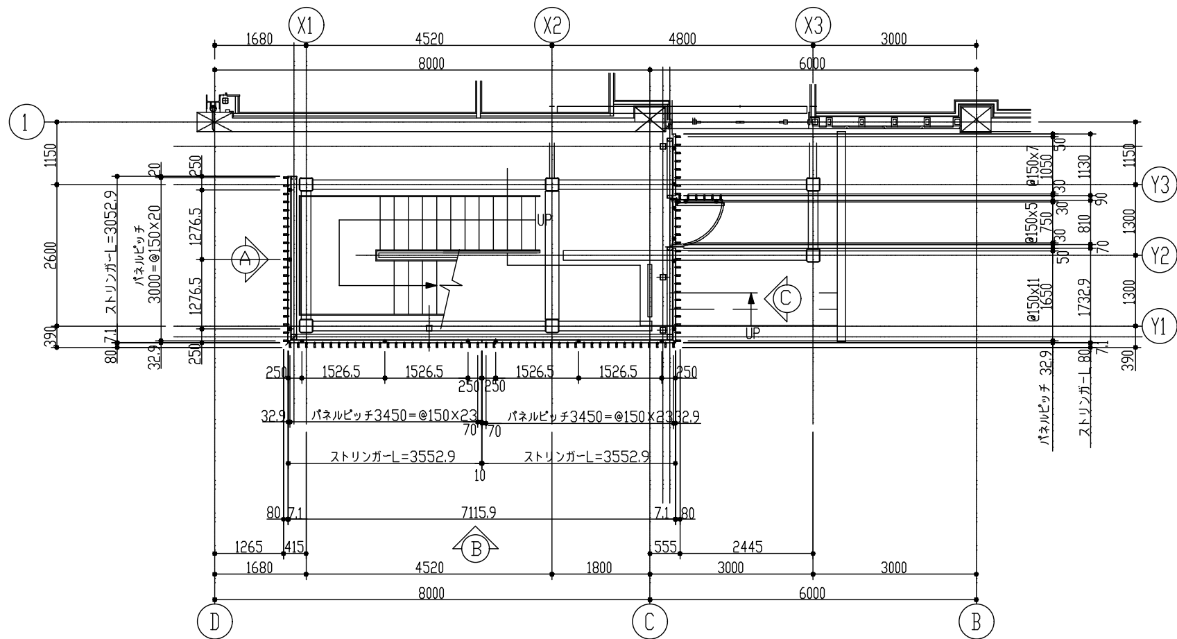
1階 平面図
