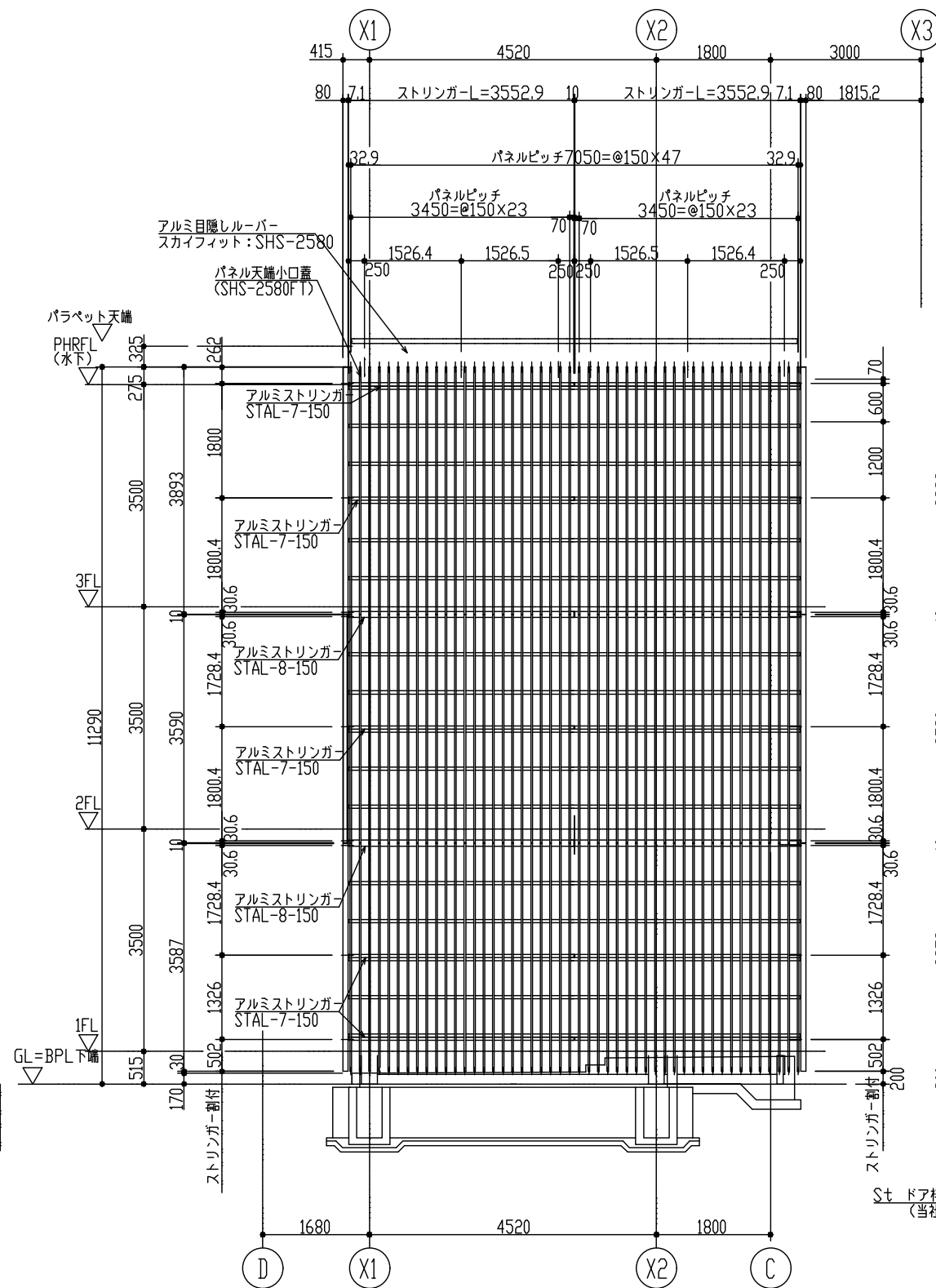
B 立面矢視図
