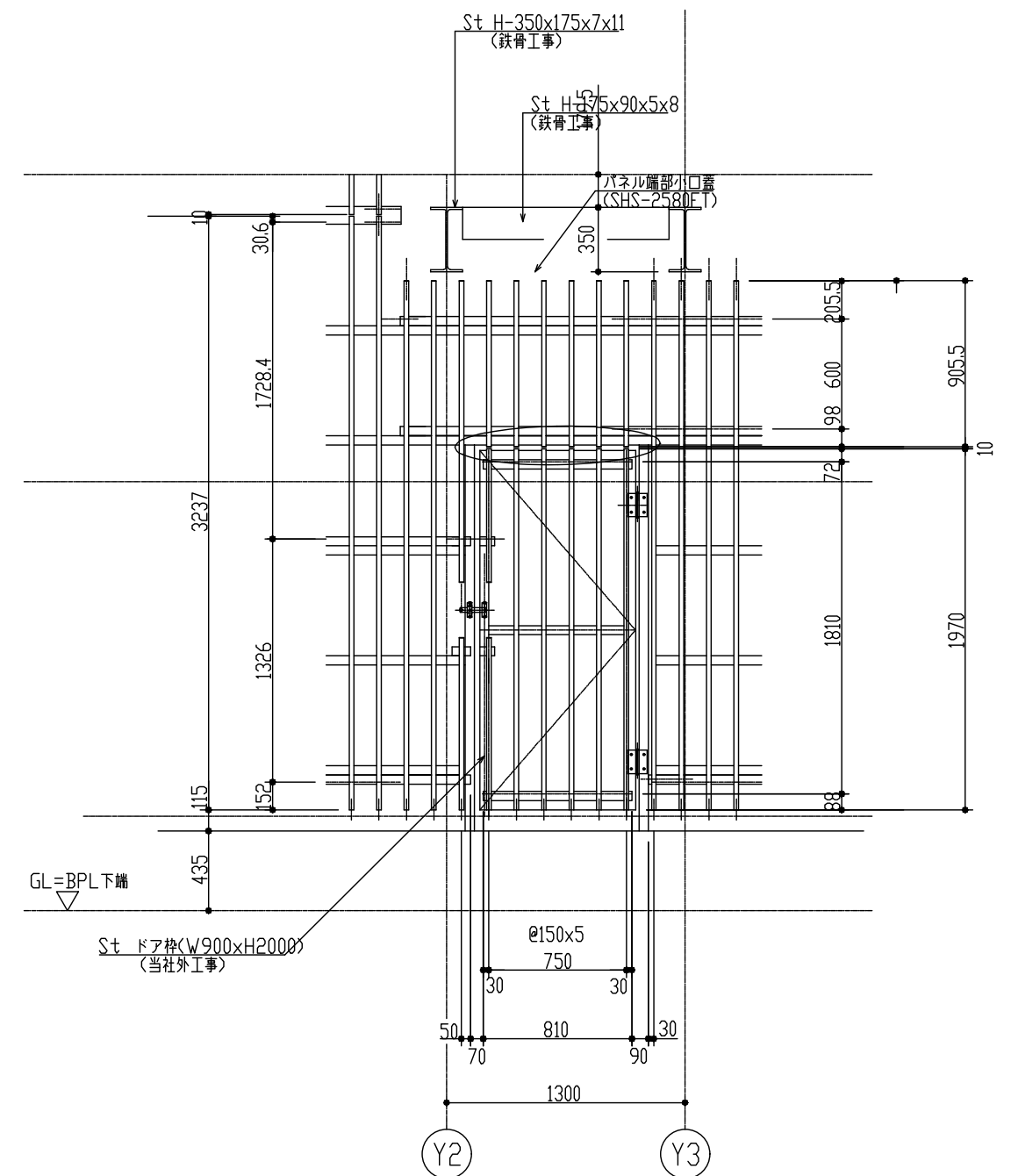
【ドア廻り 立面図】
