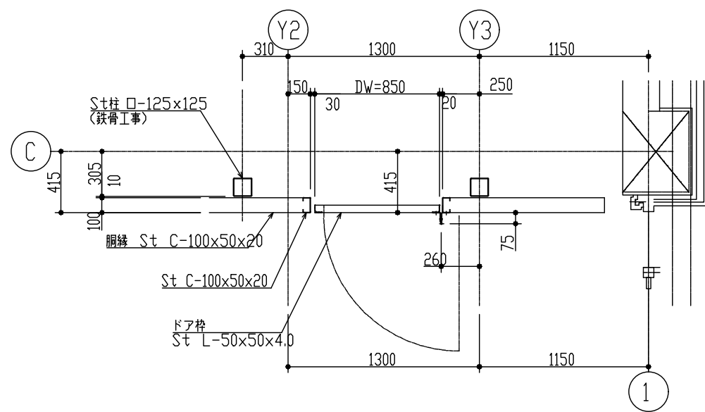
【胴縁・ドア枠 平面図】
