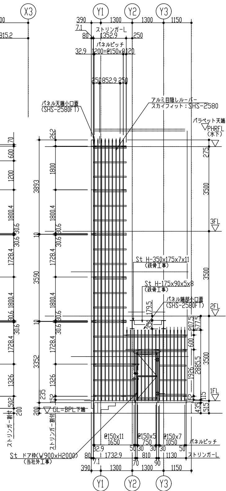
C 立面矢視図
