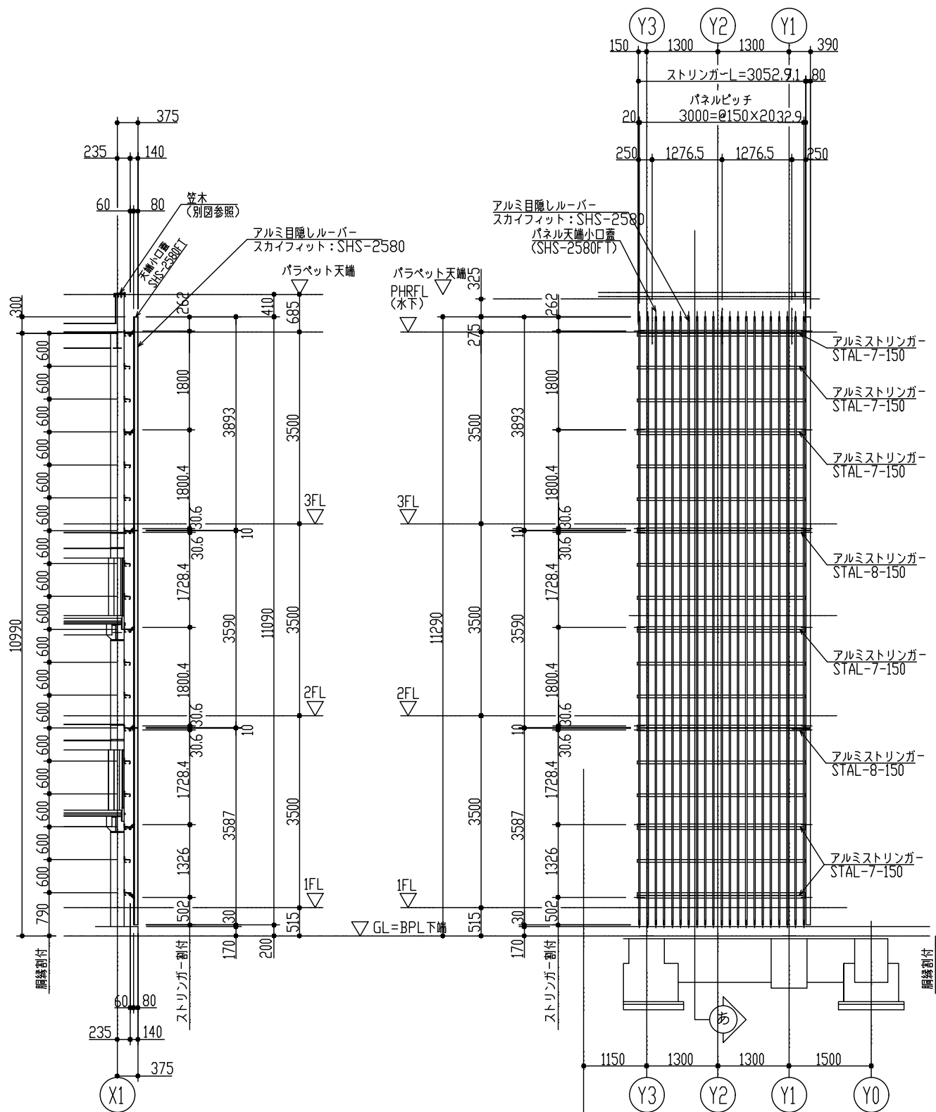
あ 断面図
