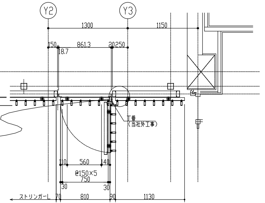
【ドア周り 平面図】
