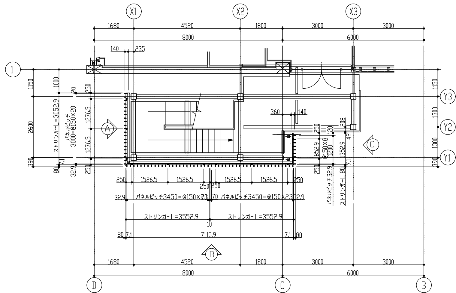
3階 平面図
