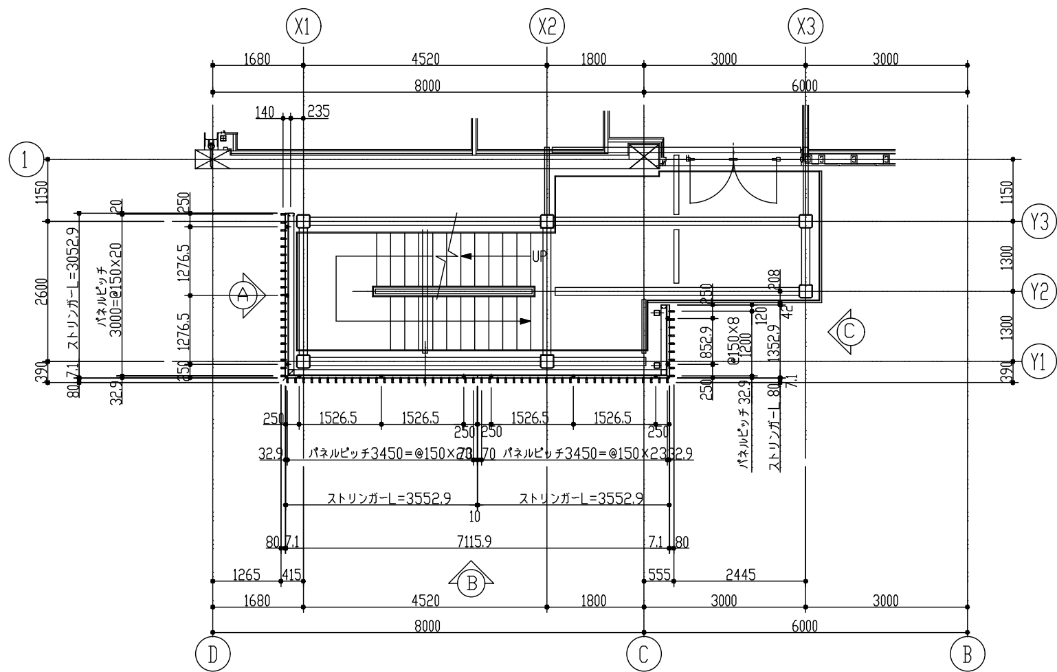
2階 平面図
