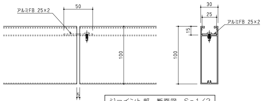
ジョイント部 断面図 S=1/2
