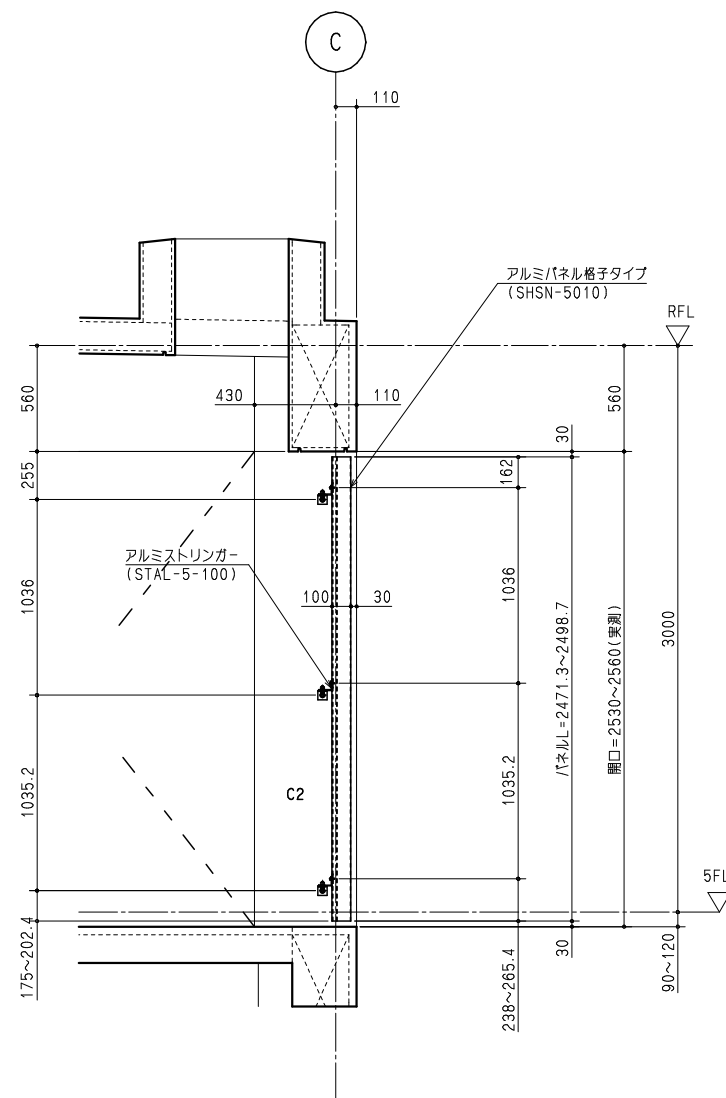
A断面図
