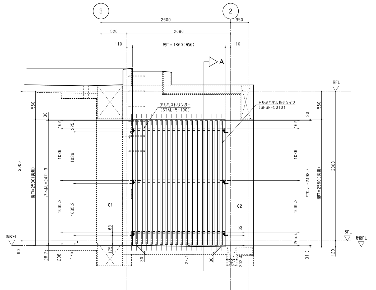
お矢視立面図
