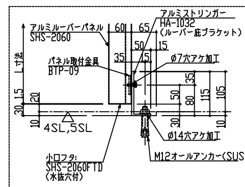
Q 部 断面図
