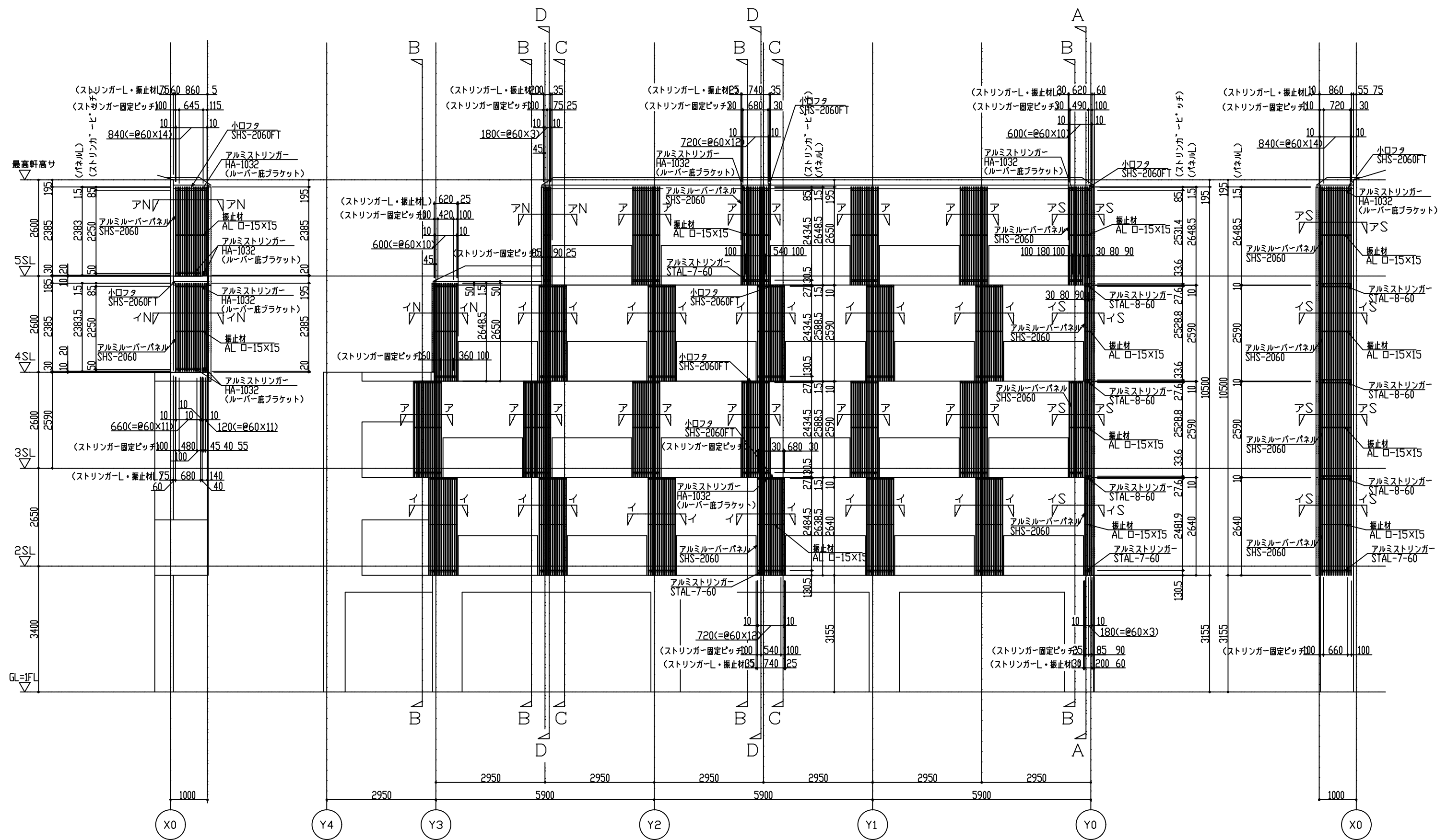
アルミルーバー 立面図
