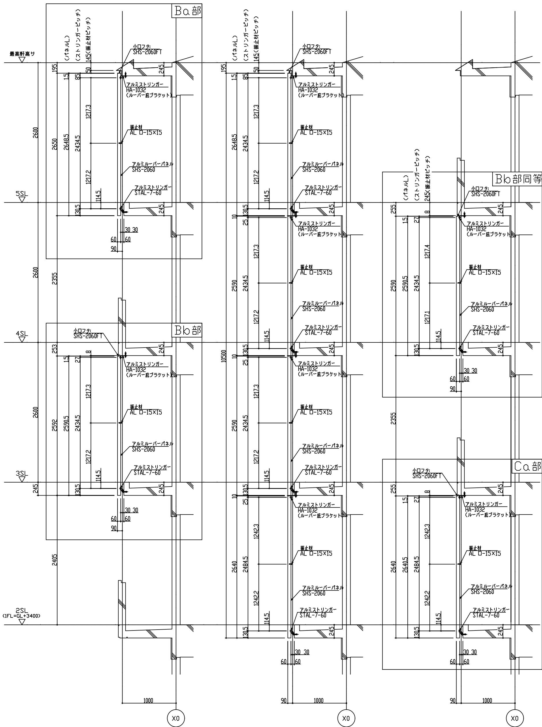
B-B断面図
