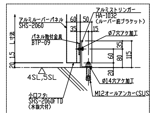
ㄋ部 断面図
