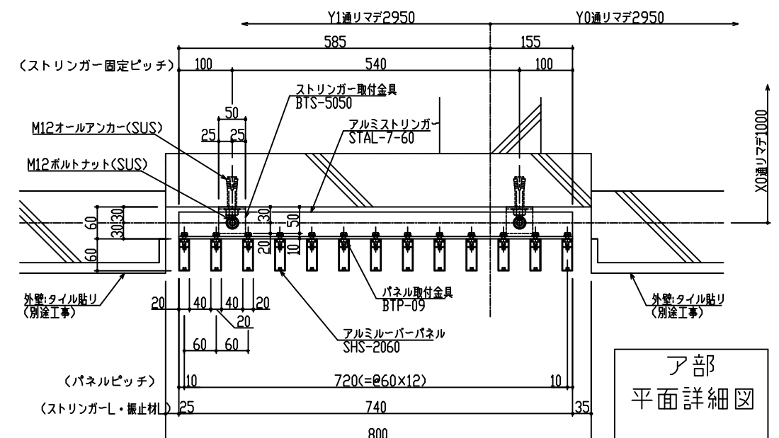
アN部 平面詳細図
