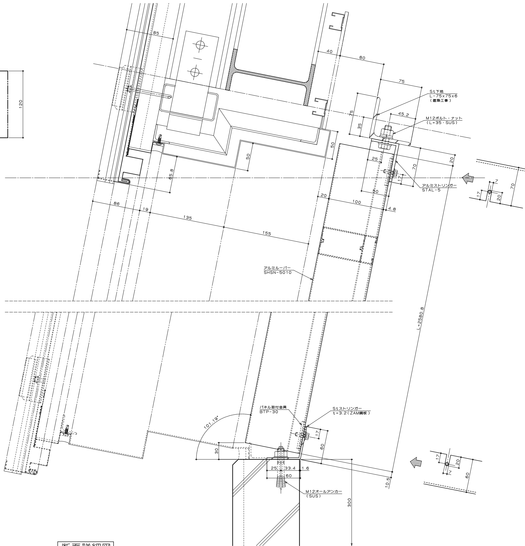
断面詳細図
