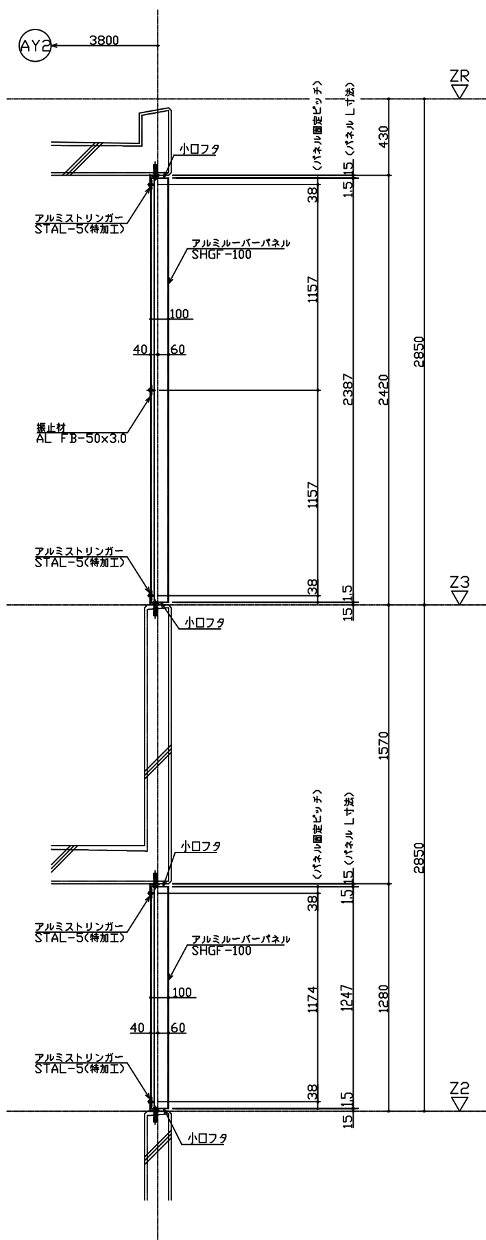
断面図
