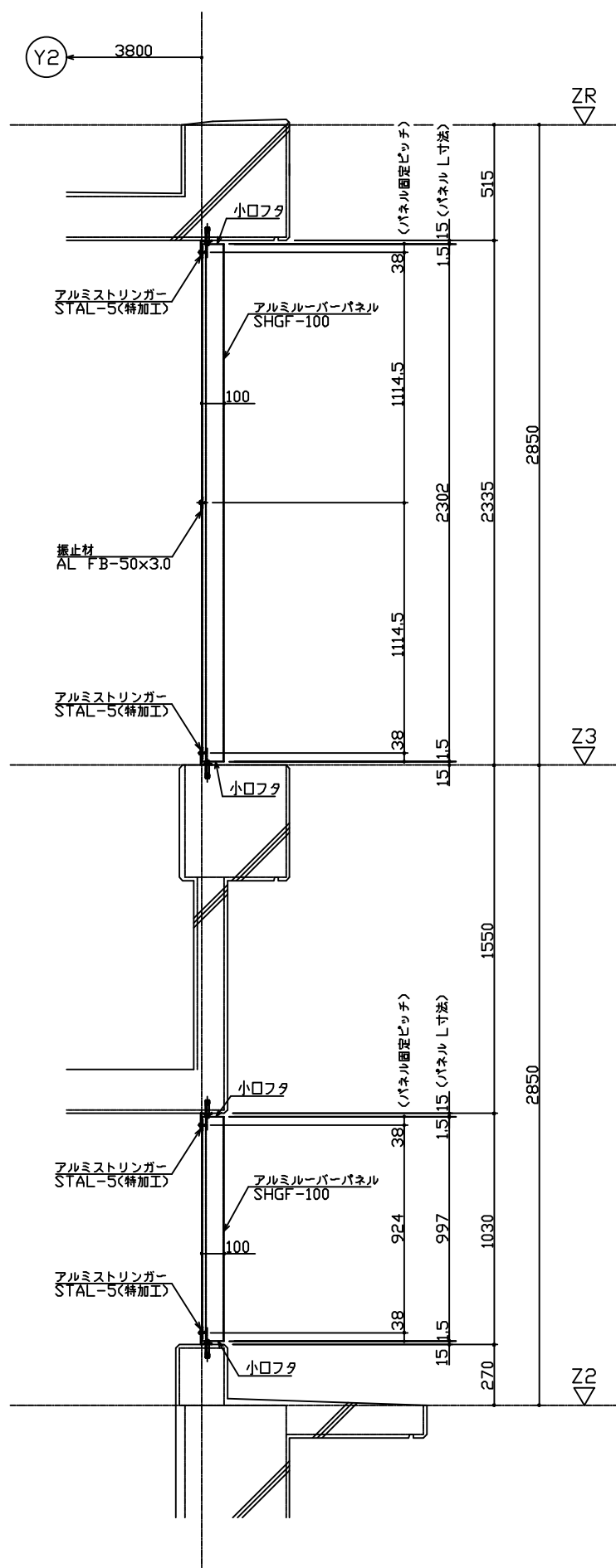
断面図
