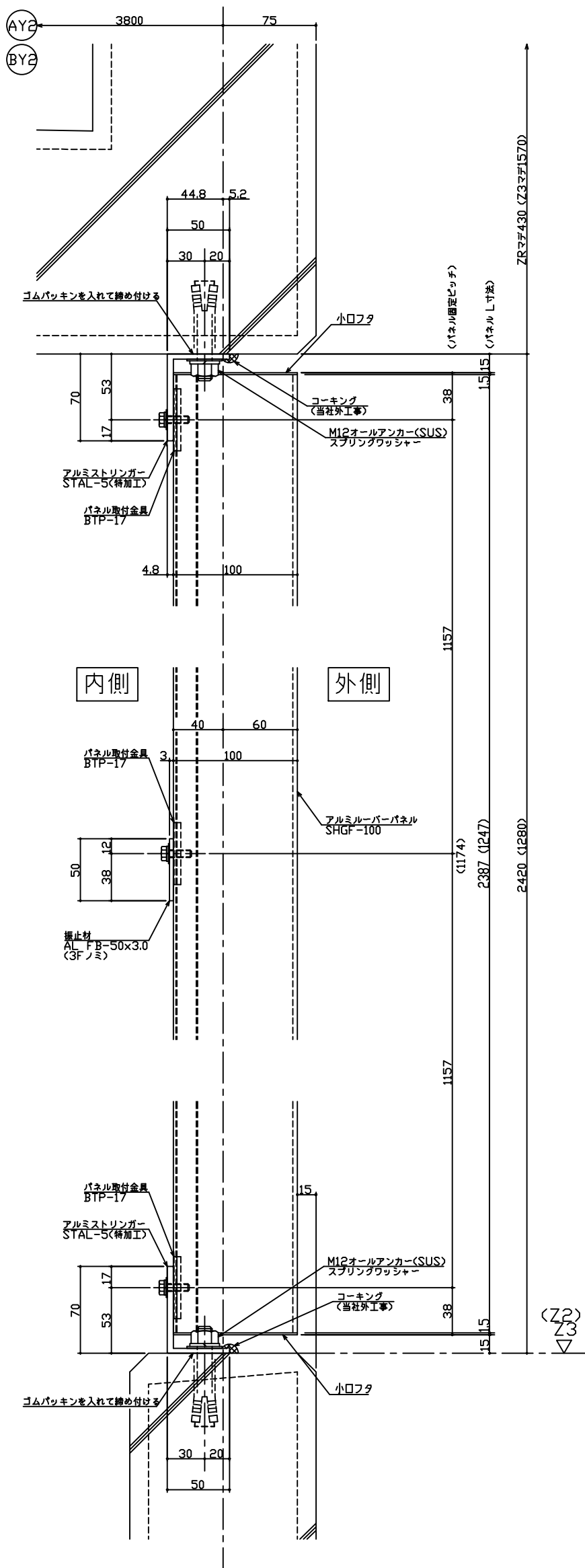
断面詳細図
