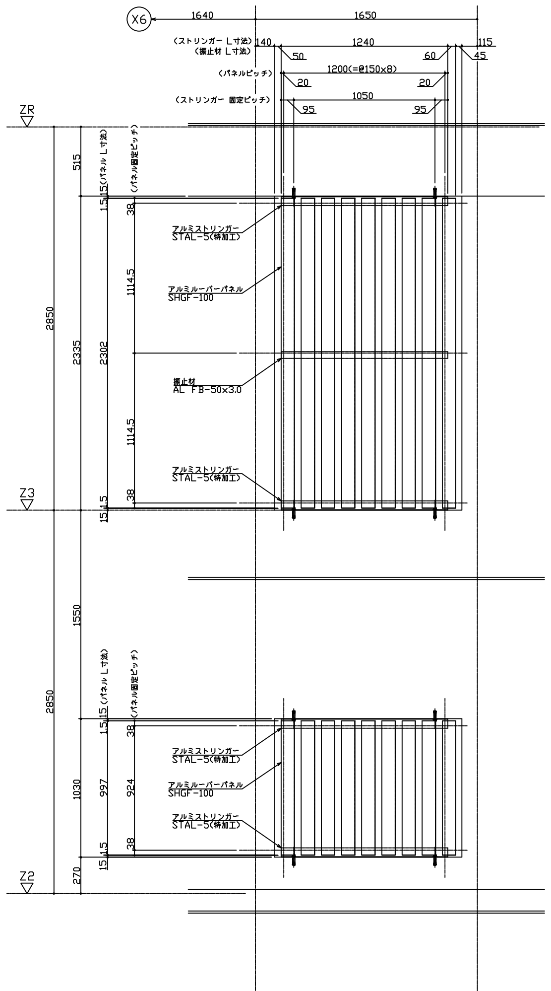
立面図
