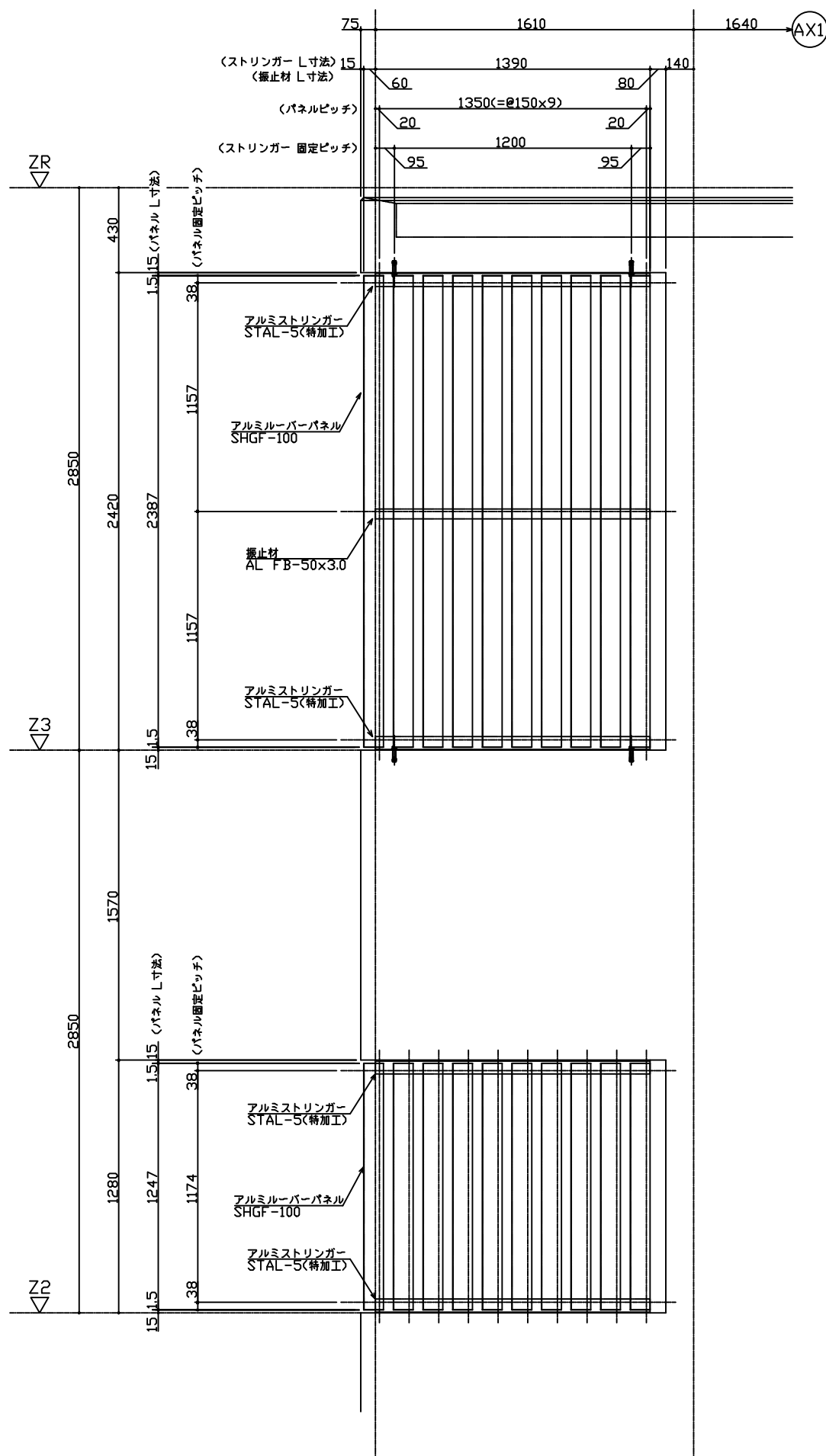
立面図
