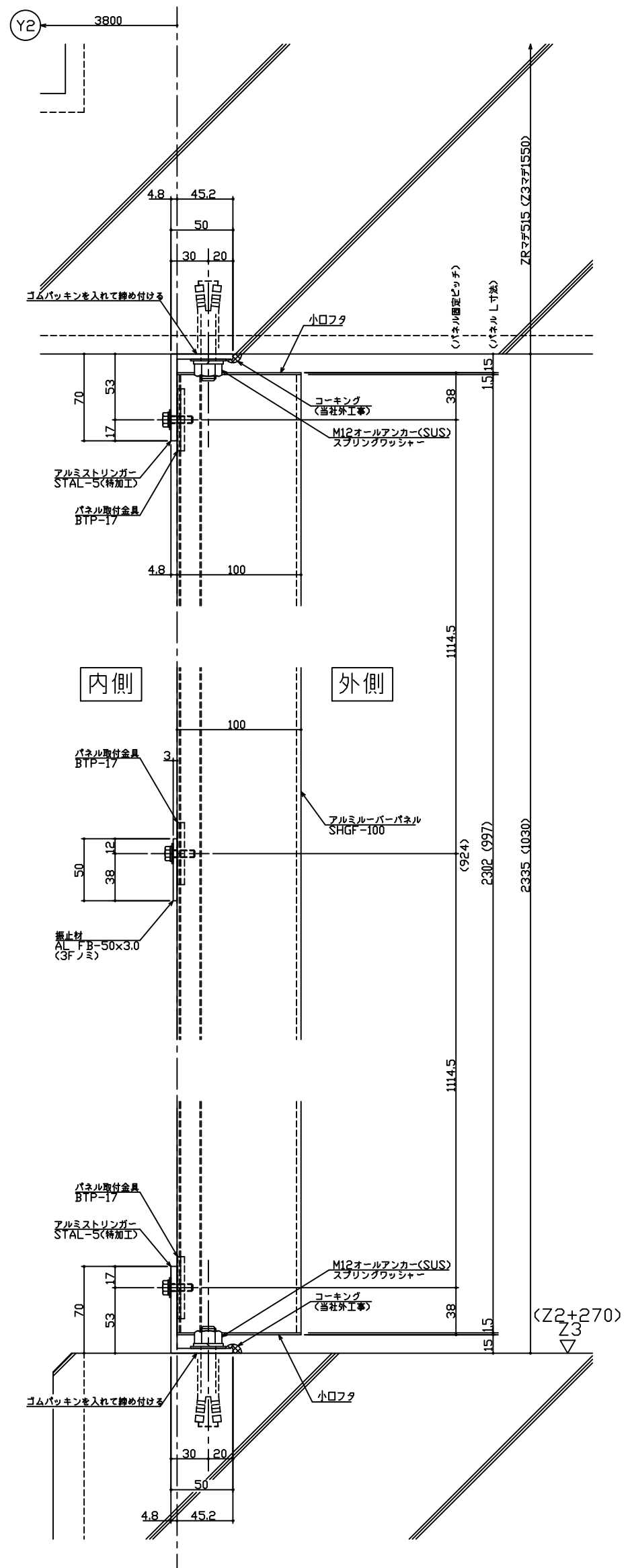
断面詳細図
