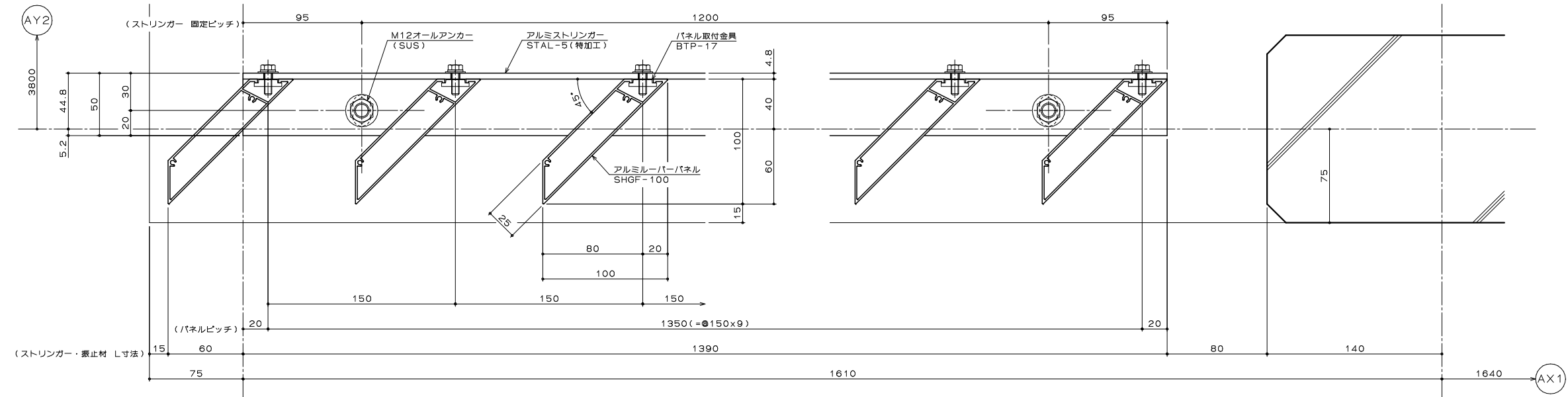
平面詳細図
