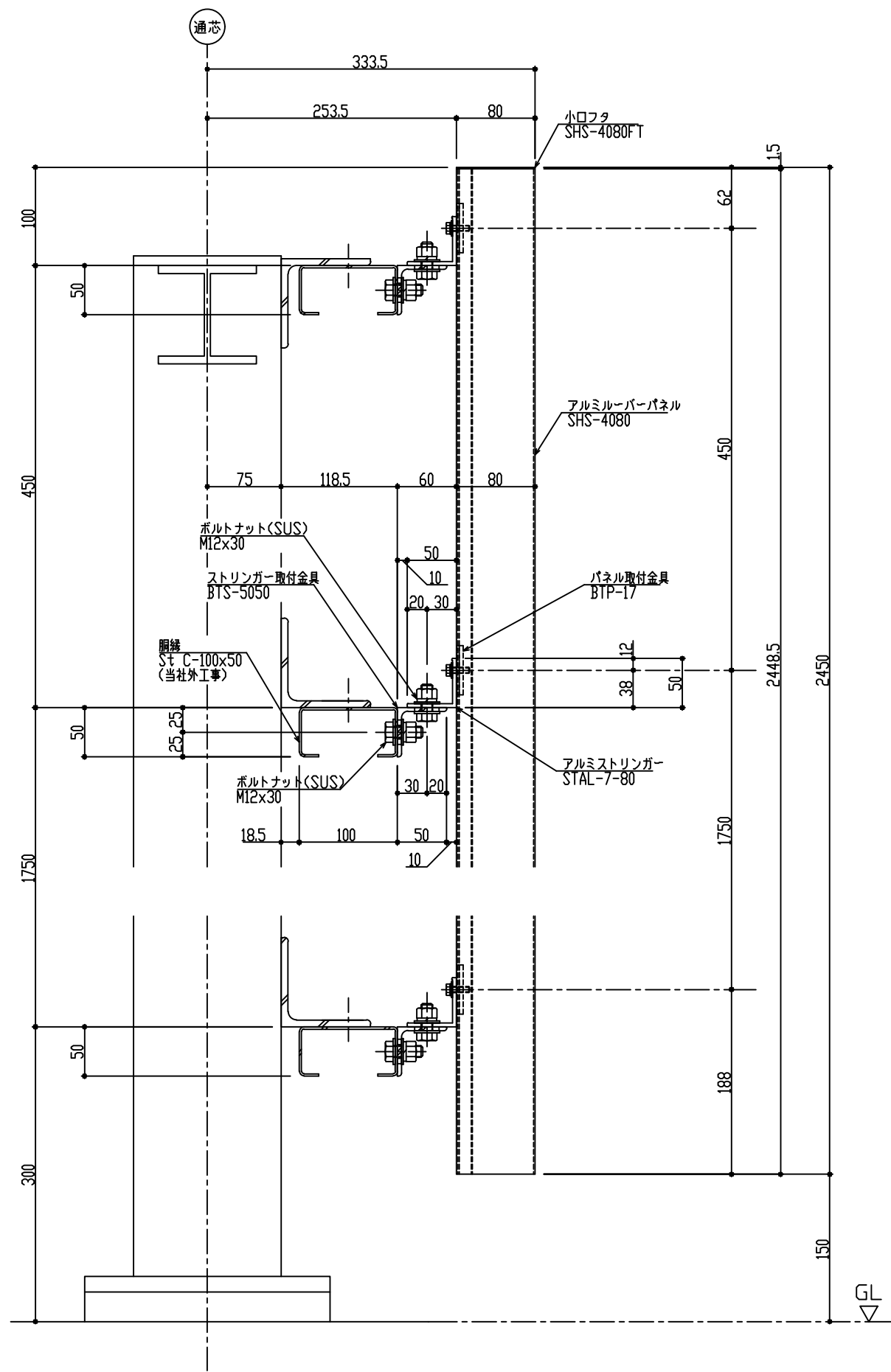
タテ 断面詳細図
