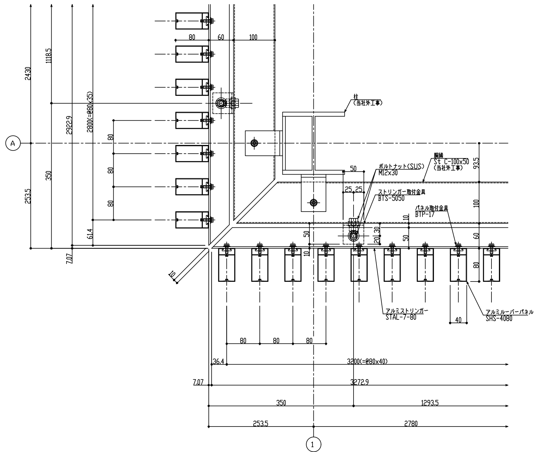
ヨコ 断面詳細図
