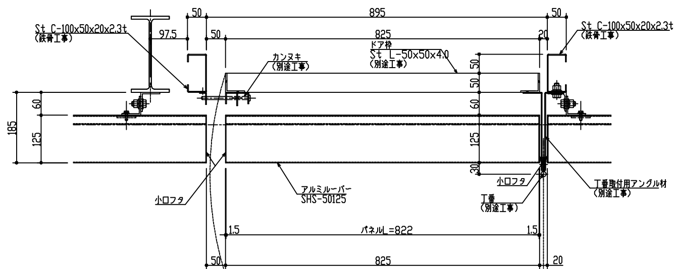
アルミルーバー 平面詳細図
