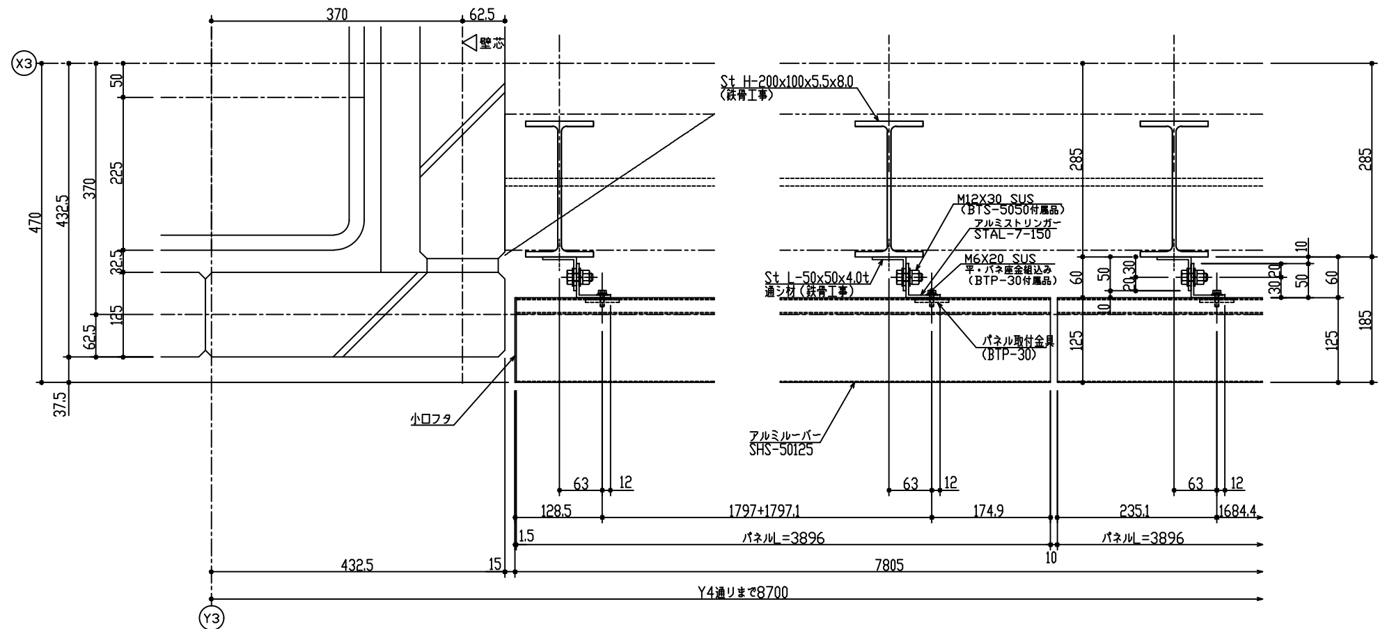
アルミルーバー 平面詳細図
