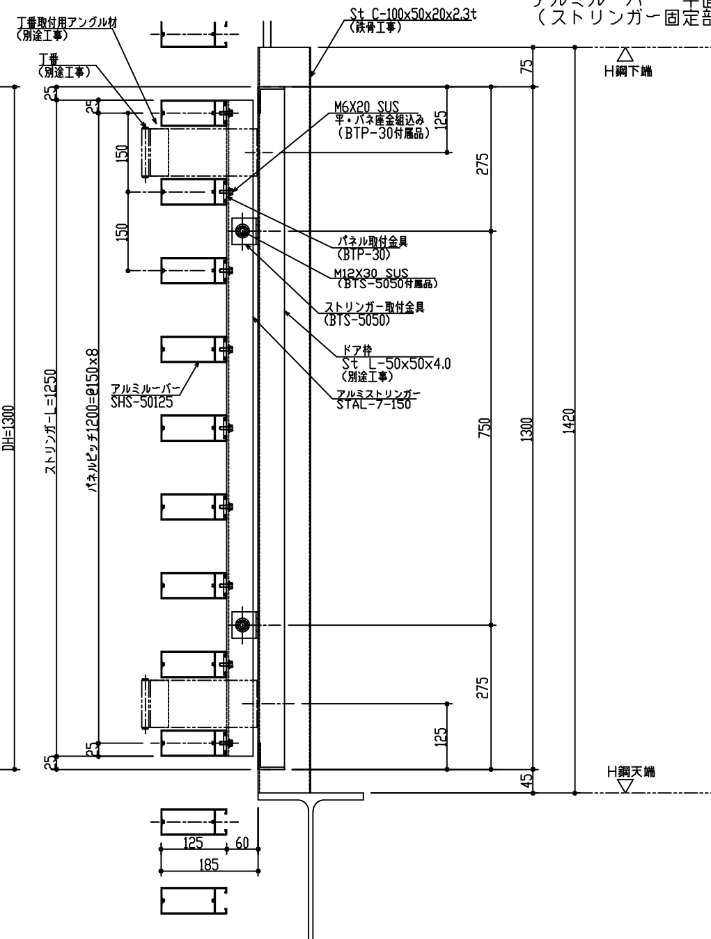
アルミルーバー 立面詳細図
