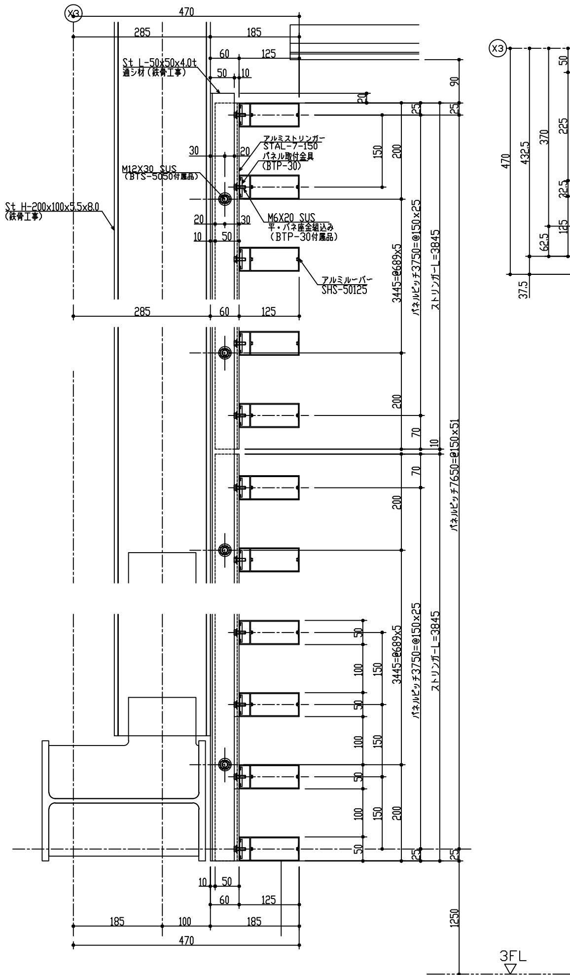
アルミルーバー 断面詳細図
