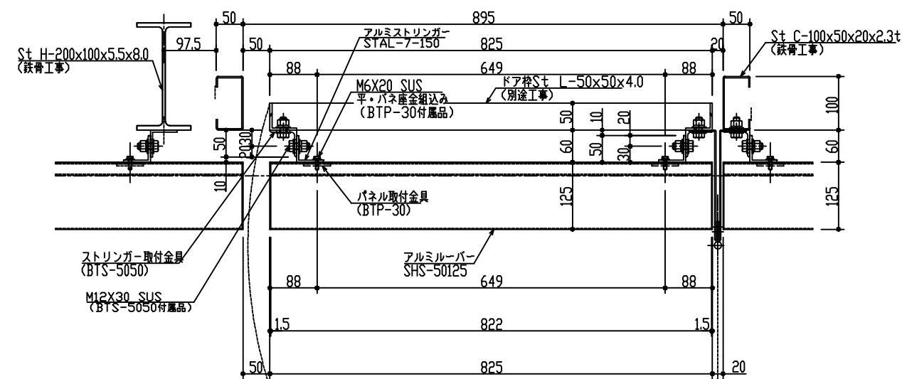
アルミルーバー 平面詳細図 (ストリッガー固定部詳細)
