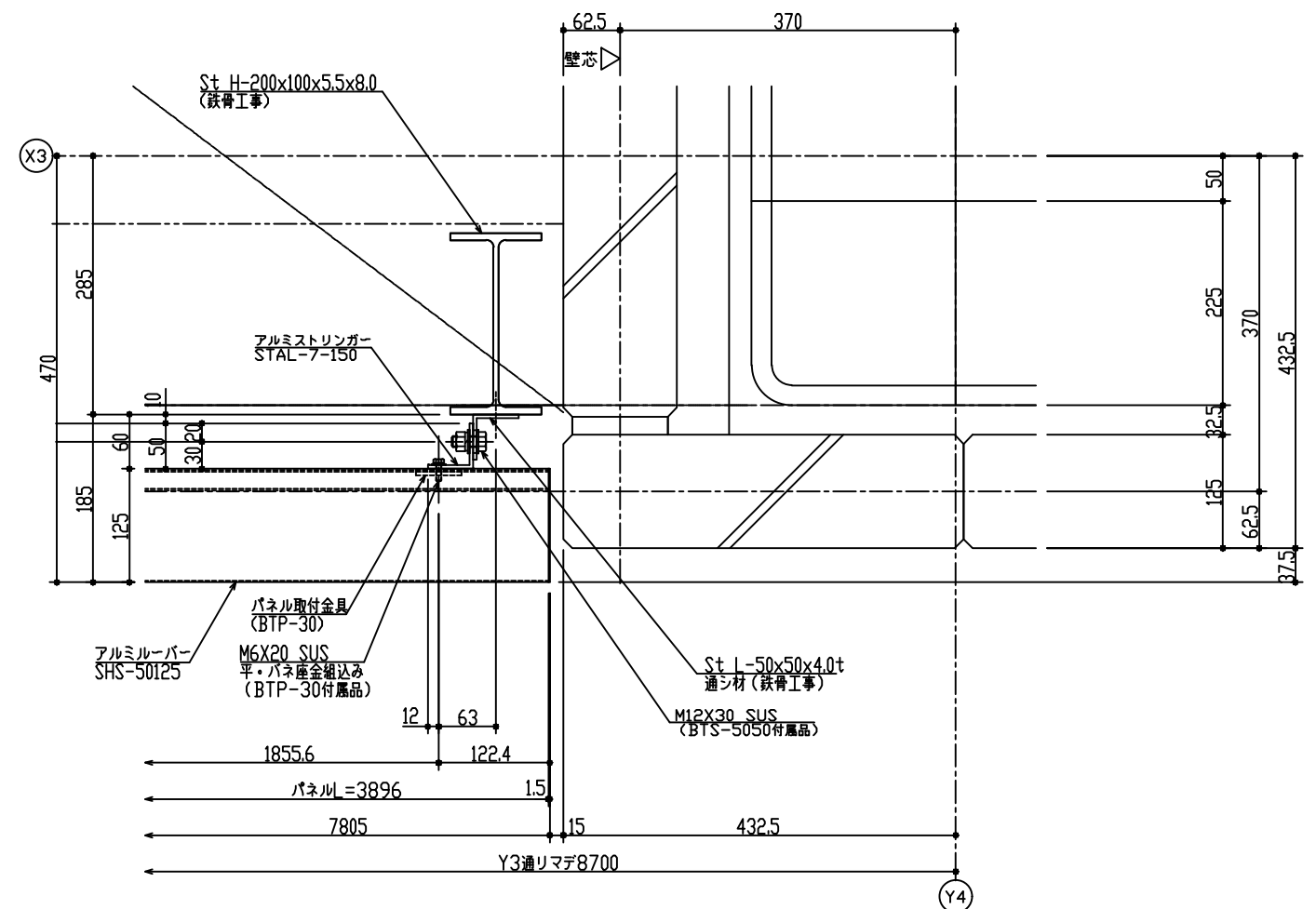
アルミルーバー 平面詳細図
