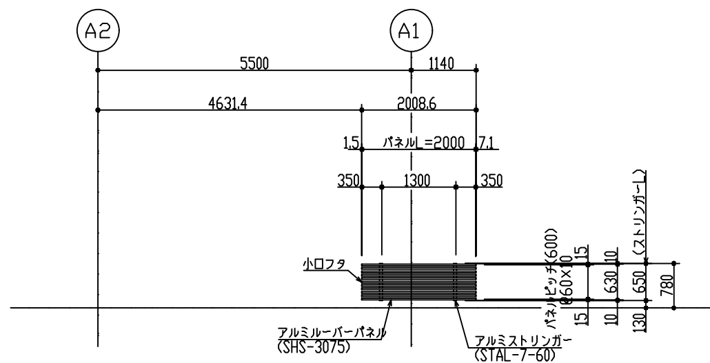
イ矢視立面図
