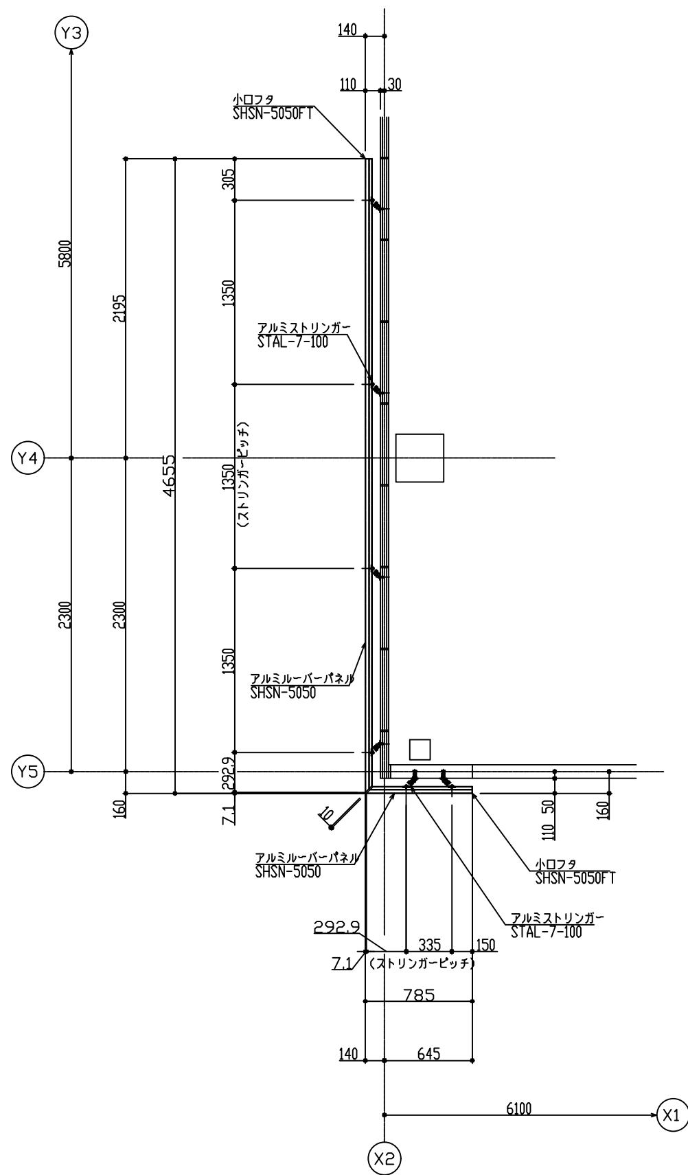
平面図
