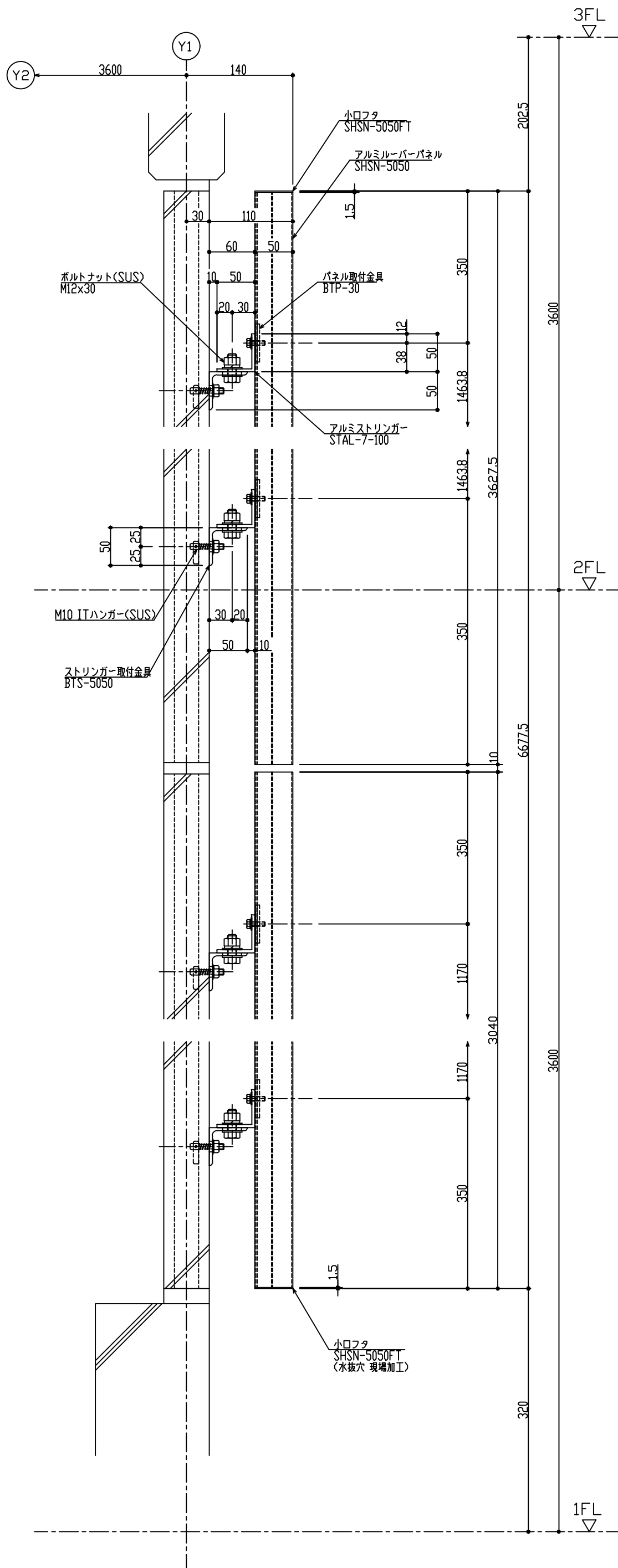
断面詳細図
