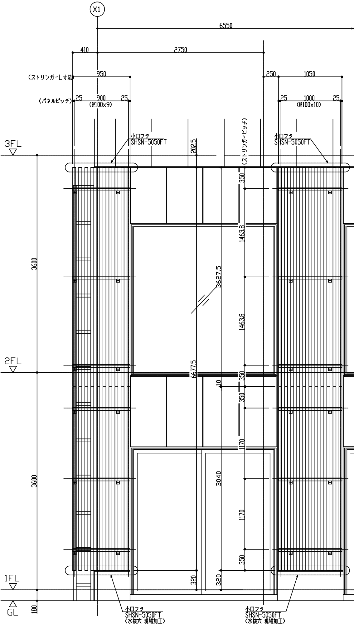
立面図 (Y1通部)
