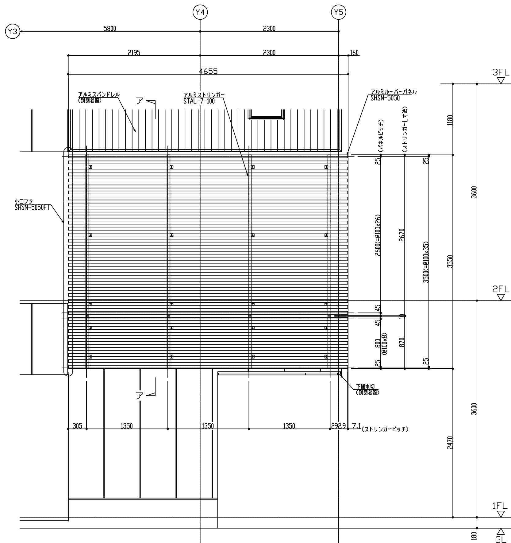
立面図 (X2通部)
