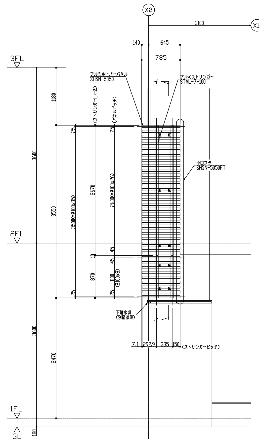
立面図 (Y5通部)
