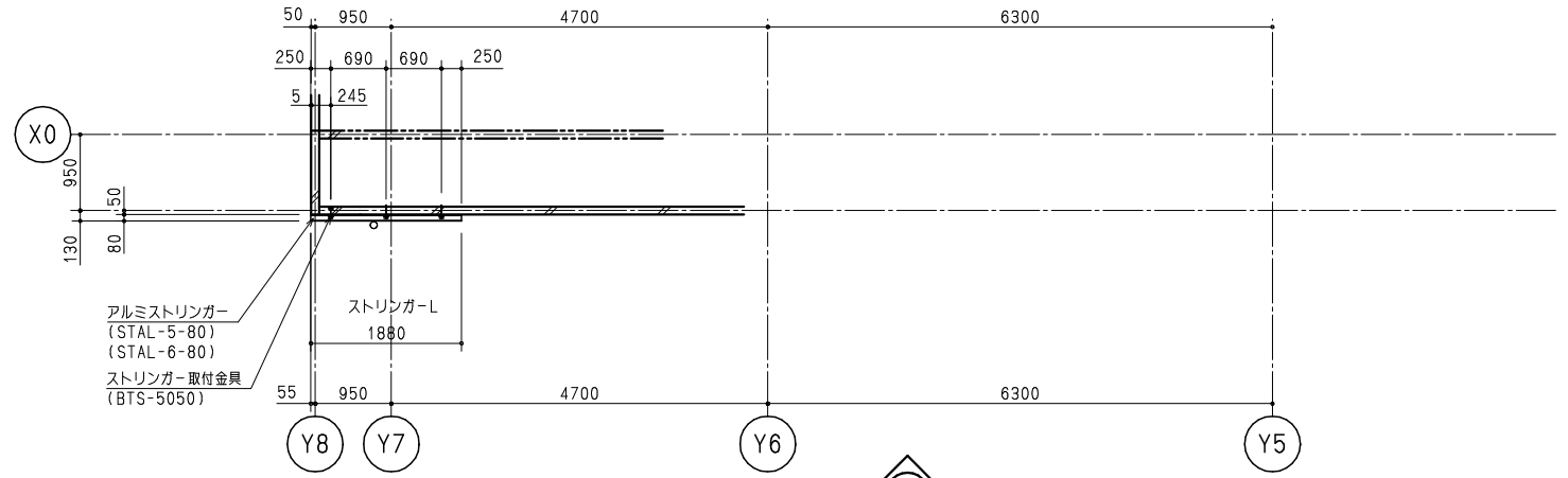
平面図
