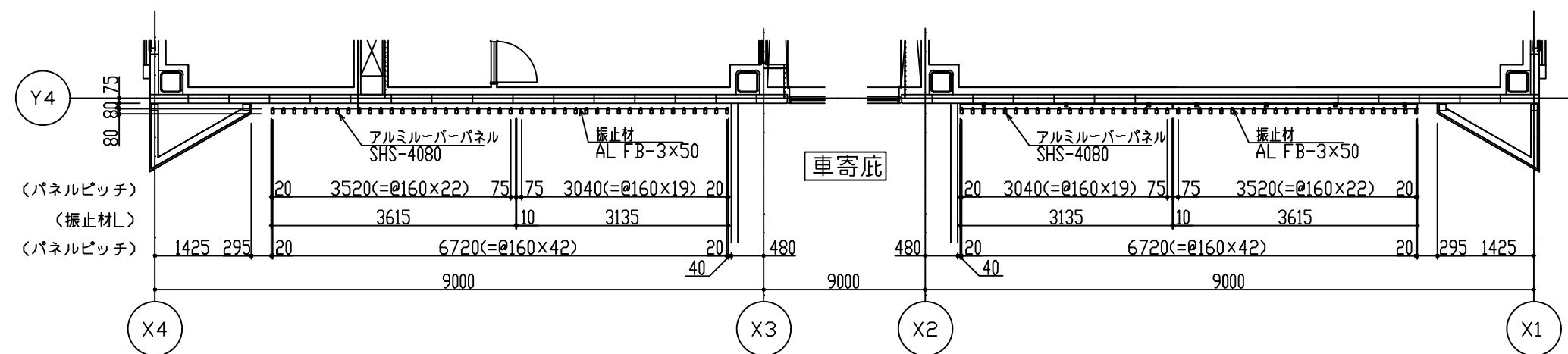
アルミルーバー イーイ平面図
