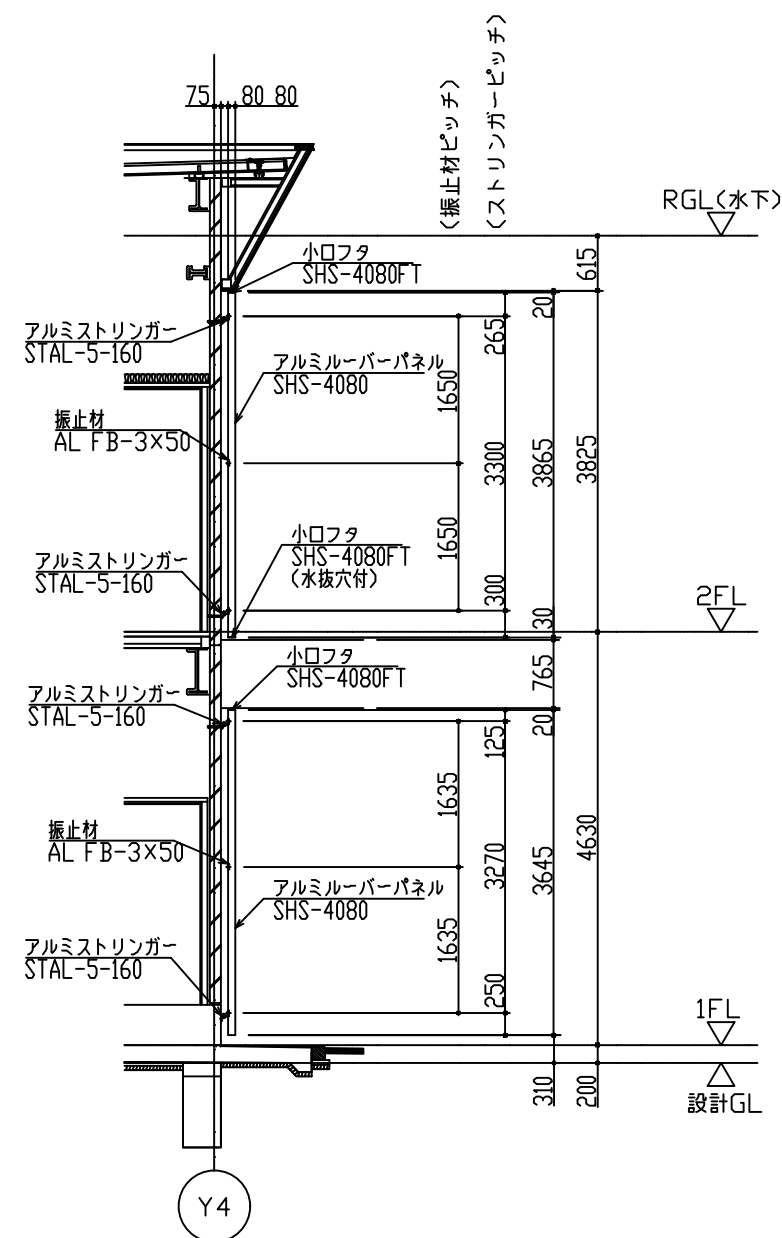
アルミルーバー B-B断面図
