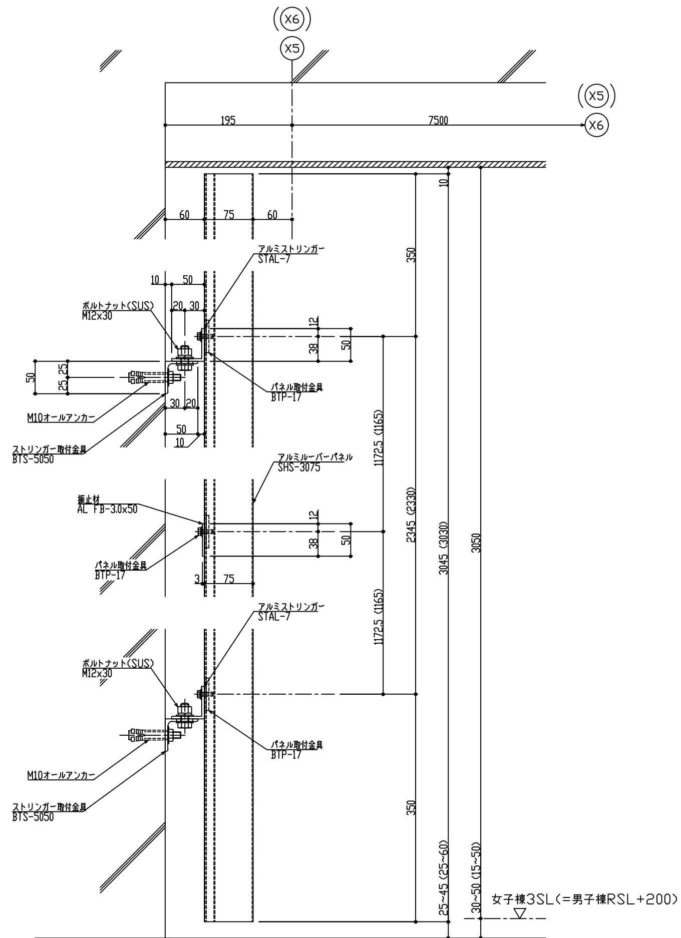
B 断面詳細図
