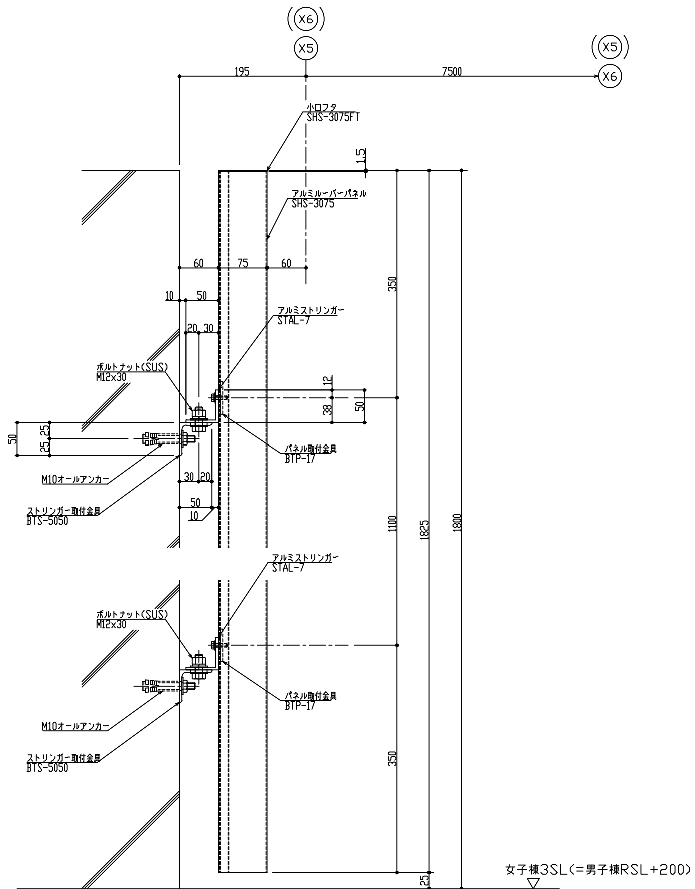
A 断面詳細図
