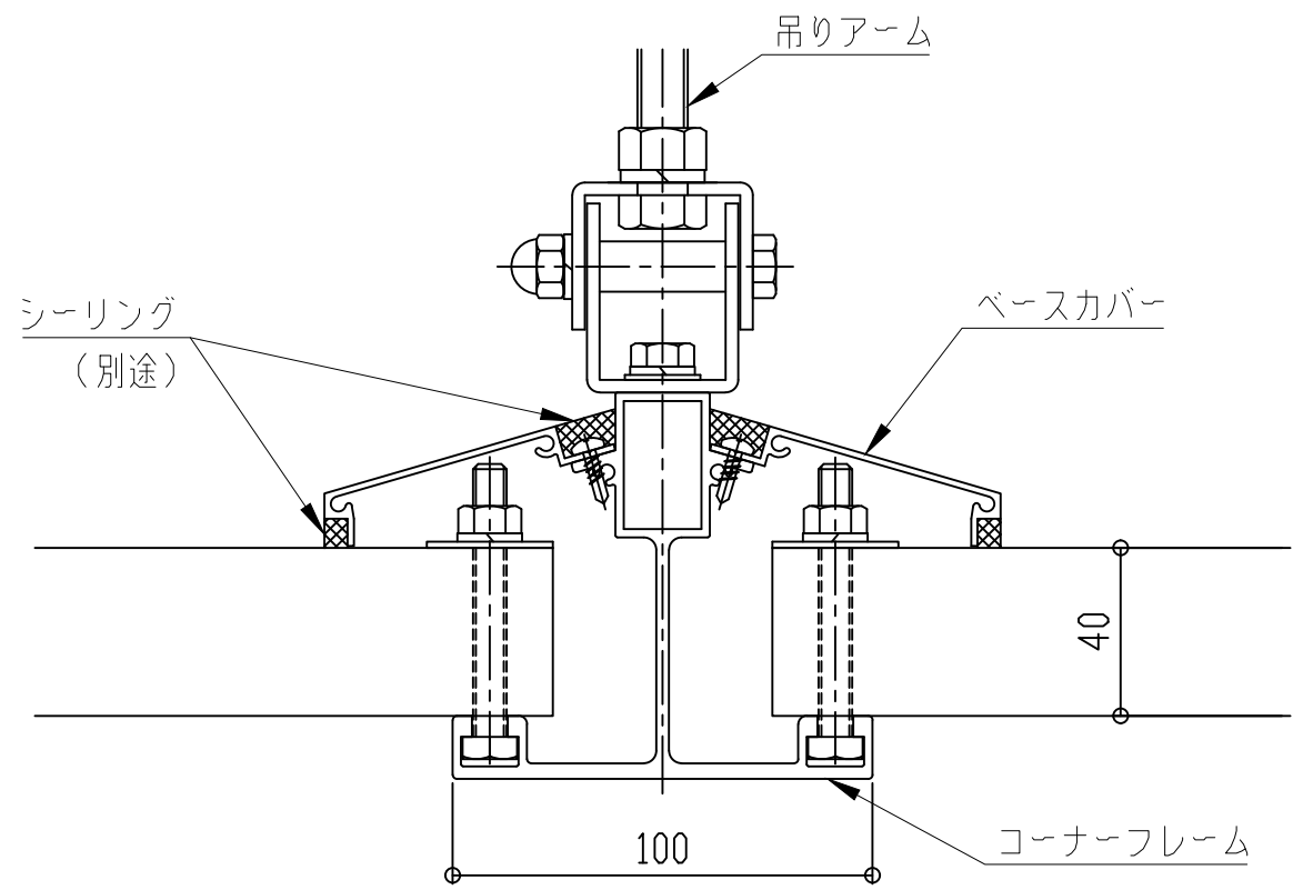
コーナーフレイム断面図
