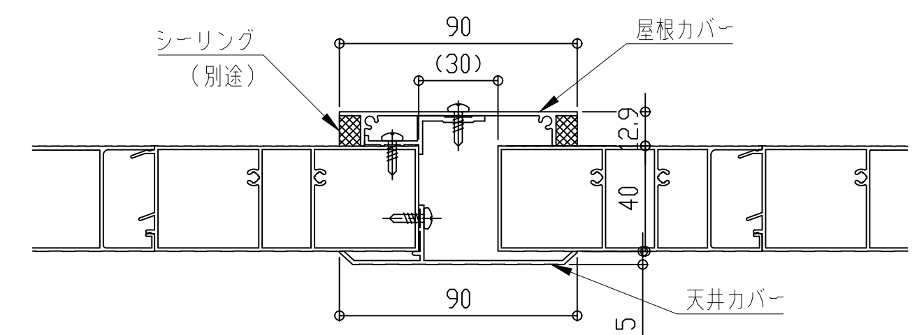
屋根カバー断面図
