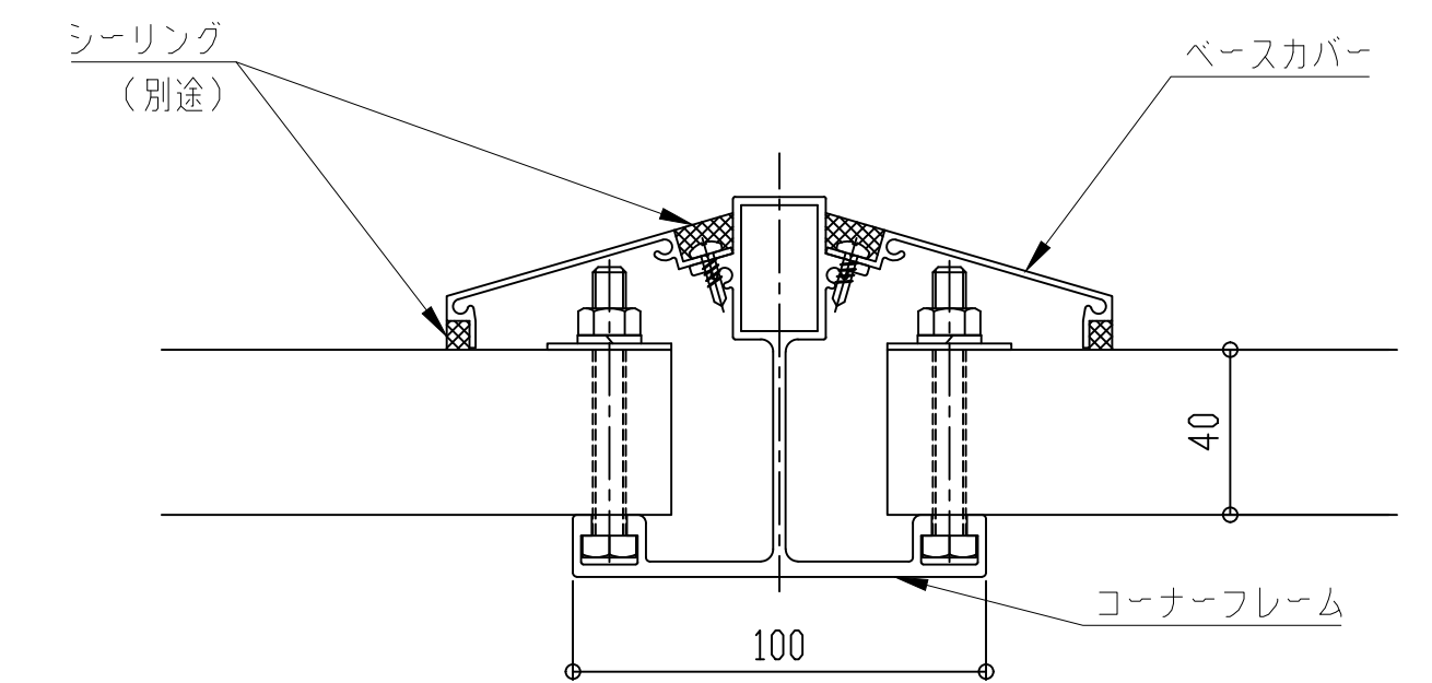
コーナーフレーム断面図
