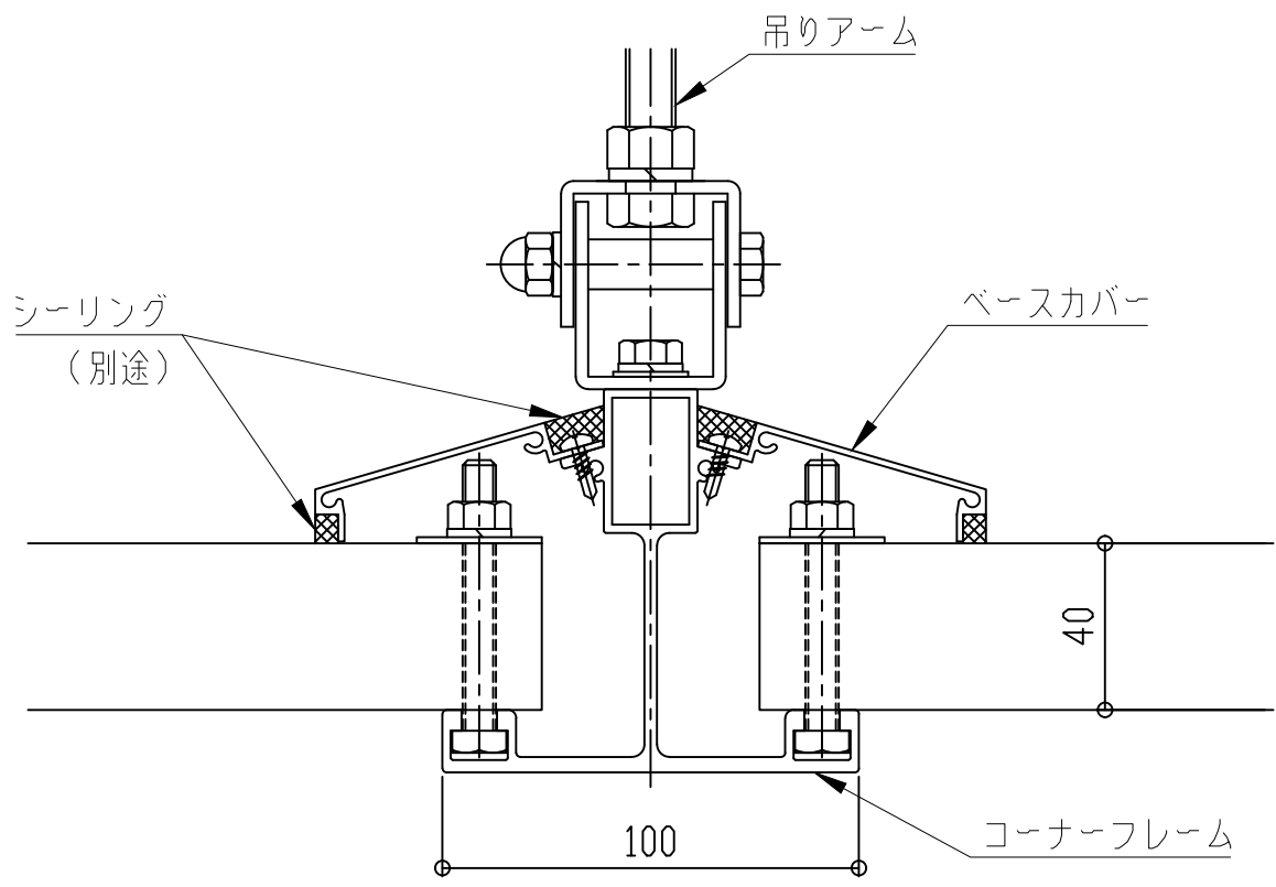
コーナフレーム断面図
