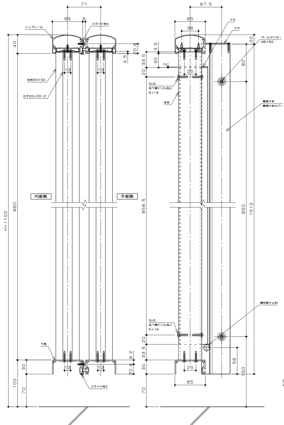
断面図 S = 1/4
