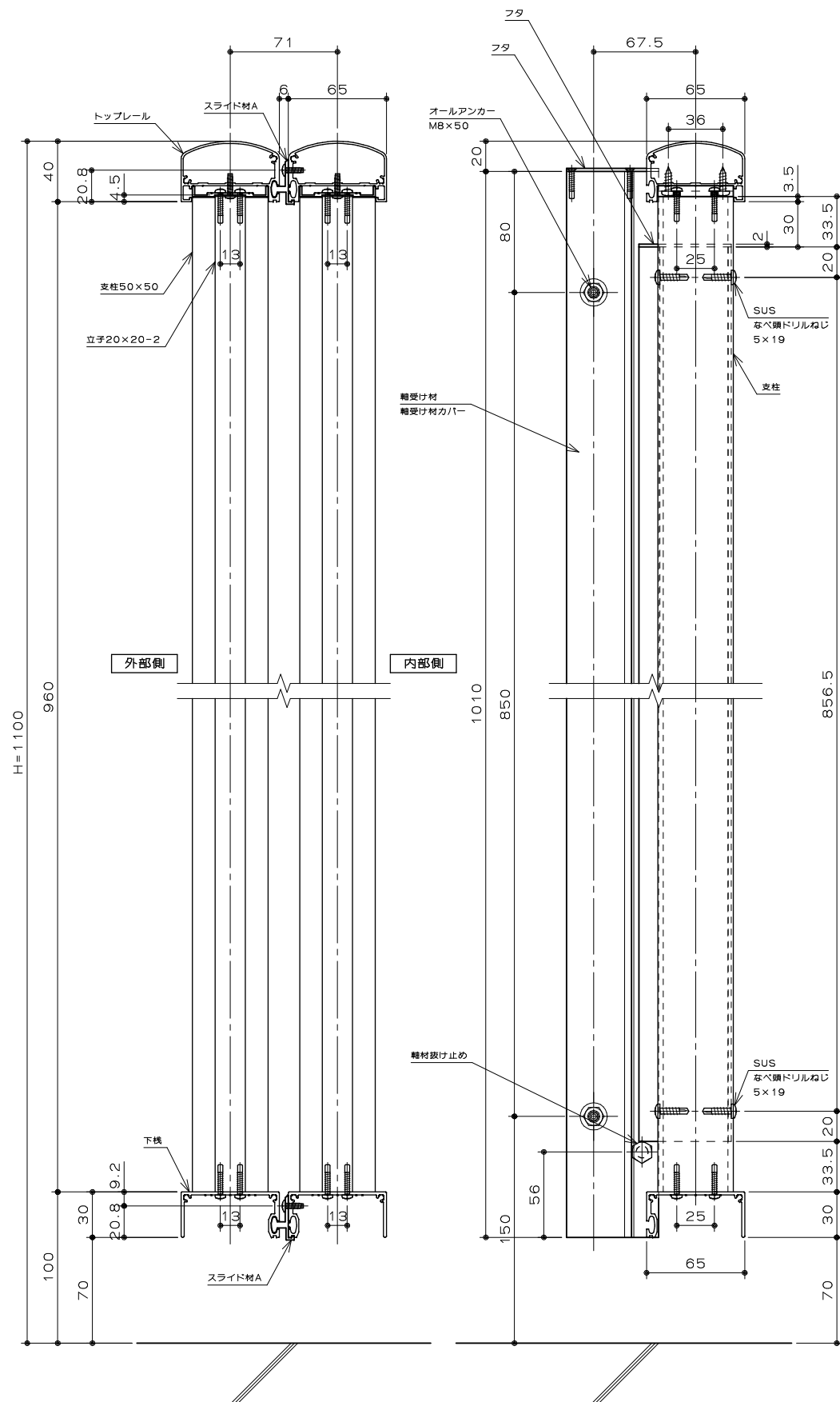
あ断面図 S = 1/4
