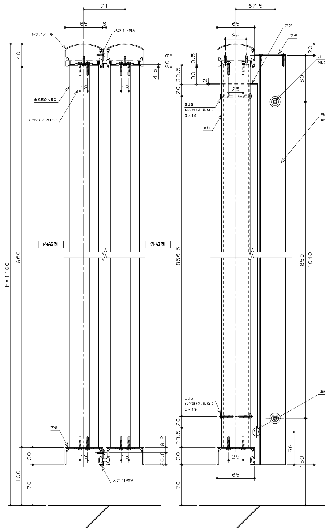
あ断面図 S=1/4
