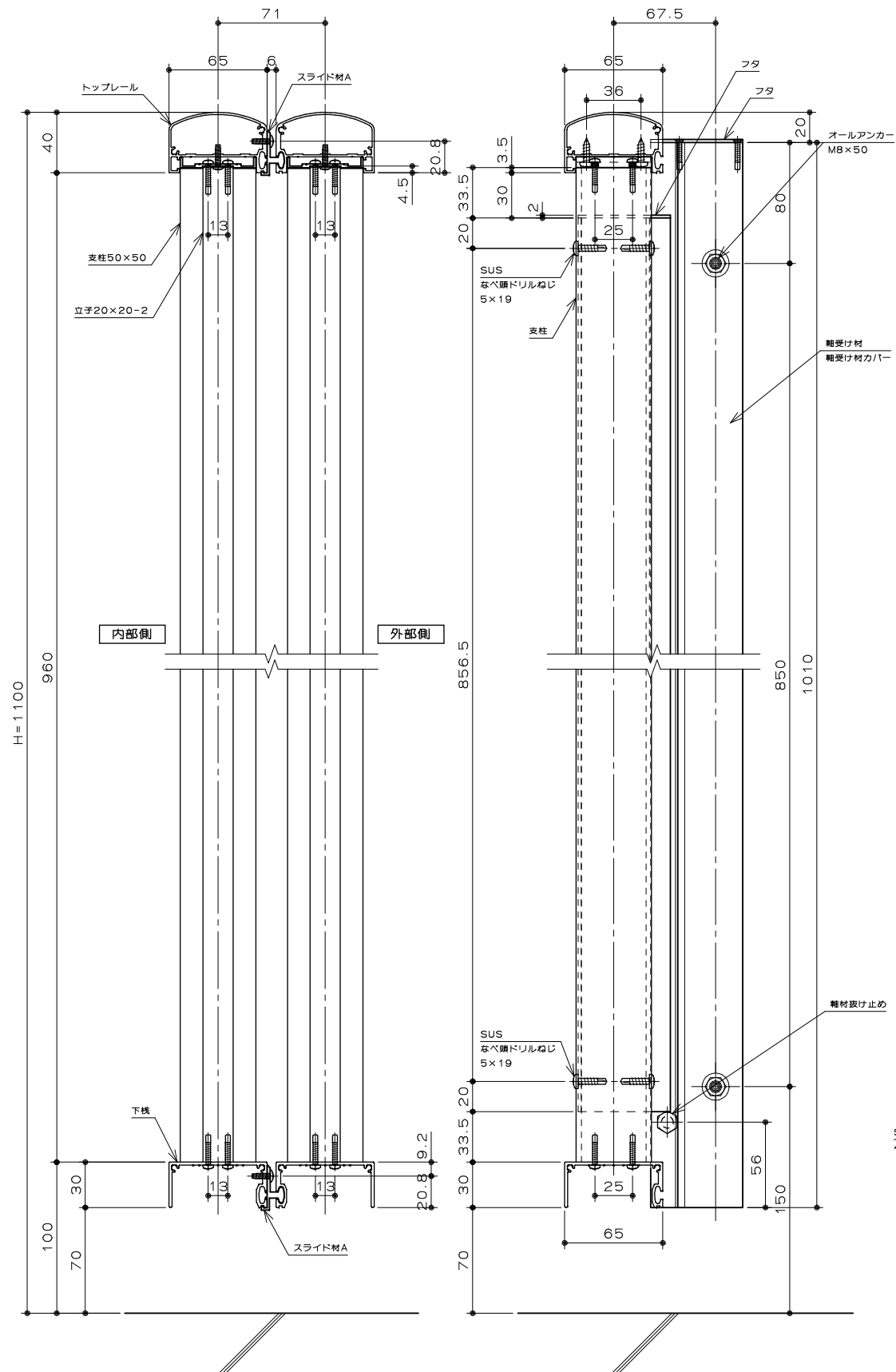
あ断面図 S=1/4
