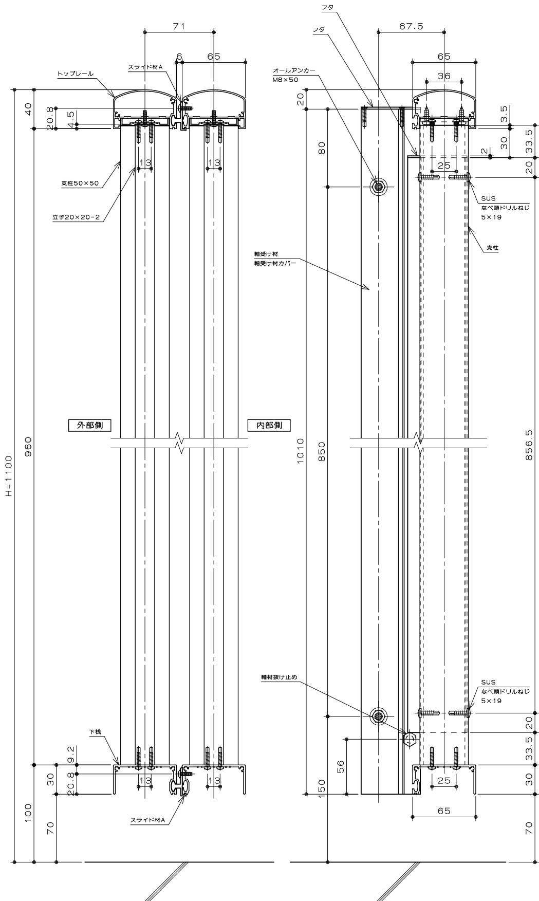
断面図 S = 1/4
