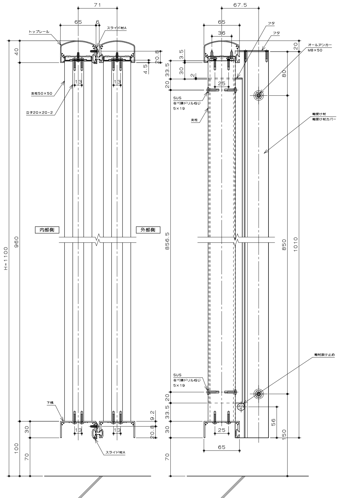
断面図 S = 1/4
