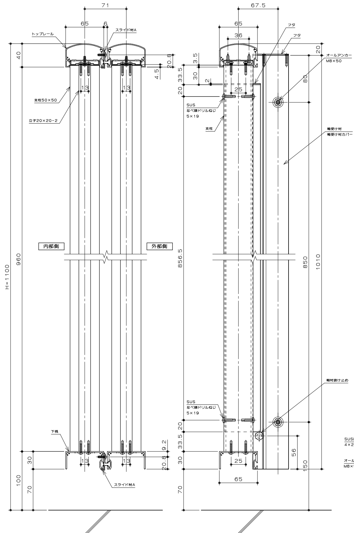
断面図 S = 1/4
