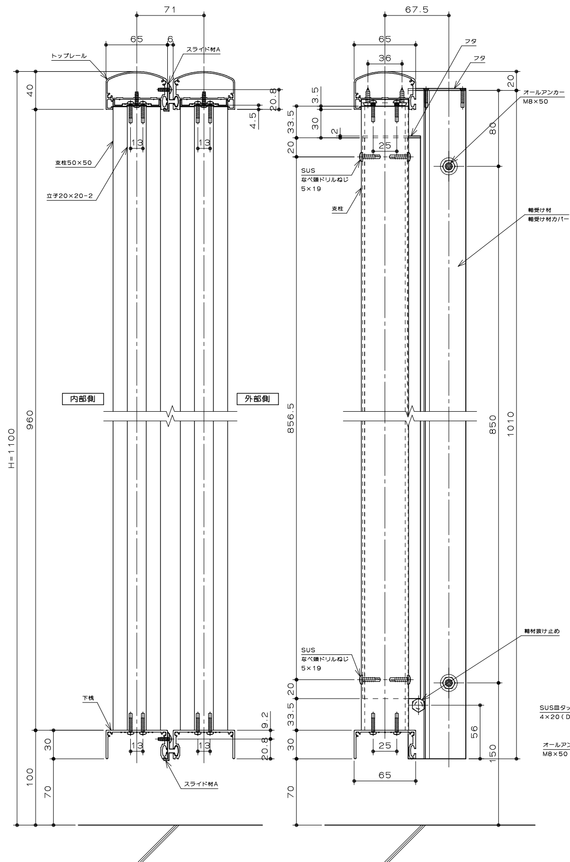
断面図 S = 1/4
