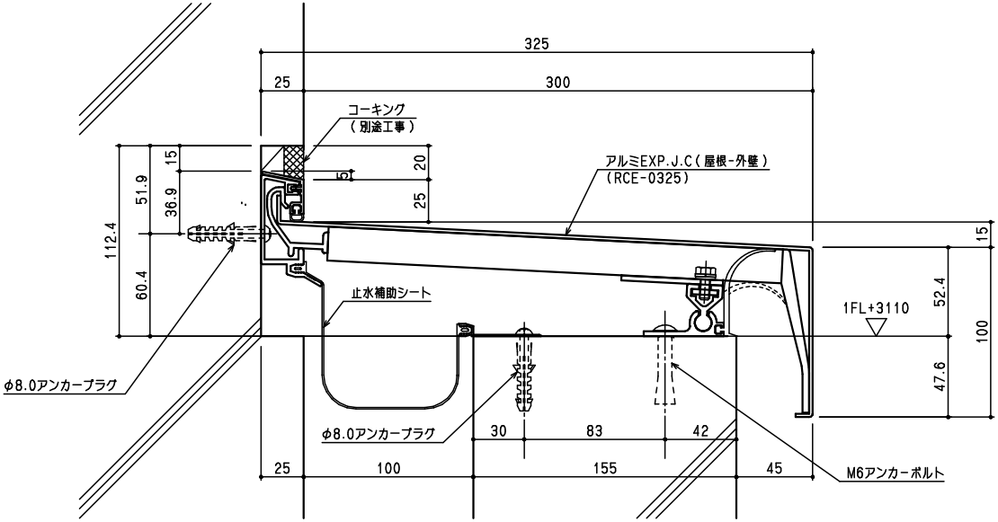
アルミEXP.J.C (屋根-外壁) 断面図 (RCE-0325)
