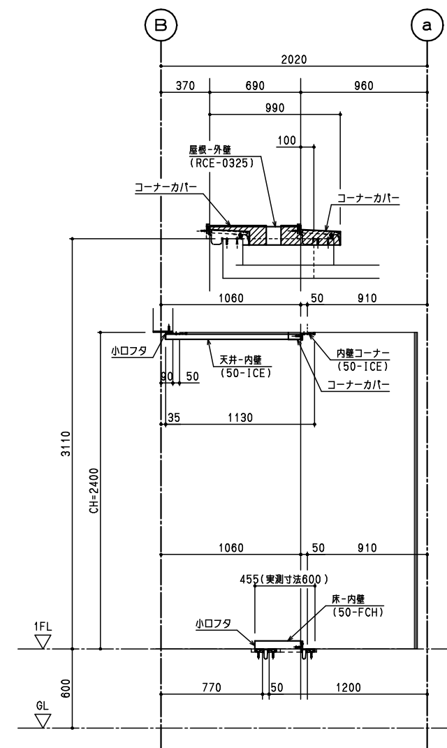
ウ矢視 立面図
