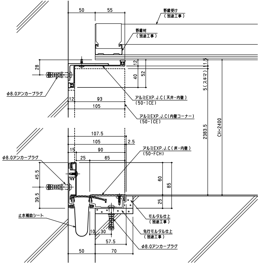
アルミEXP.J.C (天井-内壁) 断面図 (50-ICE) アルミEXP.J.C (床-内壁) 断面図 (50-FCH)
