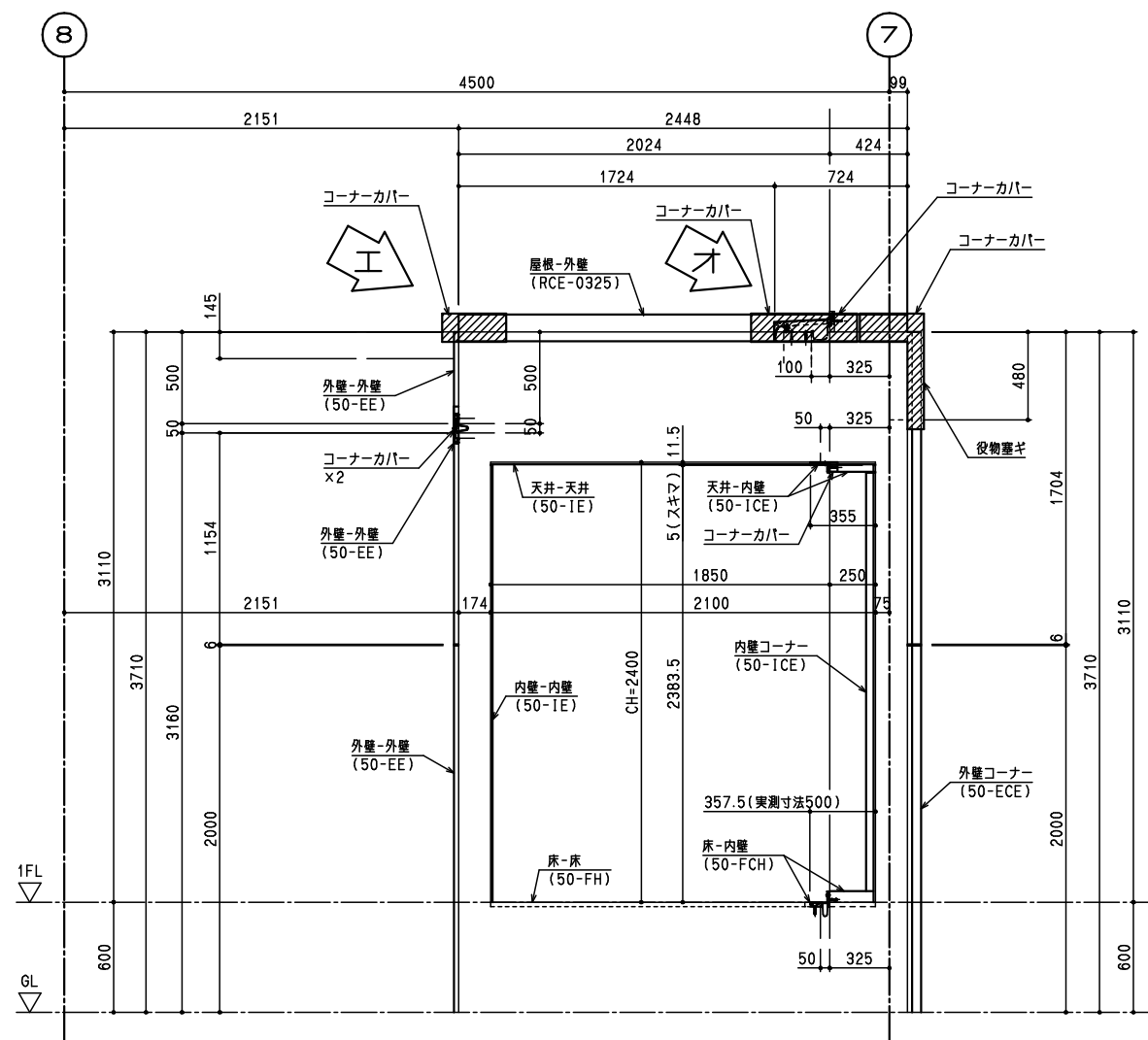
イ矢視 立面図
