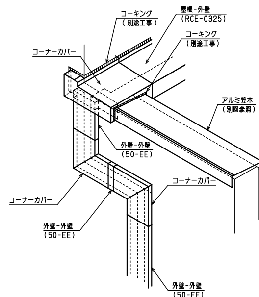
工矢視図
