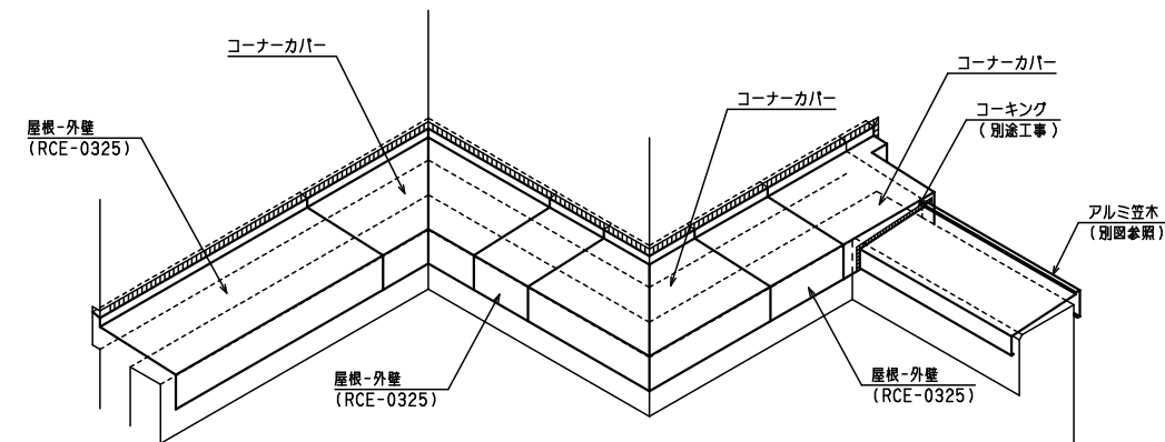
オ矢視図
