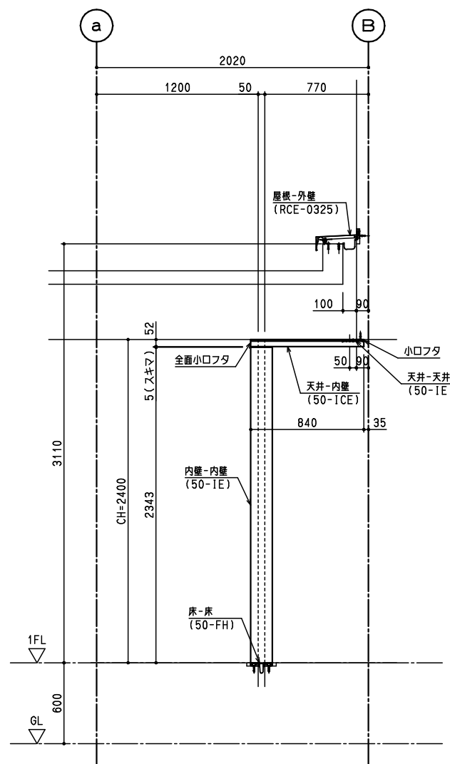
ア矢視 立面図
