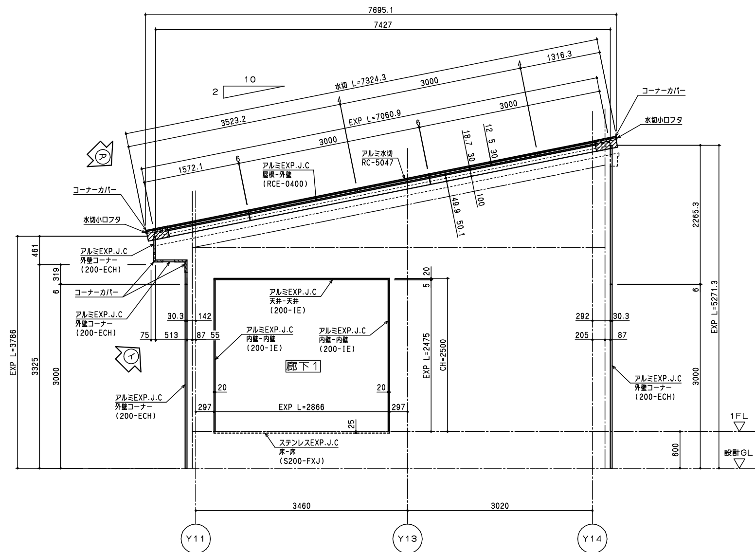
立面図
