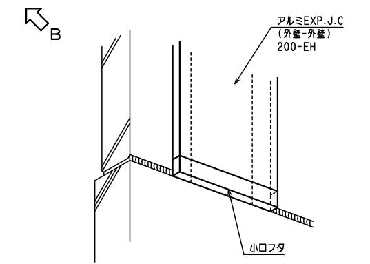
B 矢視図
