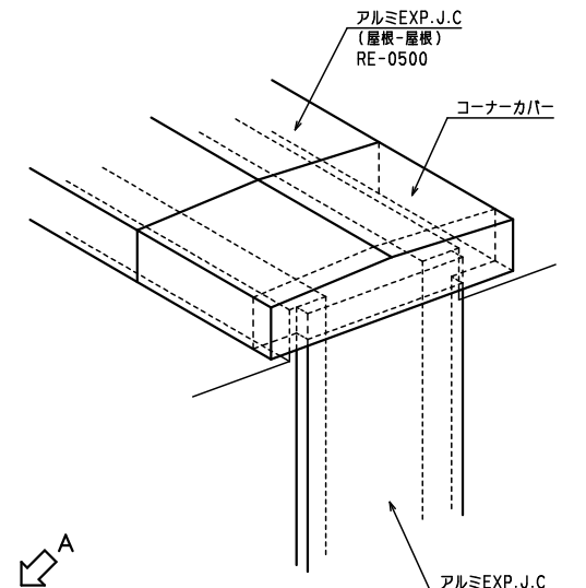
A 矢視図
