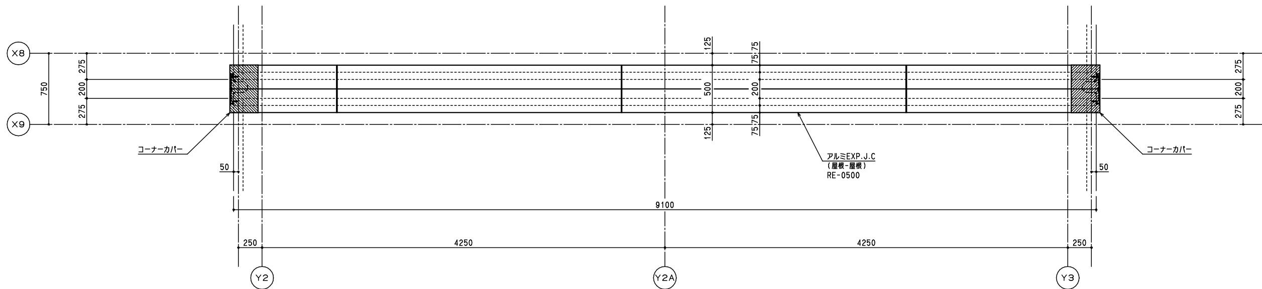
屋根伏図
