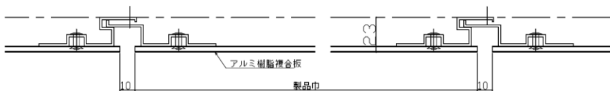
〔製品断面図〕
