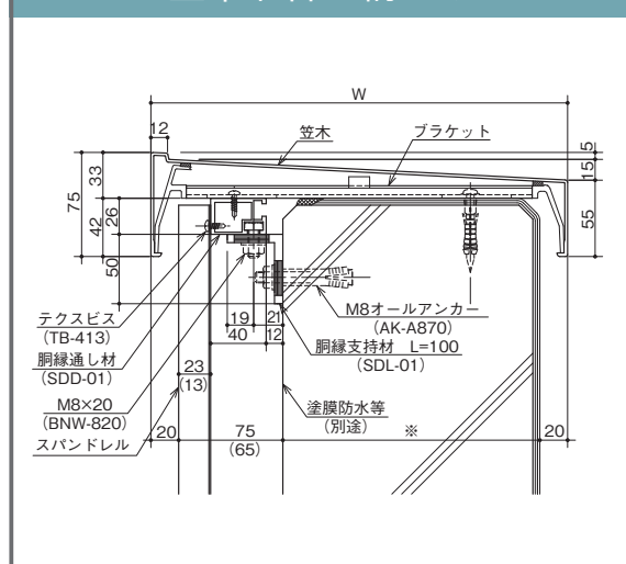
笠木取合い納まり
