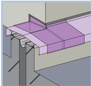
3 屋根と屋根（出隅） 屋根と外壁
