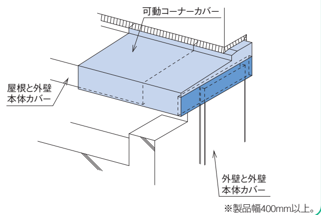
可動タイプ [屋根と外壁：外壁と外壁]
