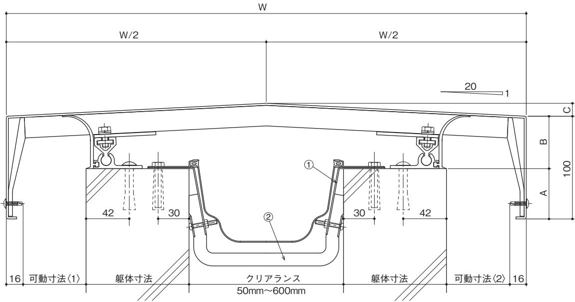
①耐火帯押えプレート ②耐火帯
