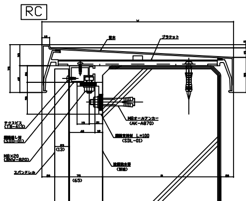
上部参考納まり図
