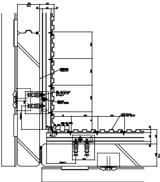
入隅部横断面図 (ALC壁)
