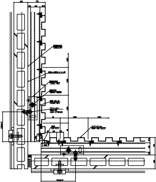
入隅部横断面図 (浮き出し型 壁セメント系)
