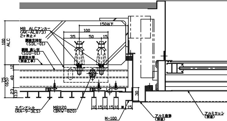
サッシ取合横断面図 (ALC)
