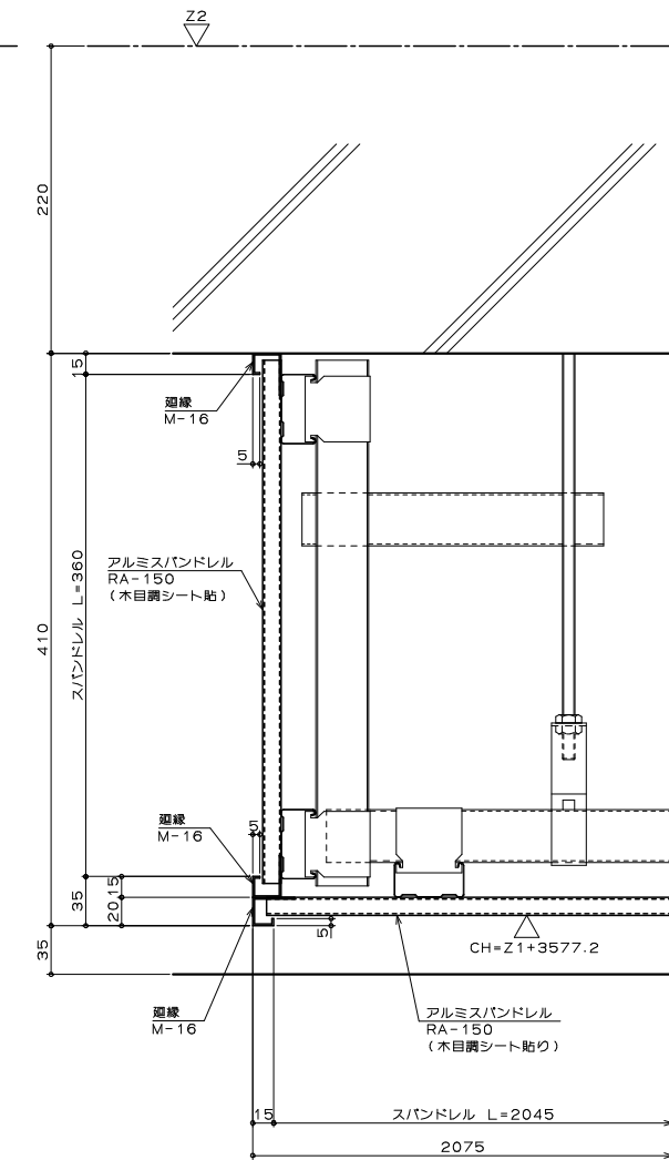
縦断面図
