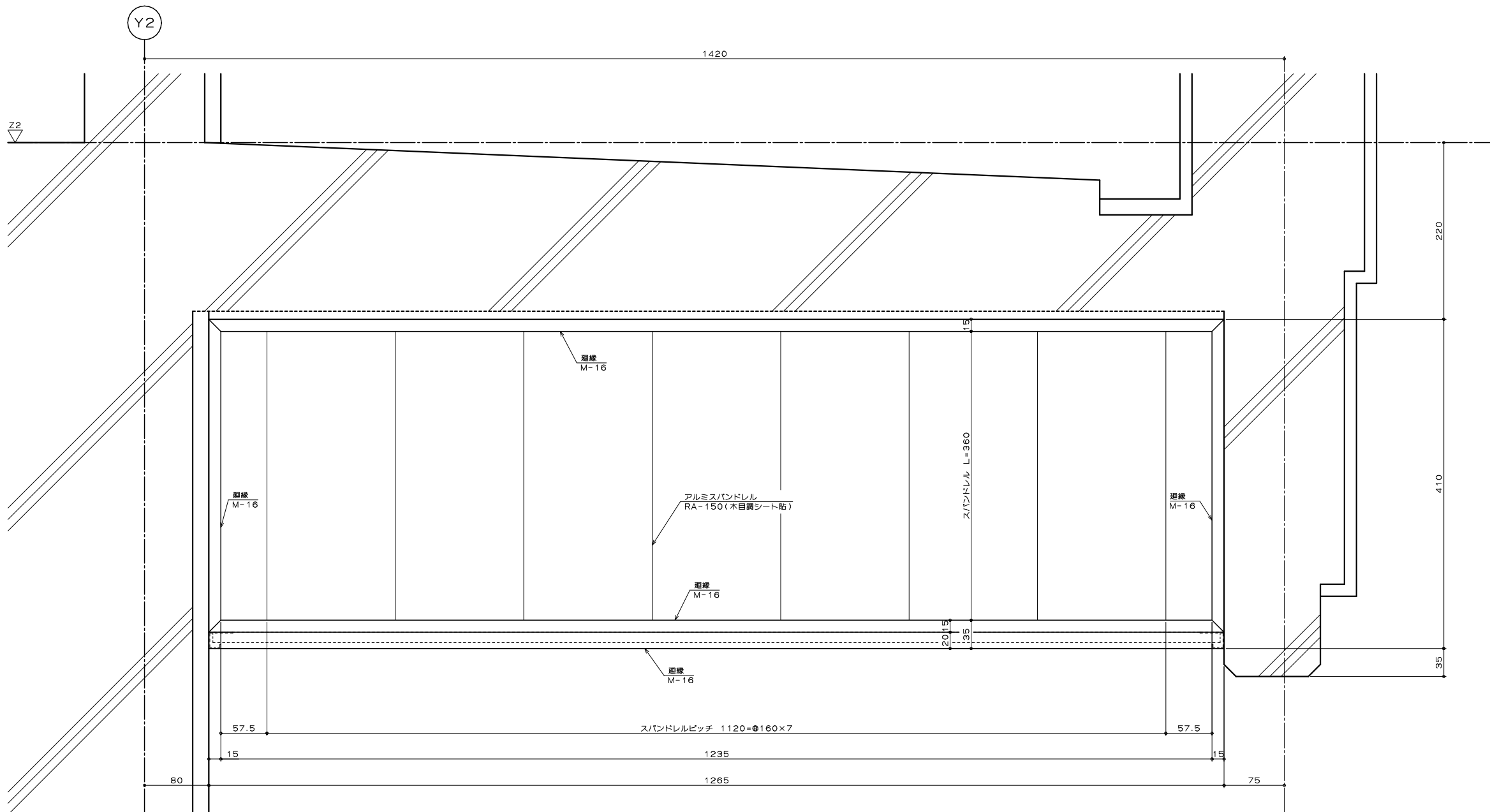
あ矢視立面図
