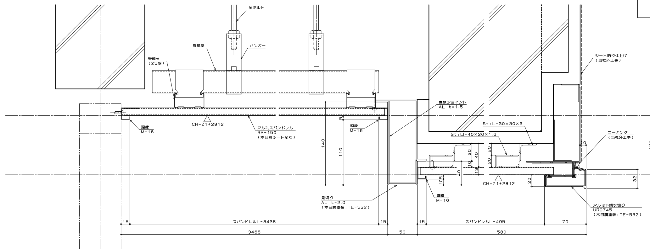
B断面詳細図
