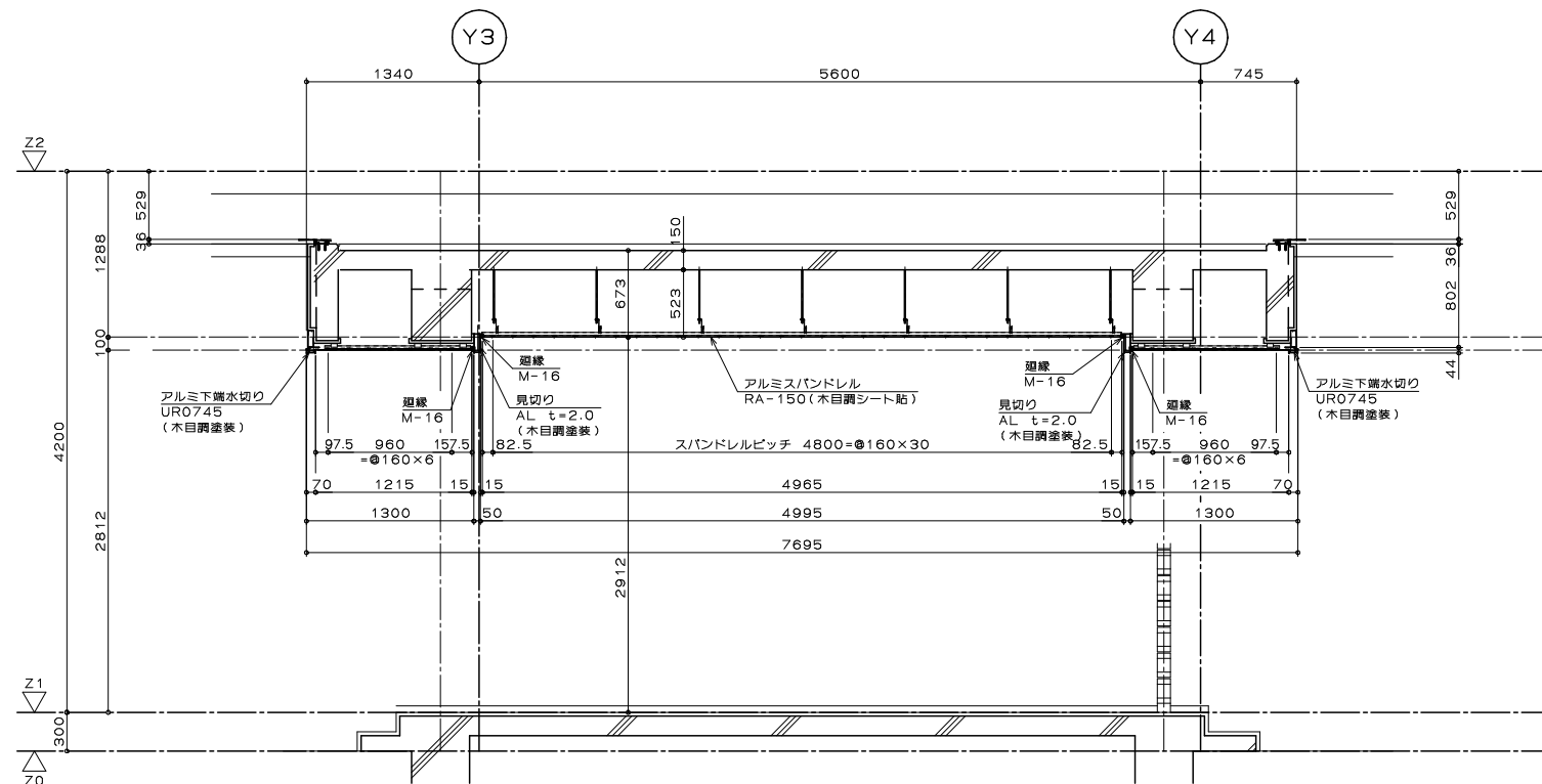
A断面図
