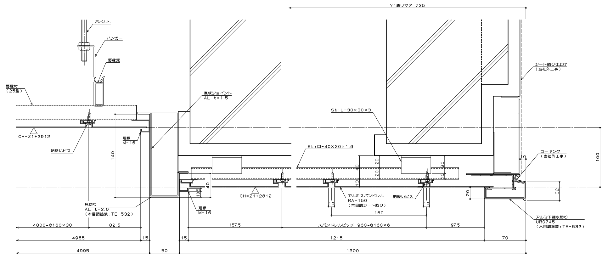
A断面詳細図
