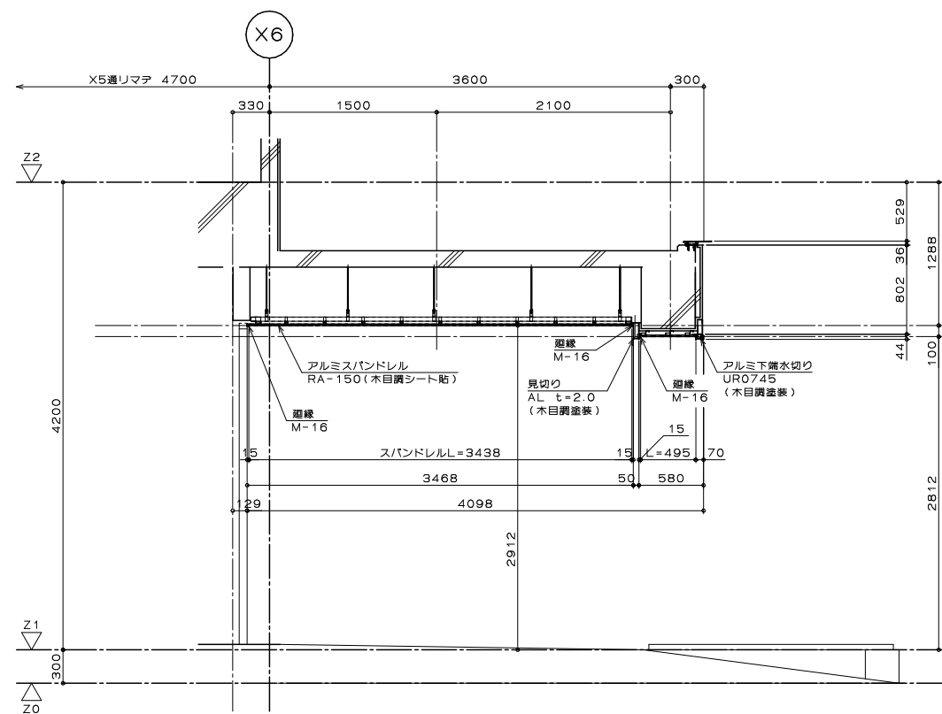
B断面図
