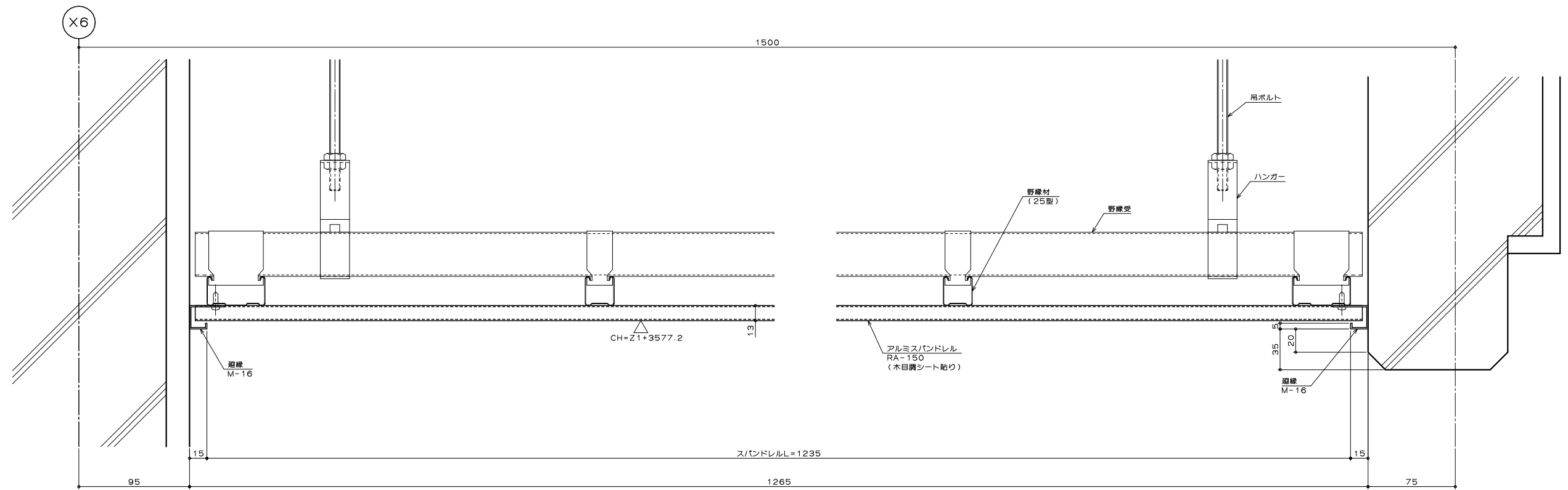
C断面詳細図
