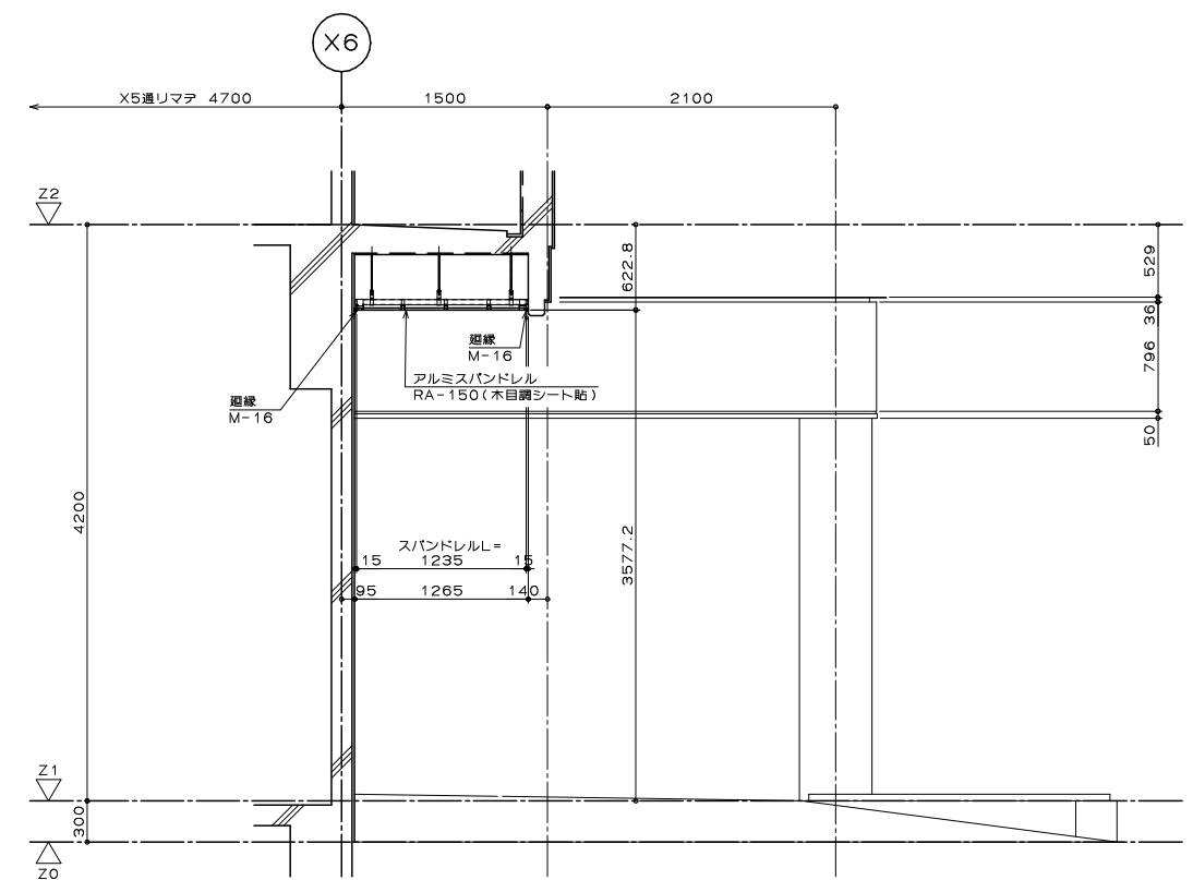
C断面図
