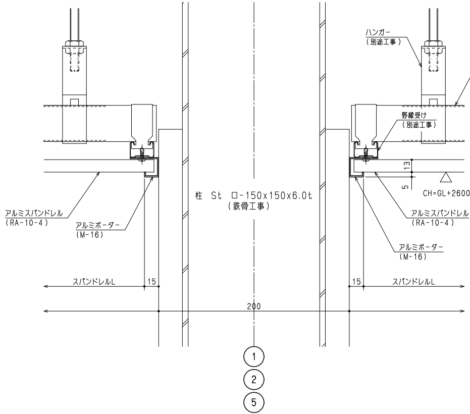
B 断面
