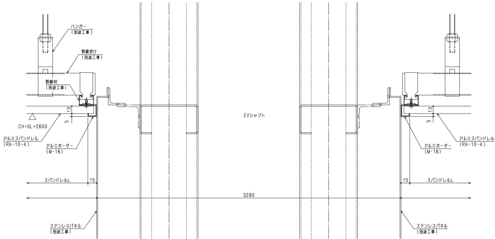
C 断面
