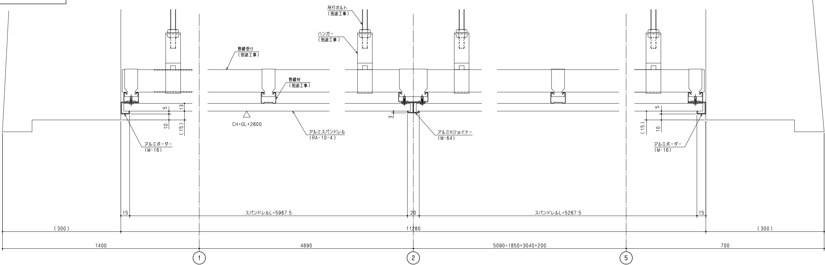
A~A' 断面
