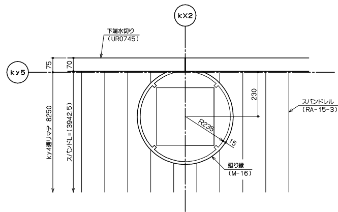
柱廻り詳細図
