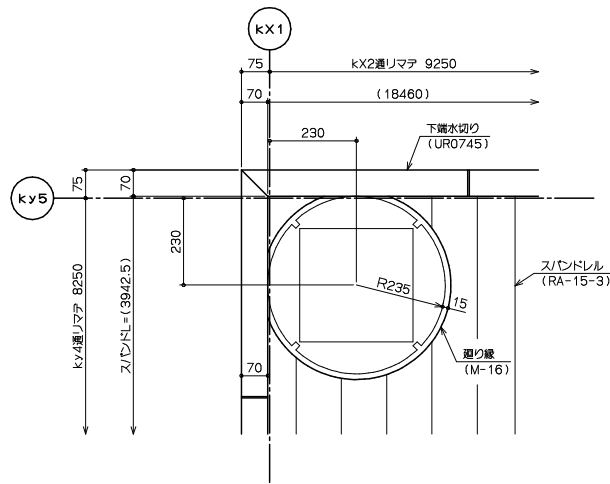
柱廻り詳細図 ※kX3通り側対称
