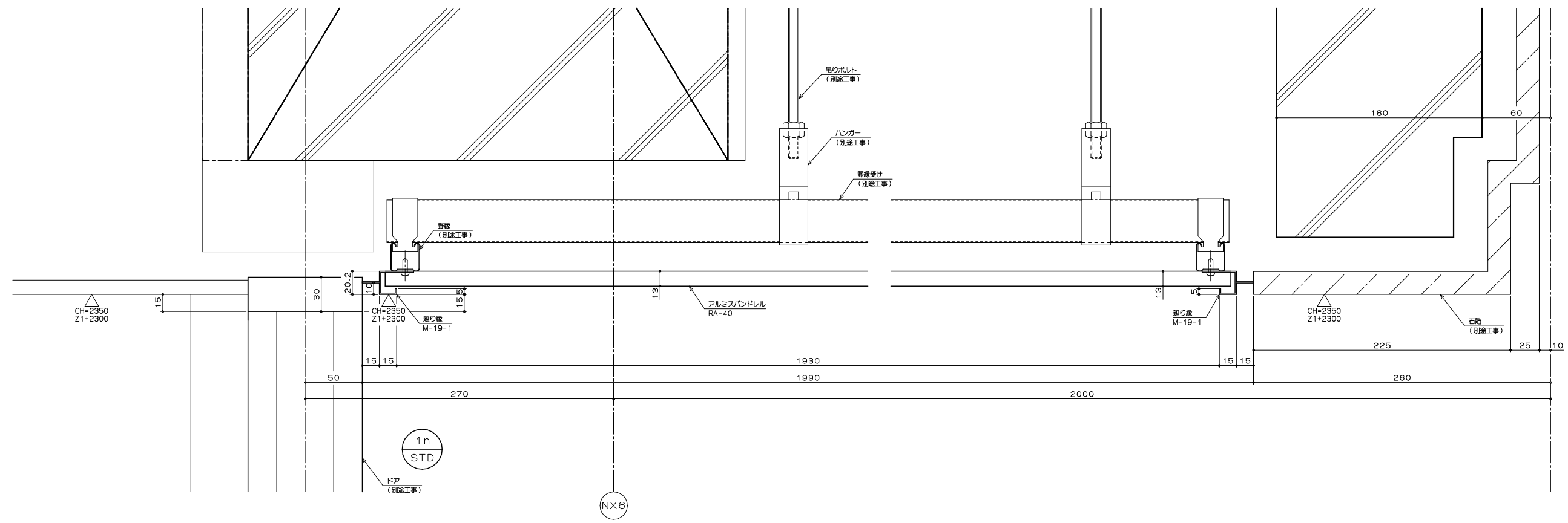
A断面詳細図
