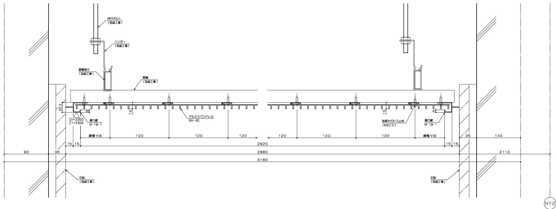
C断面詳細図
