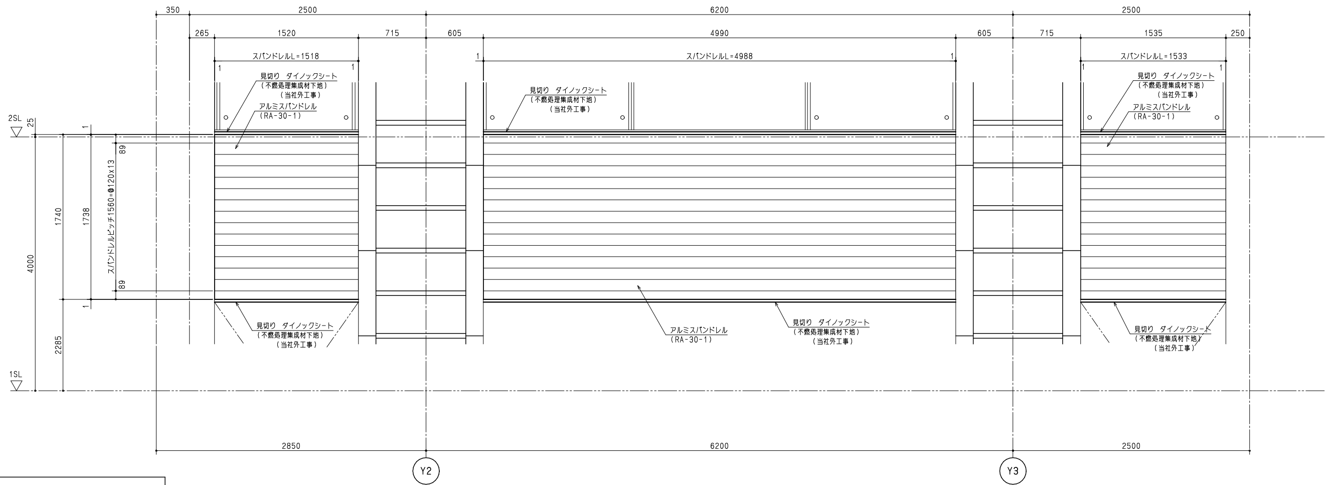
立面矢视图
