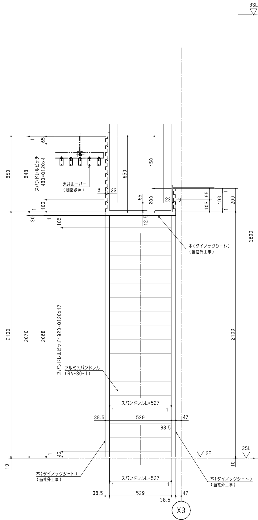
立面矢视图
