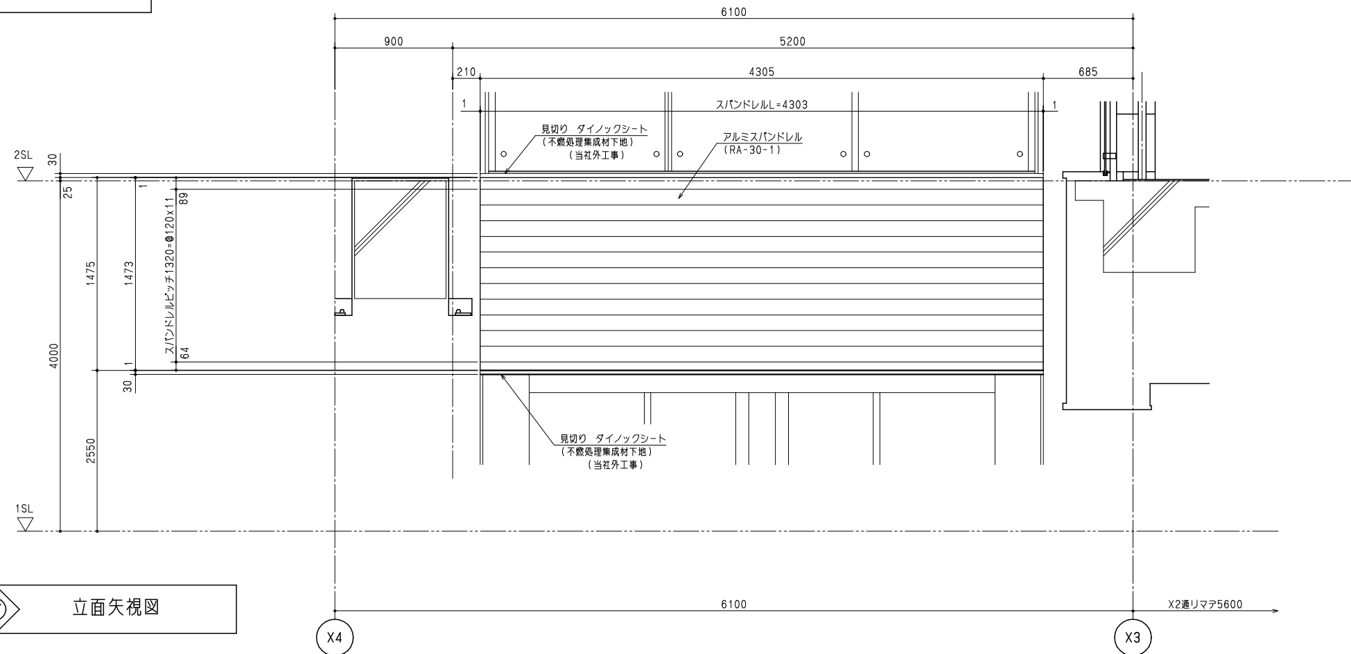
立面矢视图
