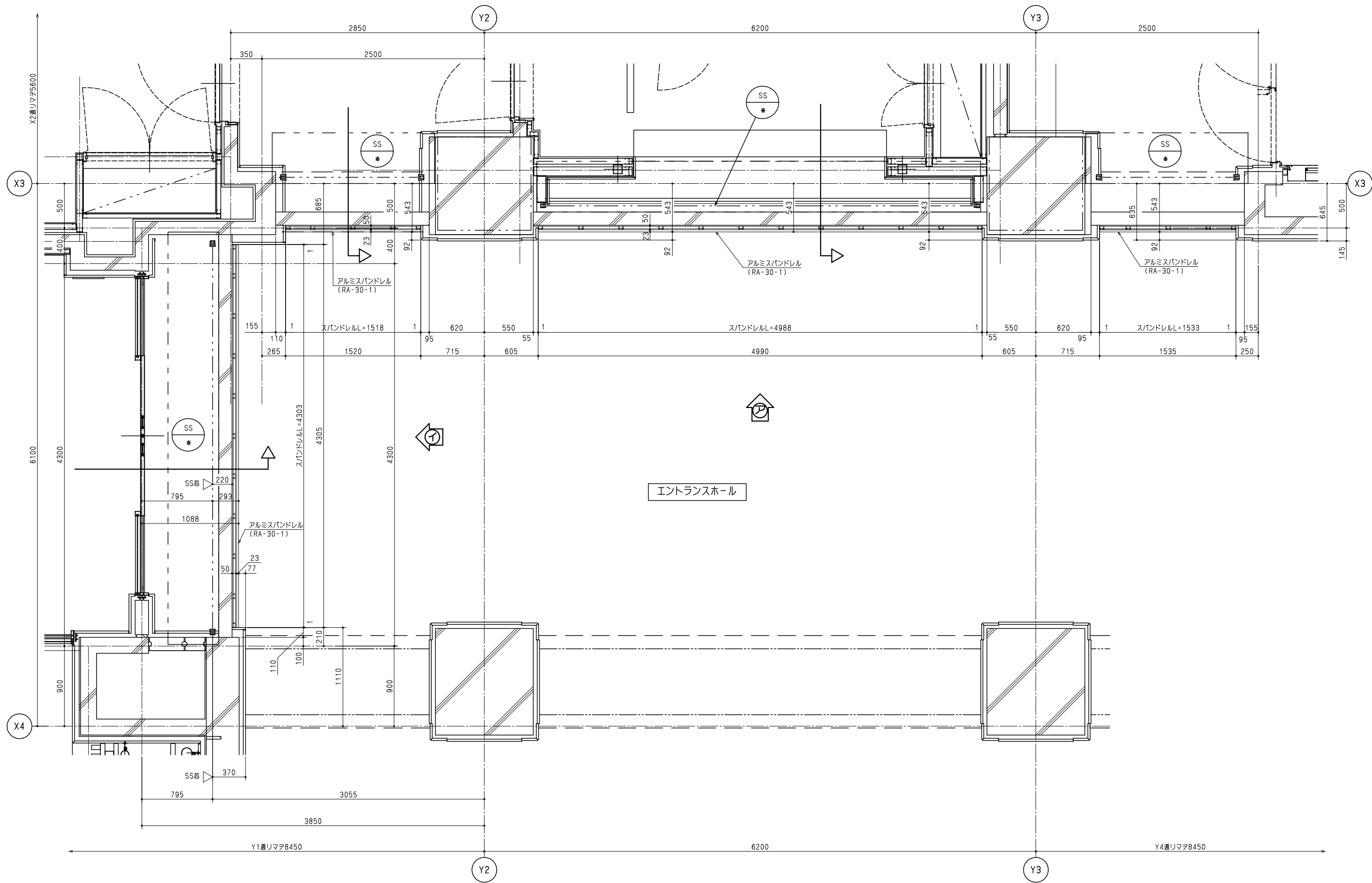
エントランスホール平面図
