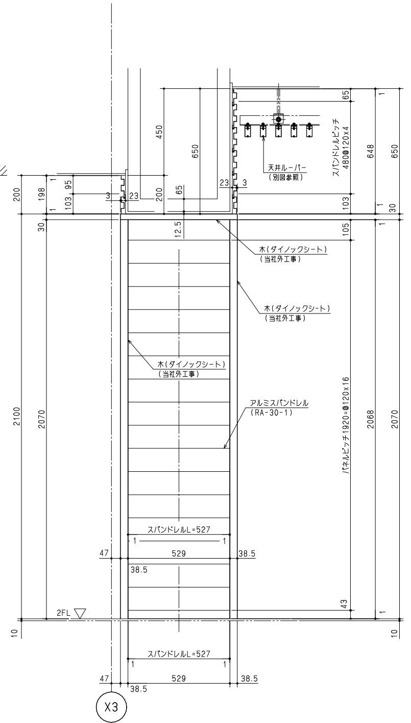
立面矢视图
