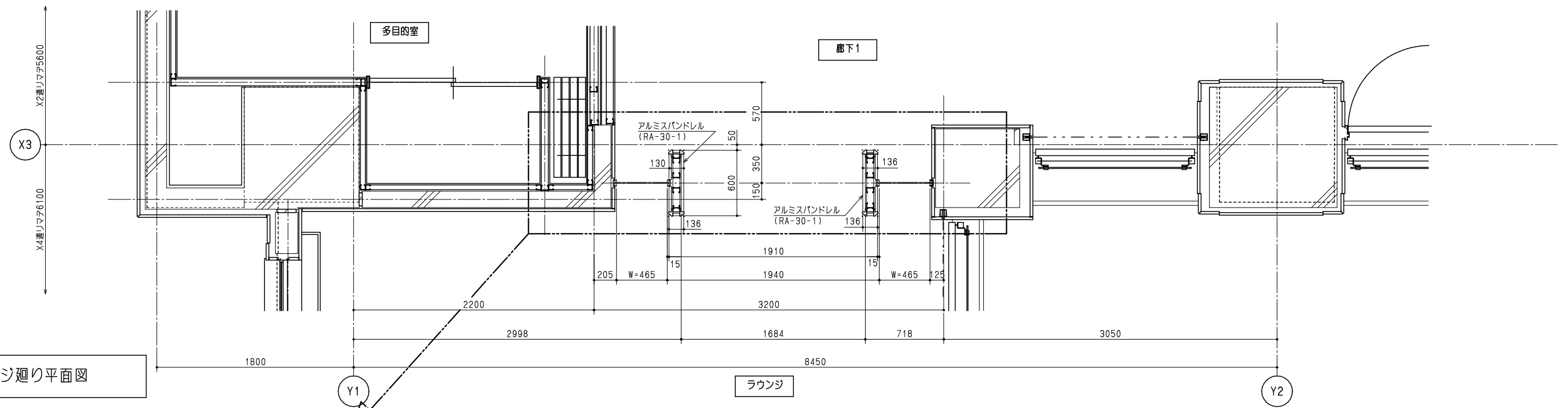
拡大図 S=1/10
