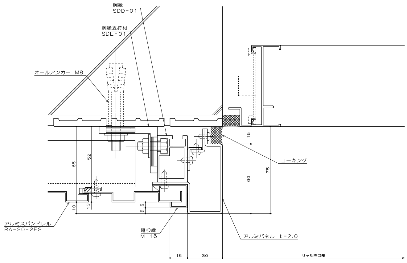
サッシ開口部 横断面図
