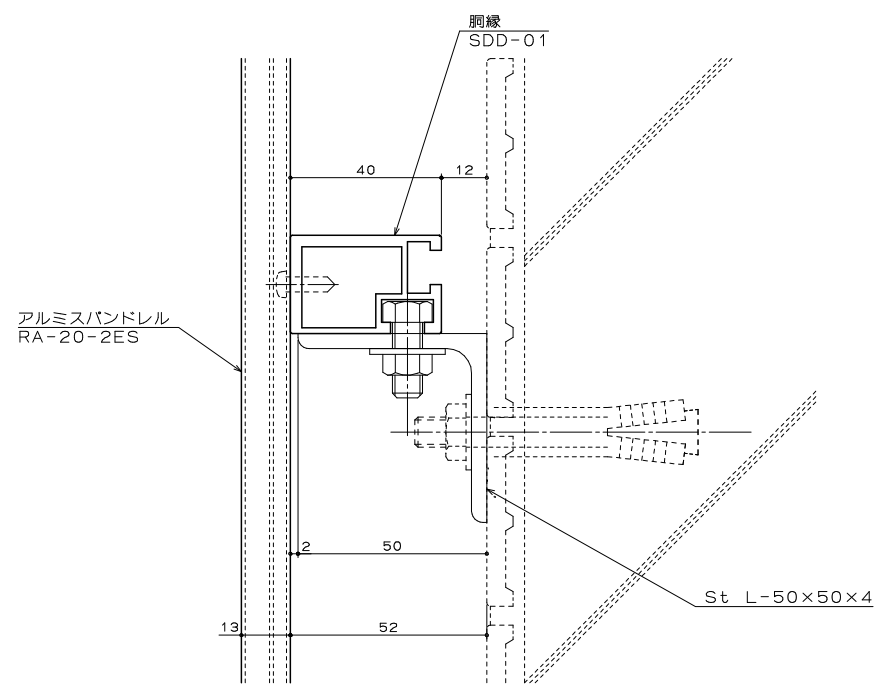
サッシ開口部 縦断面図
