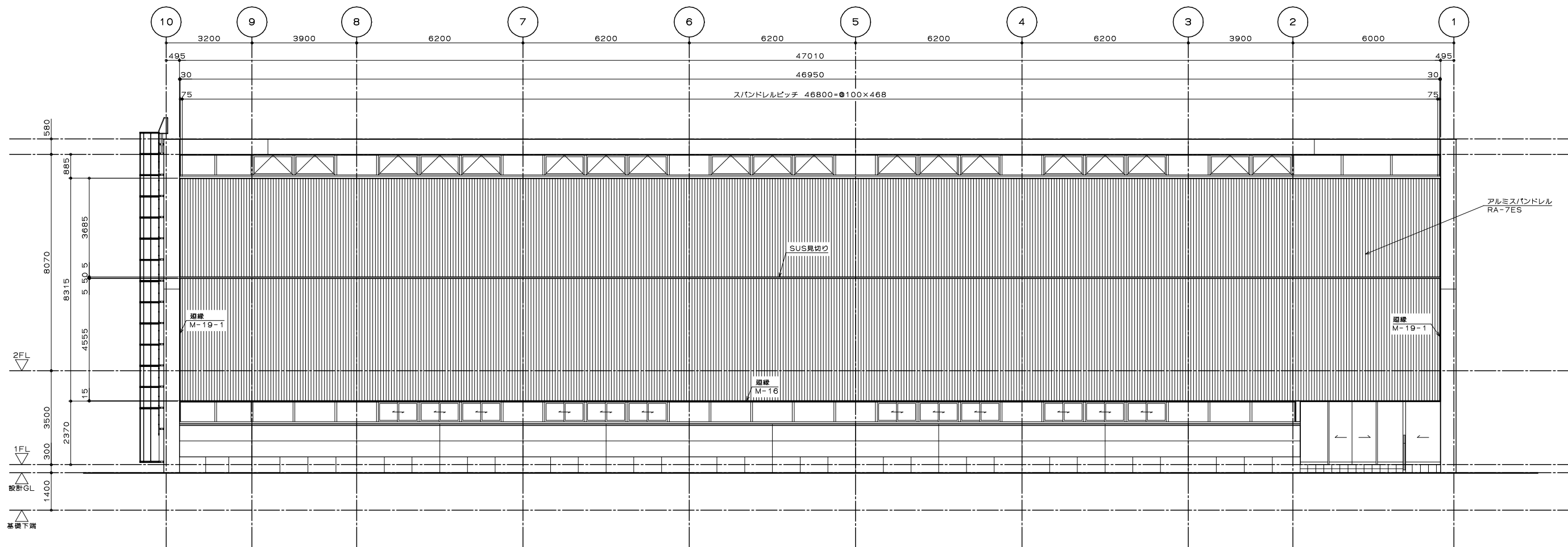
立面図
