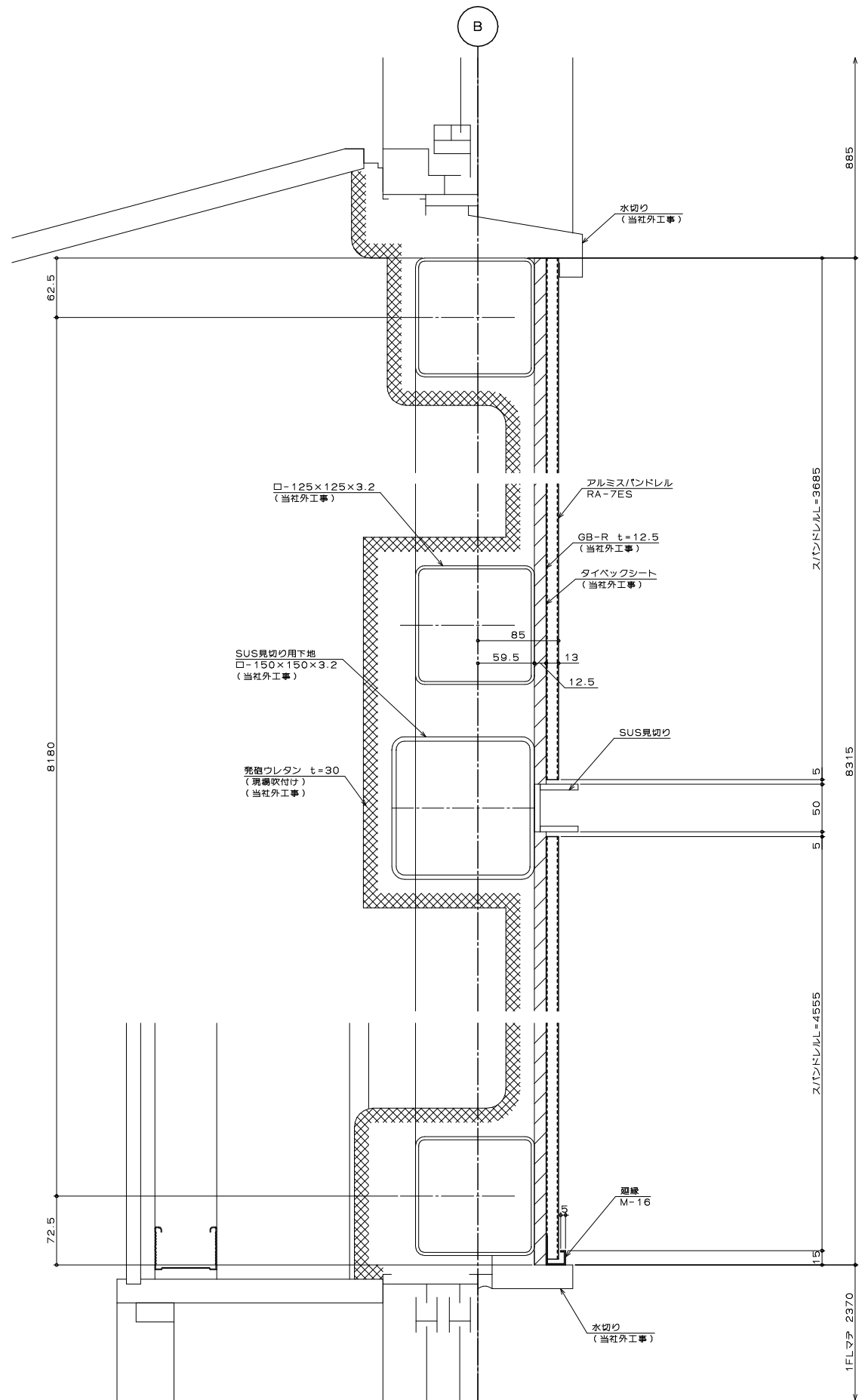
断面詳細図
