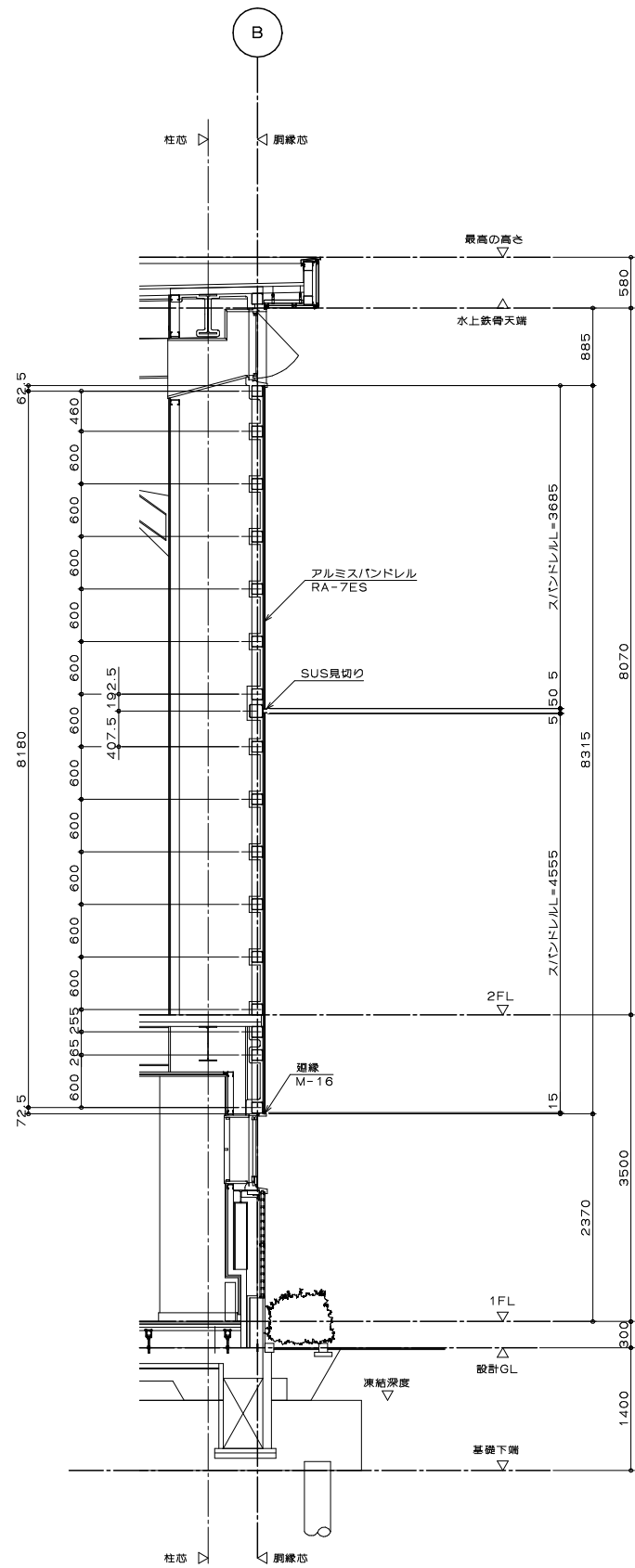
断面図
