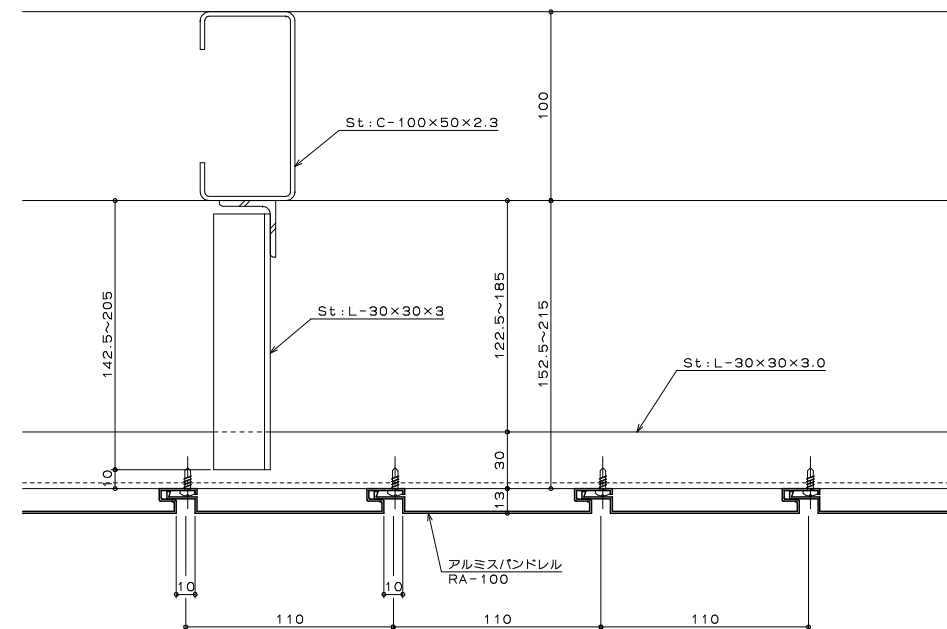
基本平面詳細図
