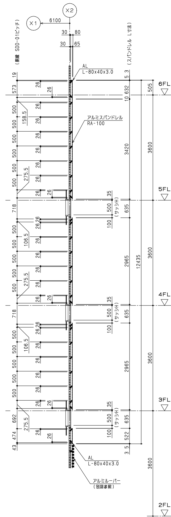
ウ-ウ 断面図
