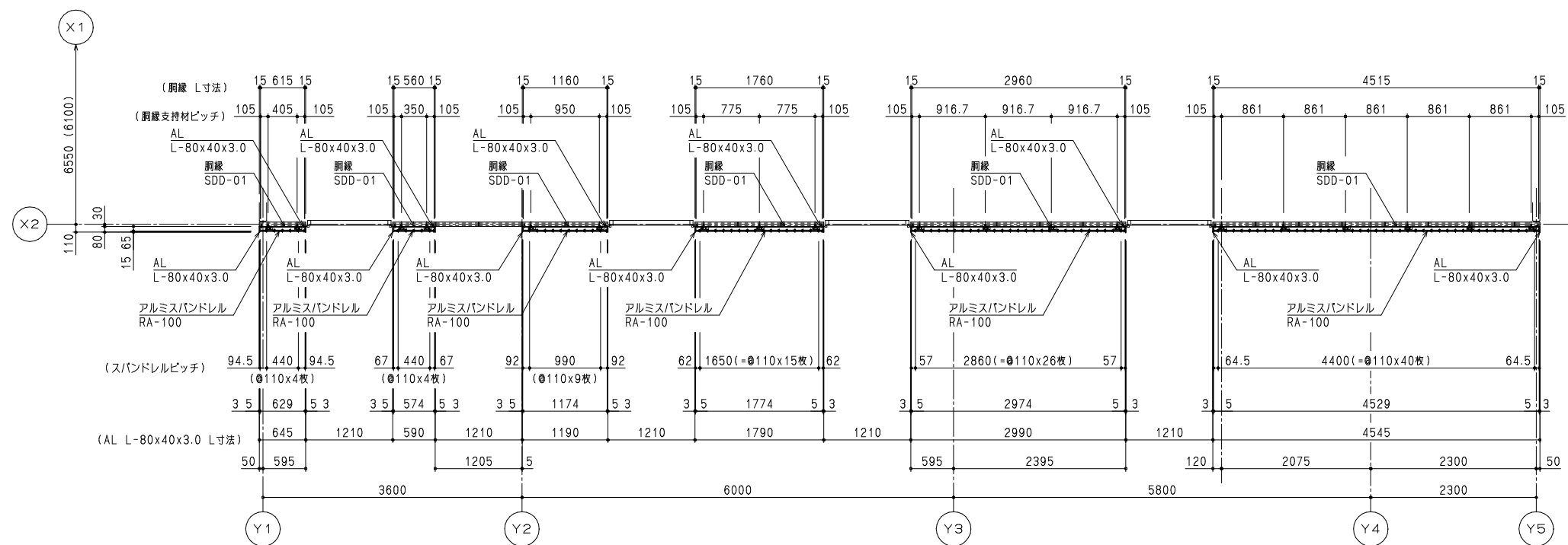
A-A 断面図
