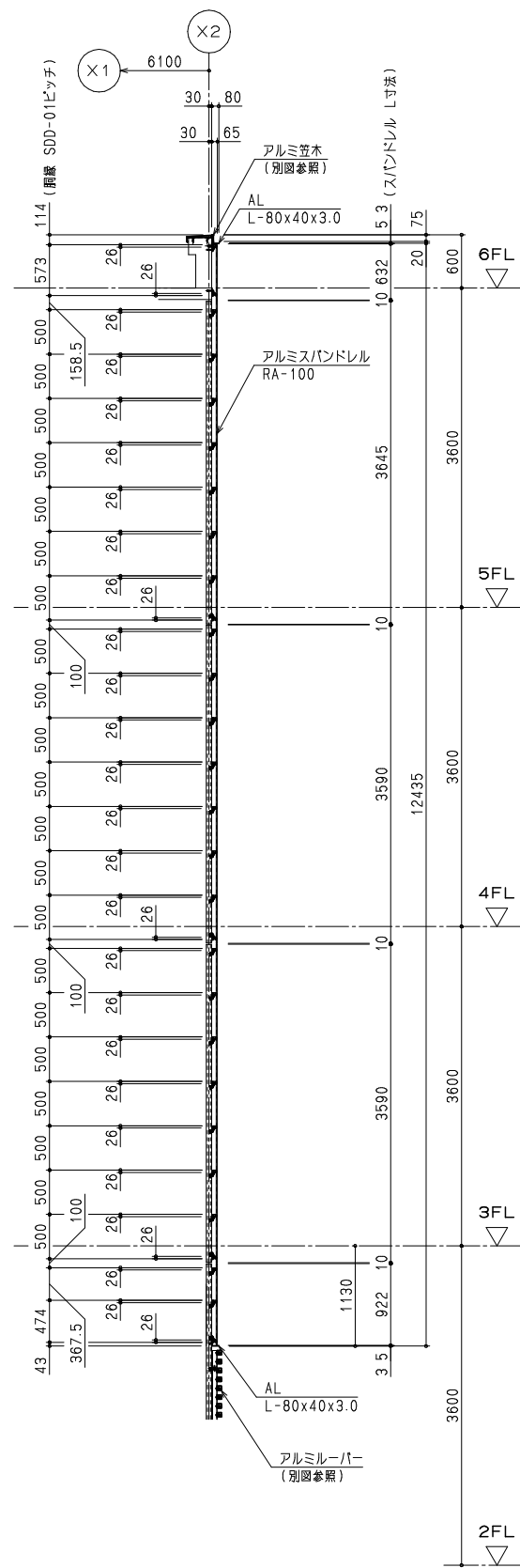
イ-イ 断面図
