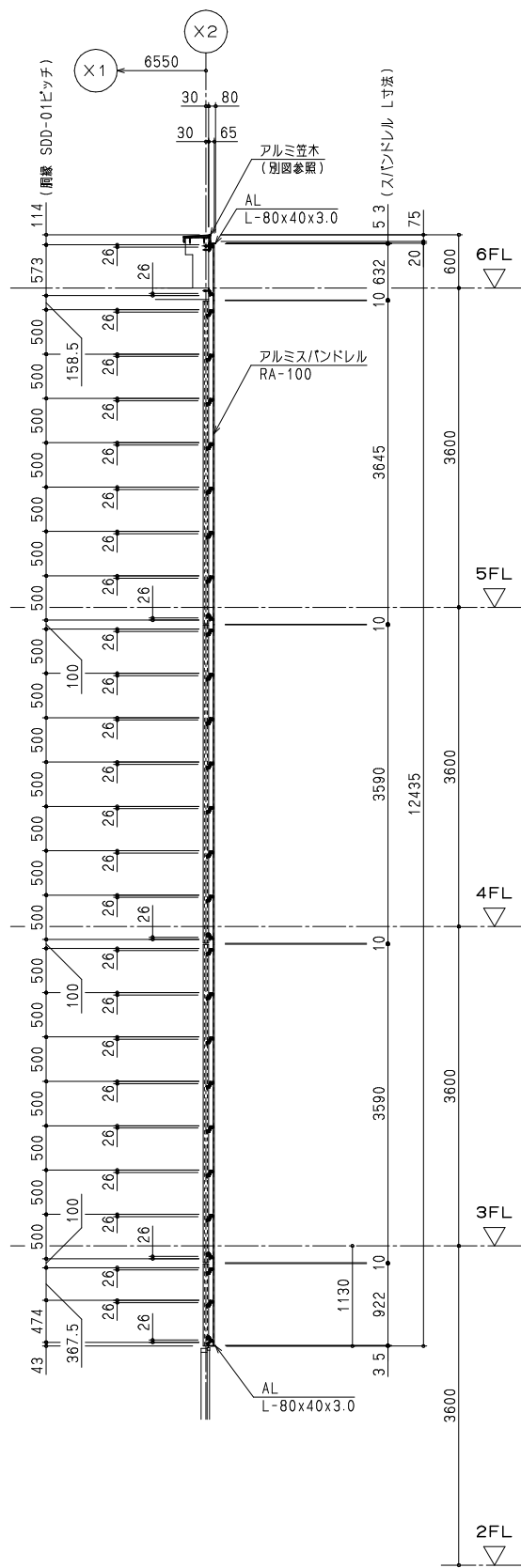
ア-ア 断面図
