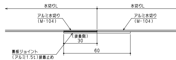
アルミ水切り (M104) ジョイント部
