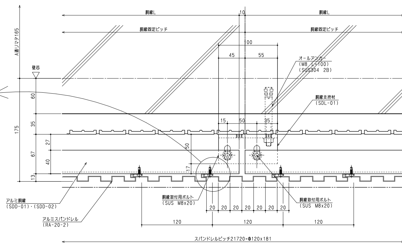
う部（胴縁目地部） 詳細図
