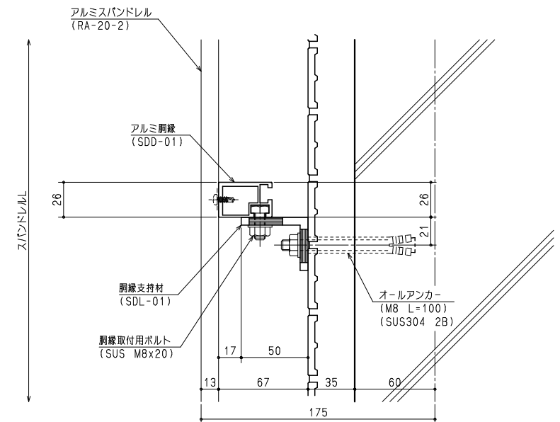
こ部 (一般中間部) 詳細図
