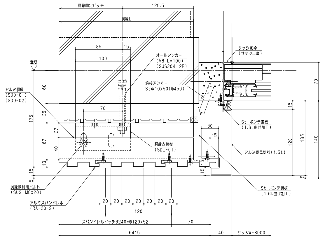
え部 詳細図
