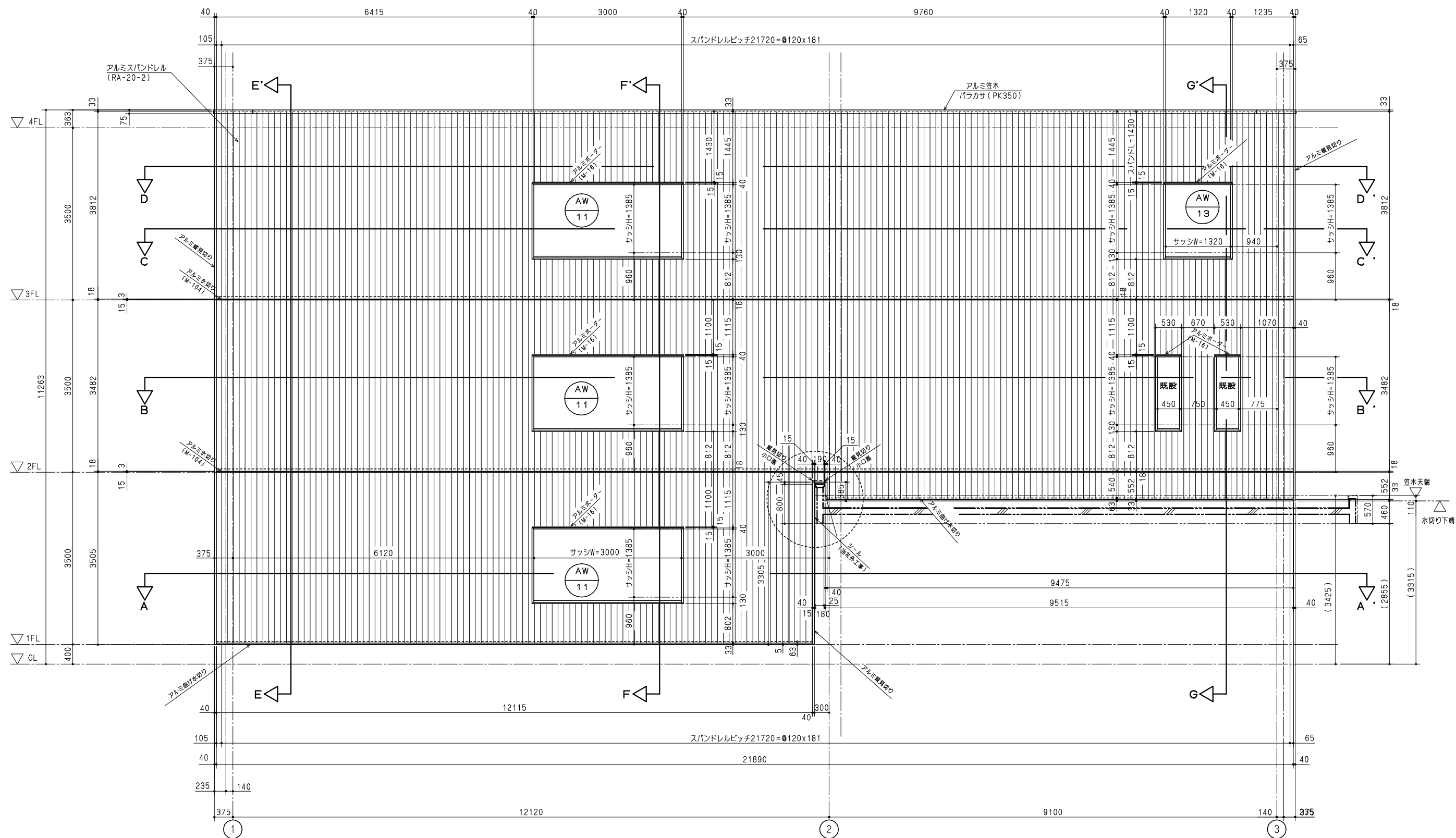
A通り 立面図
