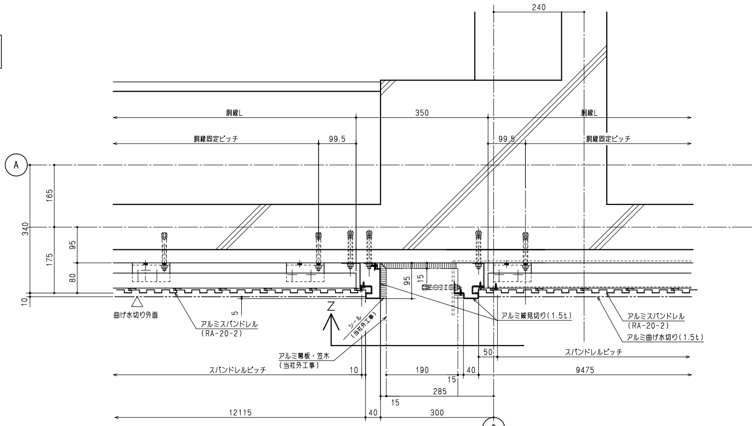
アルミ底部 縦見切り〜曲げ水切り取合い 平面詳細図
