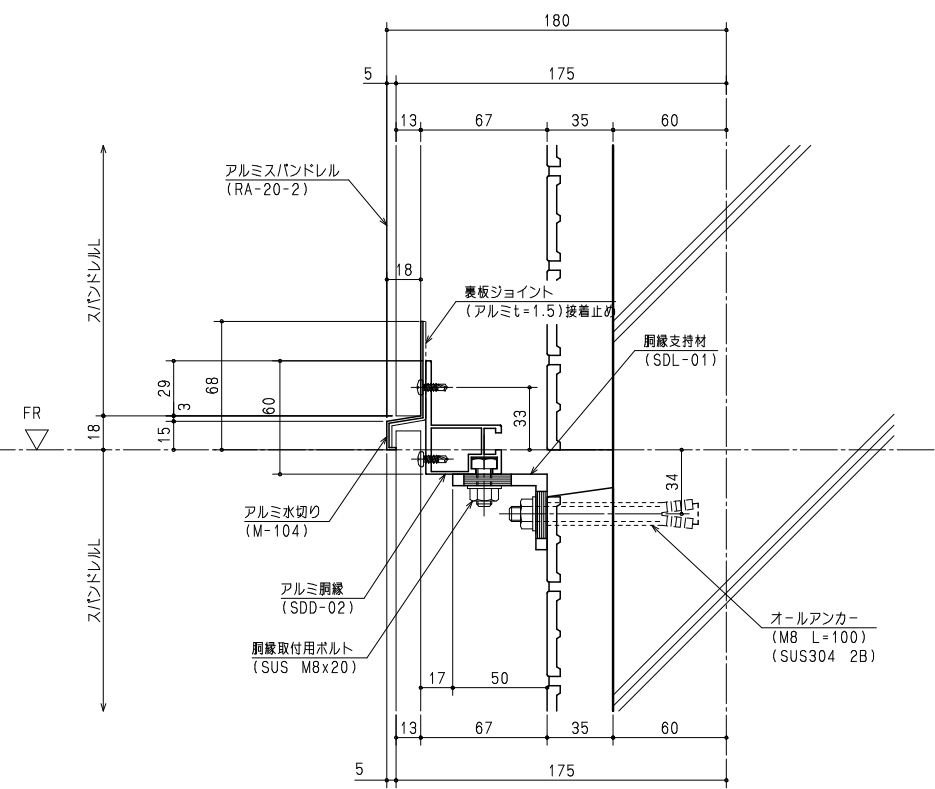
さ部 (スバンドレル目地部) 詳細図
