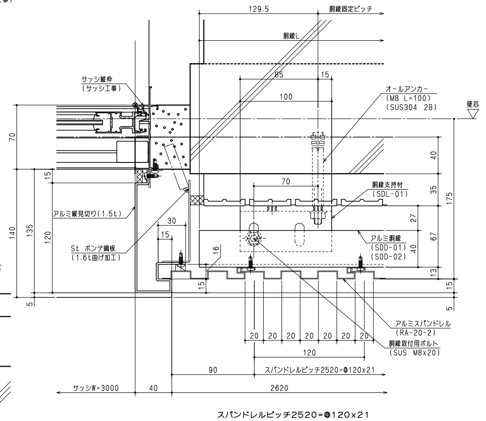
お部 詳細図
