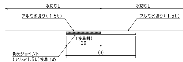
アルミ水切り (曲げ材) ジョイント部
