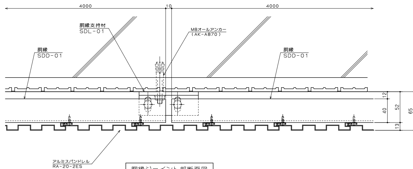
胴縁ジョイント部断面図
