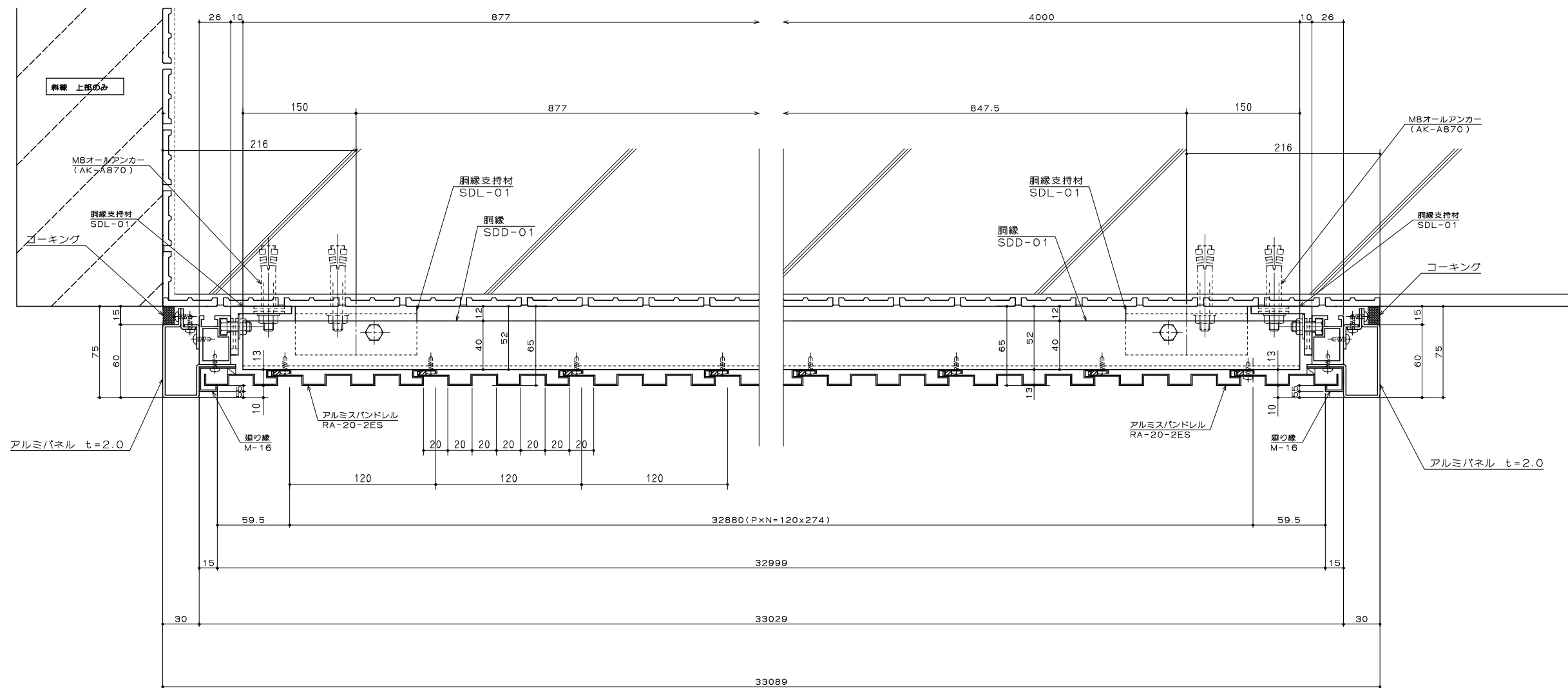
アルミスバンドレス横断面図 (北面)
