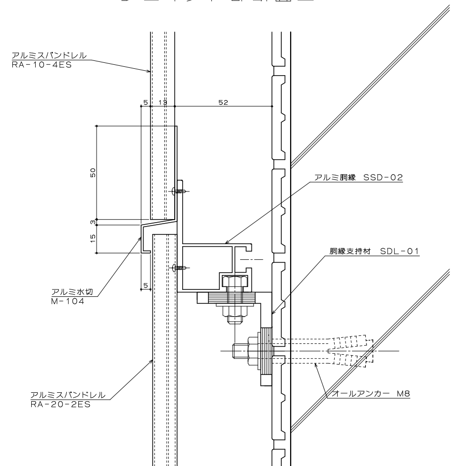
ジョイント部断面図
