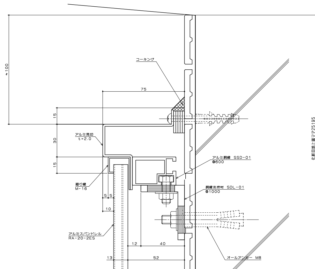
上部断面図
