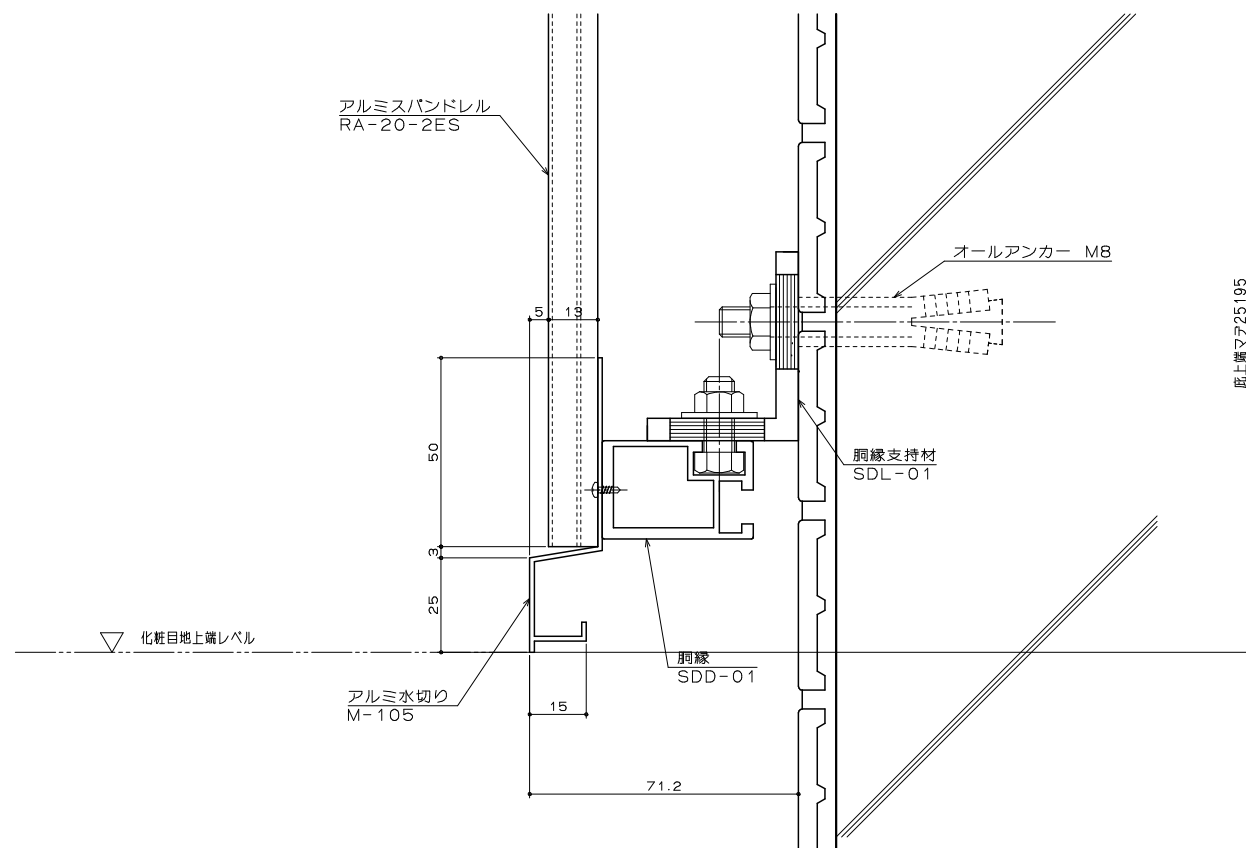
下部断面図
