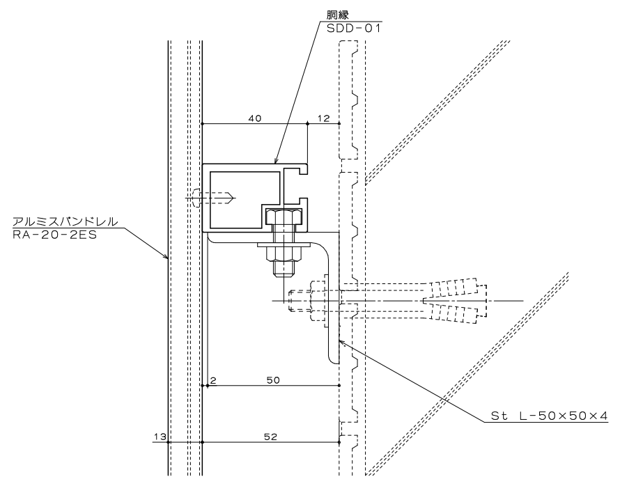
サッシ開口部 縦断面図
