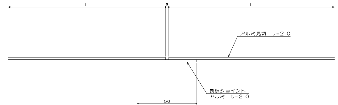
アルミ見切 ジョイント断面図
