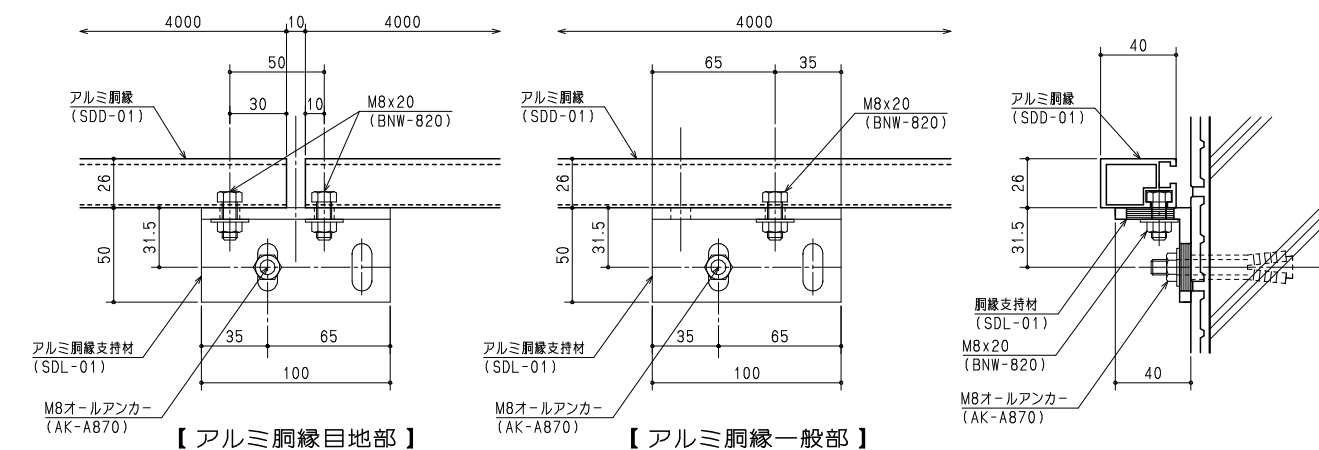
胴縁取付部断面図
