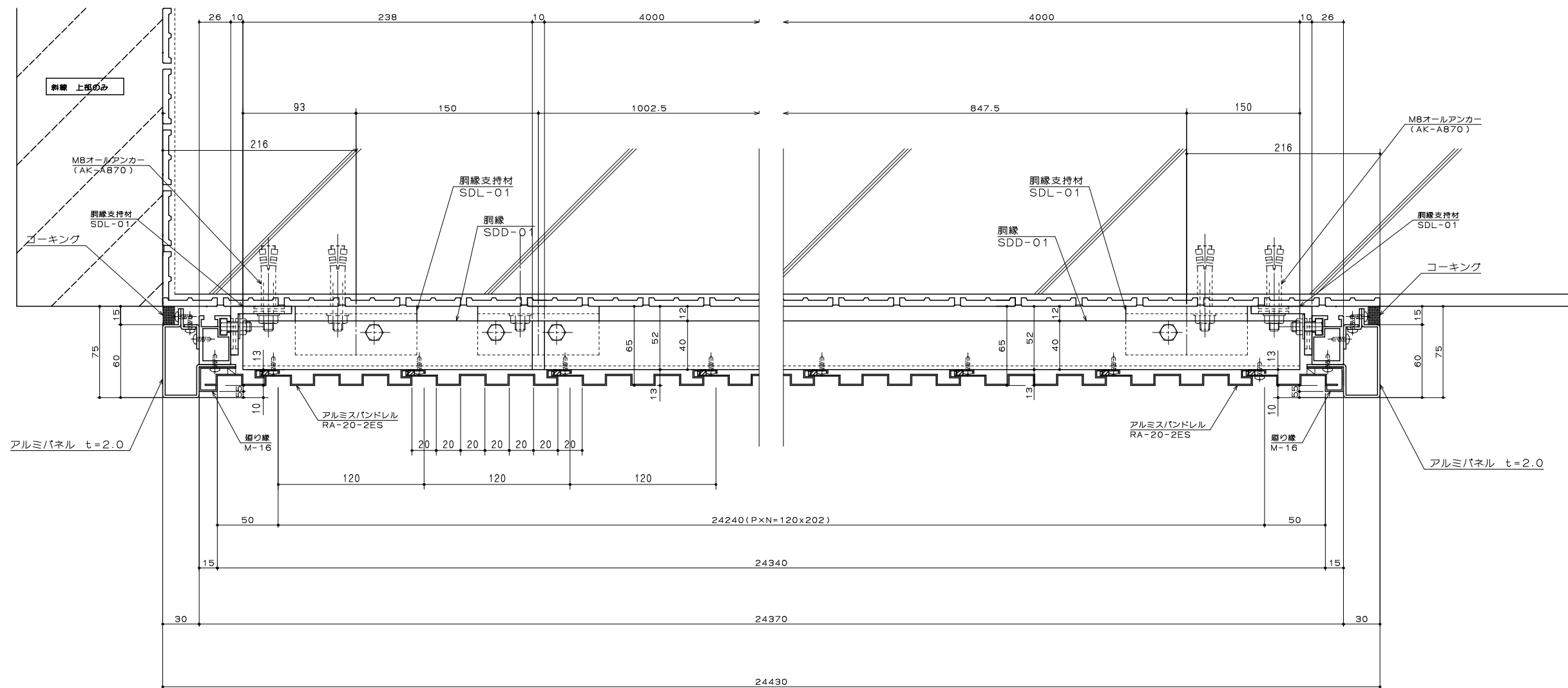
アルミスバンドレス横断面図 ( 南面 )
