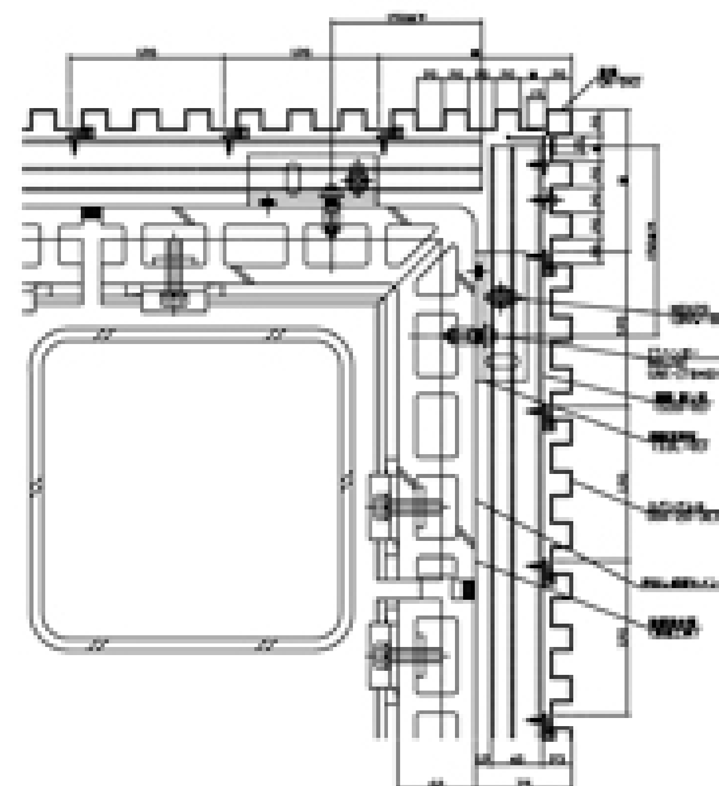
出隅部補強図 (壁筋と床筋の交点に注意)
