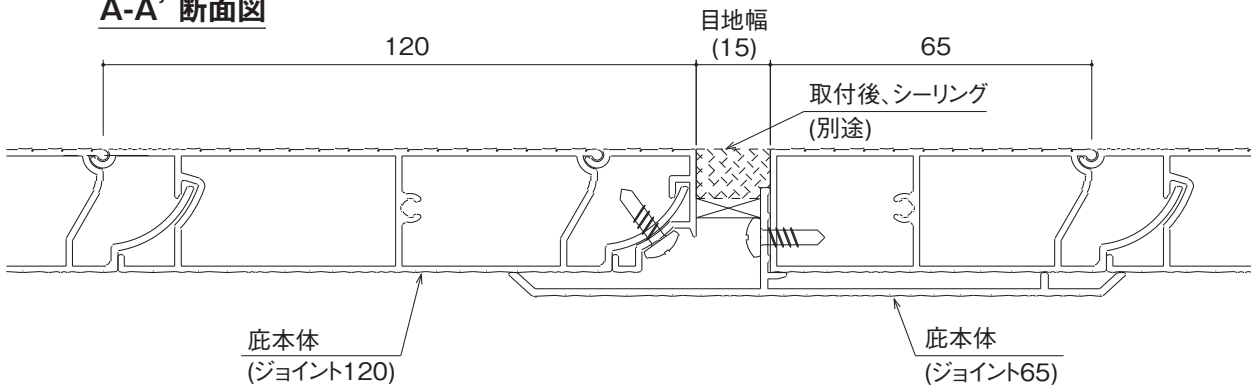
A-A' 断面図
