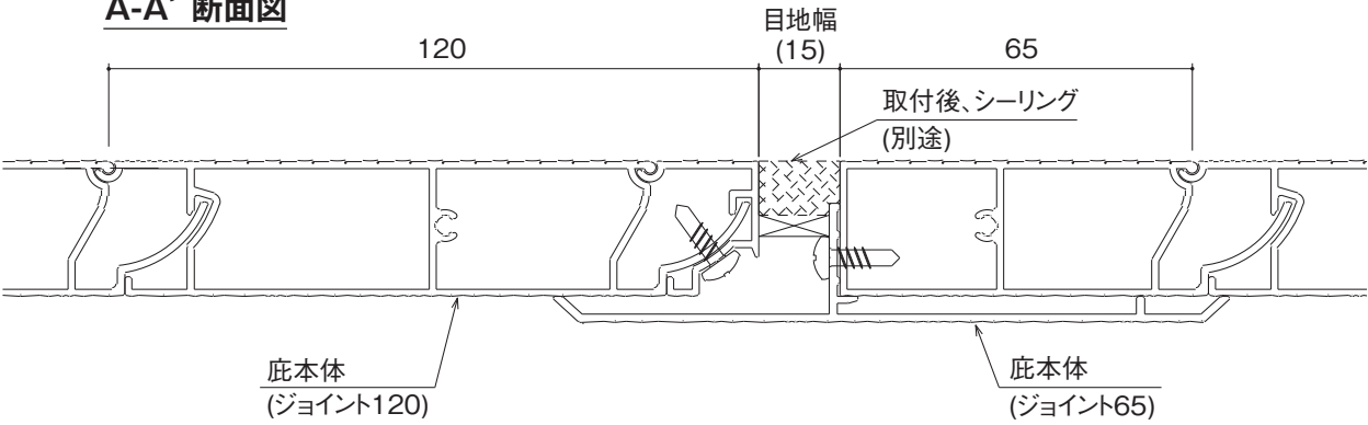
A-A' 断面図
